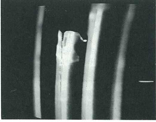
核三廠反應爐 控制棒底控 部分斷裂，用 水底攝影拍攝 R41的症狀， 控制棒斷裂、 腫脹，肉眼 可見。
