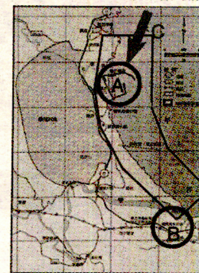
突堤效應: 因重件碼頭阻礙, 使東北季風冬天無法將沙源順利帶回福隆海域 A重件碼頭 B福隆海水域場 C東北季風
