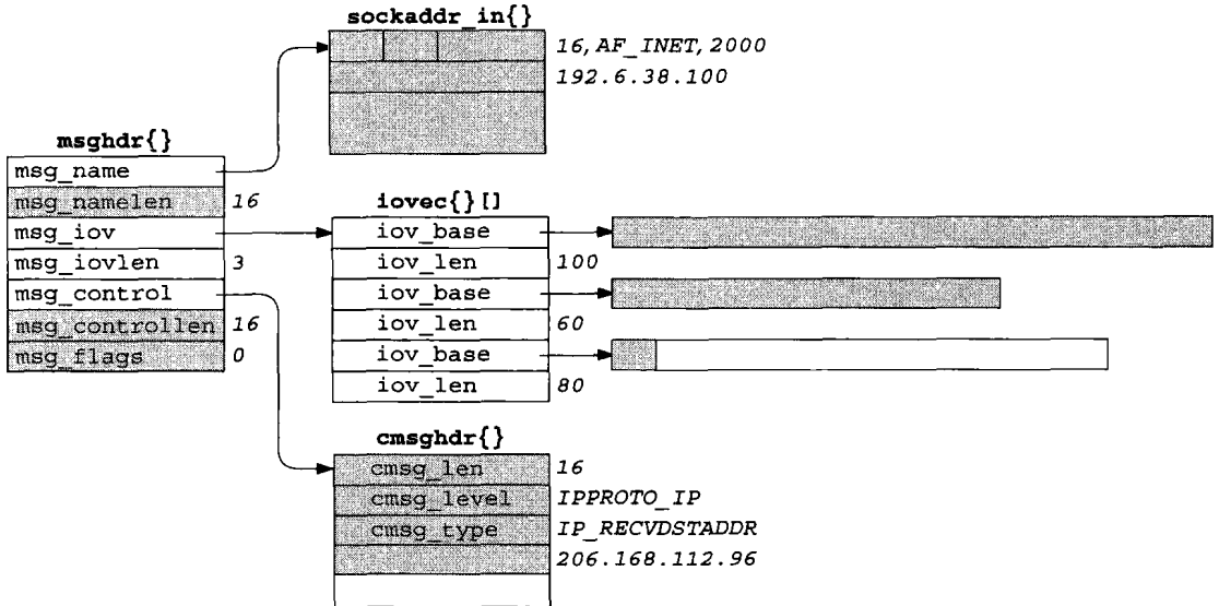
图14-9 recvmsg返回时对图14-8的更新
