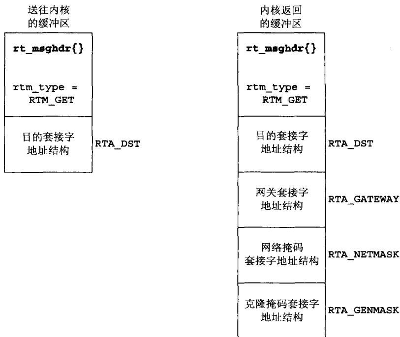
图18-5 RTM_GET命令通过路由套接字与内核交换的数据
