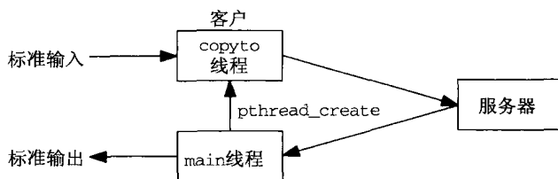
图26-1 使用线程重新编写str_cli
