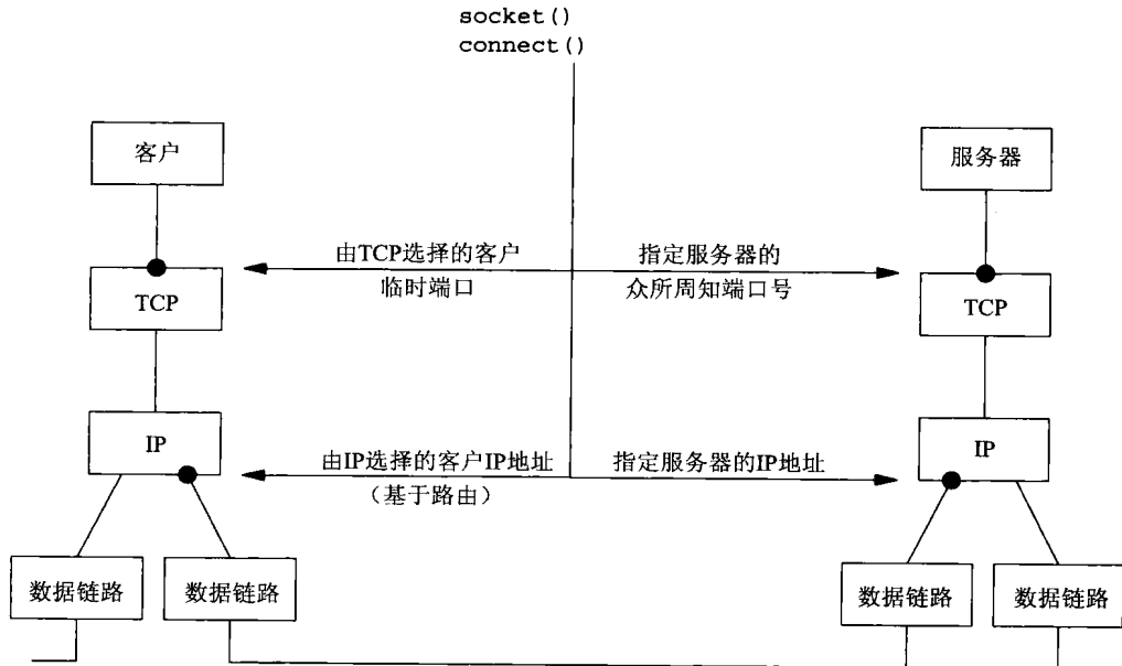
图5-15 从客户的角度总结TCP客户/服务器
