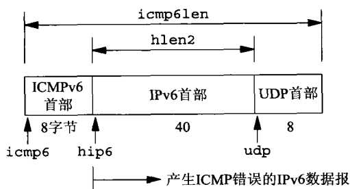
图28-22 处理ICMPv6错误涉及的首部、指针和长度
