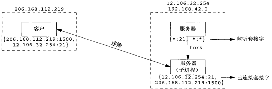
图2-13 并发服务器让子进程处理客户
