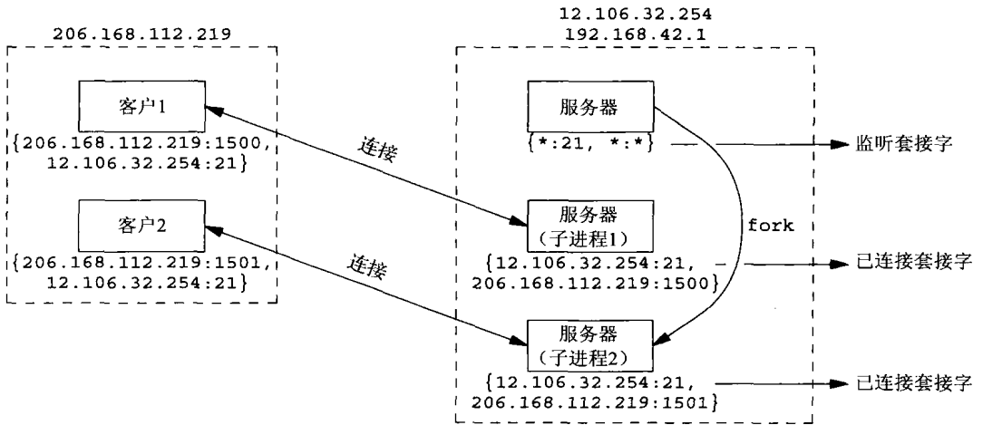
图2-14 第二个客户与同一个服务器的连接
