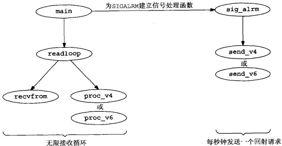
图28-3 我们的ping程序中各个函数的概貌
