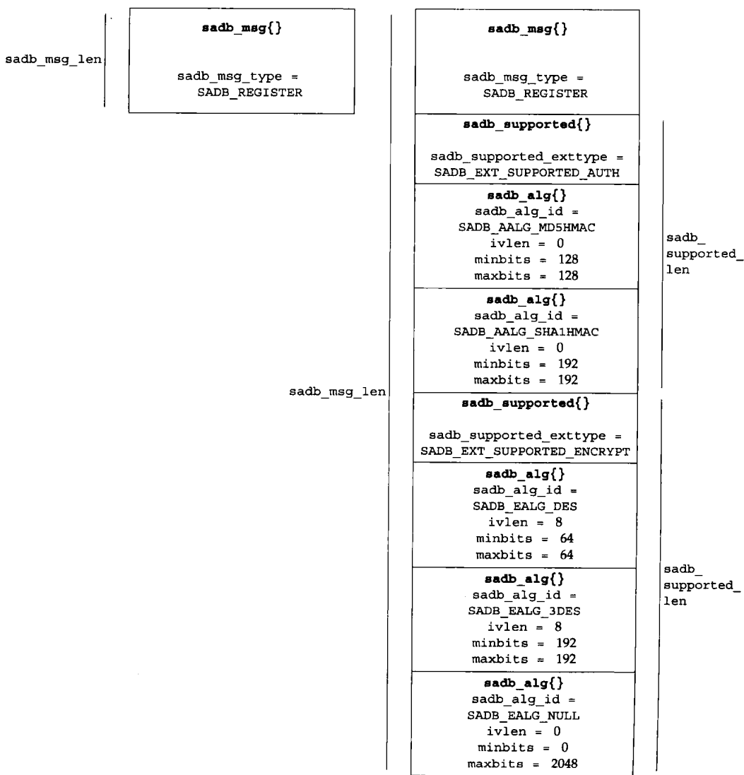
图19-14 内核为SADB_REGISTER请求返回的应答
