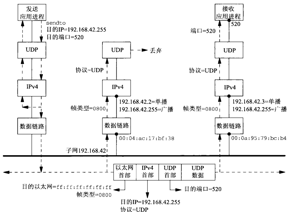
图20-4 UDP数据报广播示例
