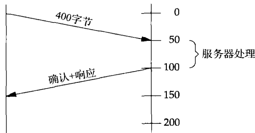
图E-8 使用writev代替设置TCP_NODELAY套接字选项
