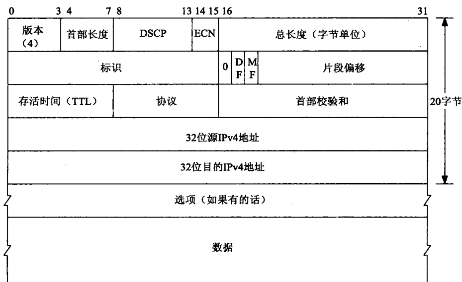
图A-1 IPv4首部格式
