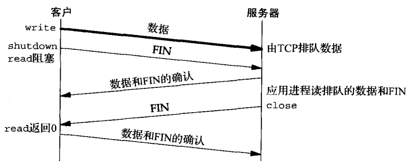
图7-10 用shutdown来获取对方已接收数据
