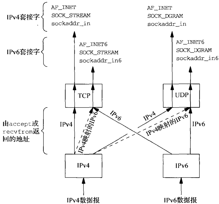
图12-3 根据接收套接字类型处理收到的IPv4数据报或IPv6数据报
