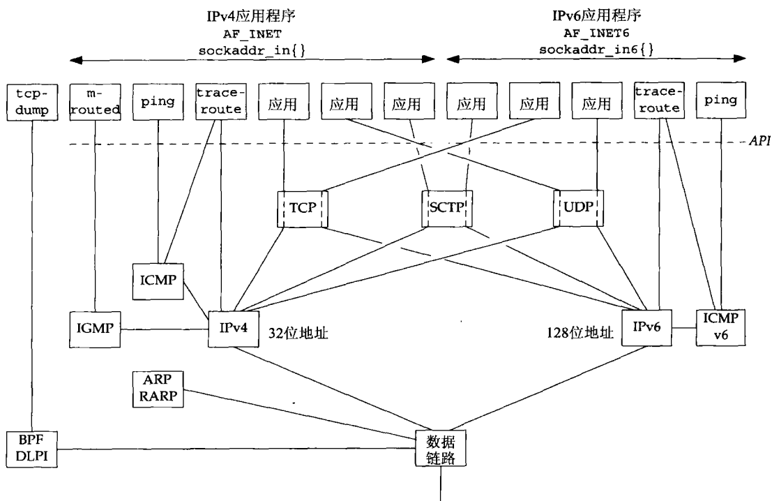
图2-1 TCP/IP协议概况
