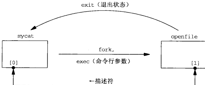
图15-8 启动执行 openfile 程序后的 mycat 进程
