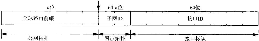
图A-8 IPv6全球单播地址一般格式
