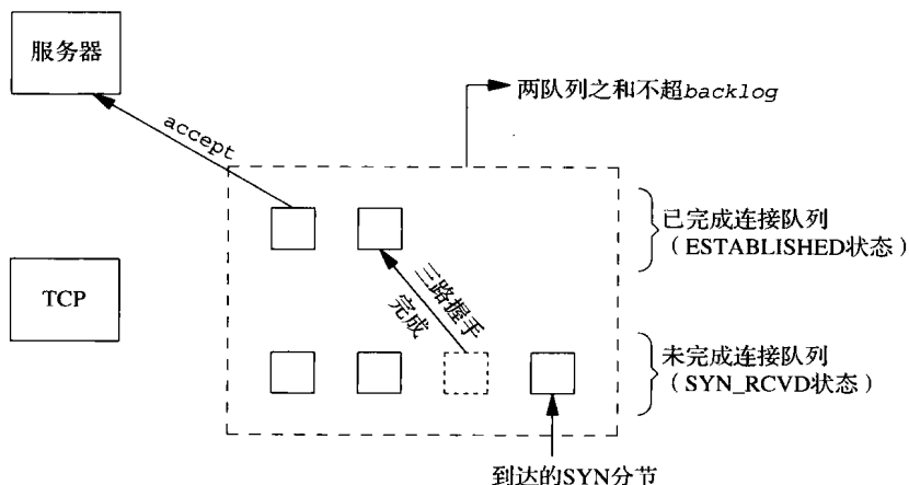
图4-7 TCP为监听套接字维护的两个队列
