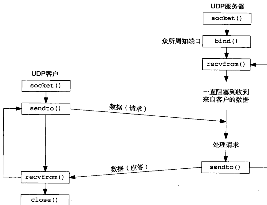
图8-1 UDP客户/服务器程序所用的套接字函数
