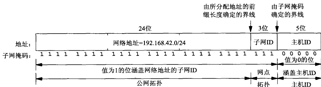
图A-4 24位网络ID伴以3位子网ID和5位主机ID
