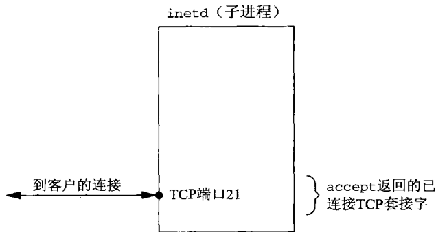
图13-9 子进程中的inetd描述符
