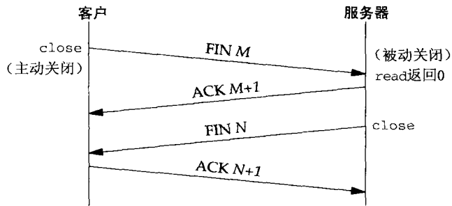
图2-3 TCP连接关闭时的分组交换
