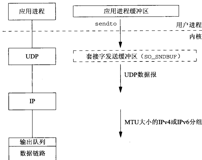
图2-16 应用进程写UDP套接字时涉及的步骤与缓冲区
