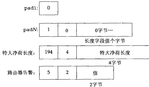
图27-9 IPv6步跳选项
