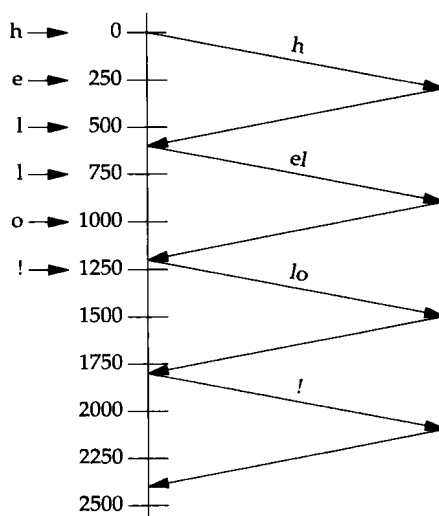
图7-14 禁止Nagle算法时由服务器回显的六个字符 图7-15 开启Nagle算法时由服务器回显的六个字符
