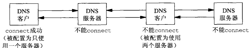
图8-16 DNS客户、服务器与connect函数的例子
