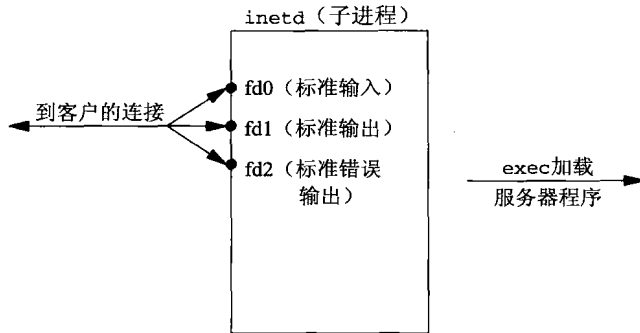
图13-10 dup2后子进程中的inetd描述符
