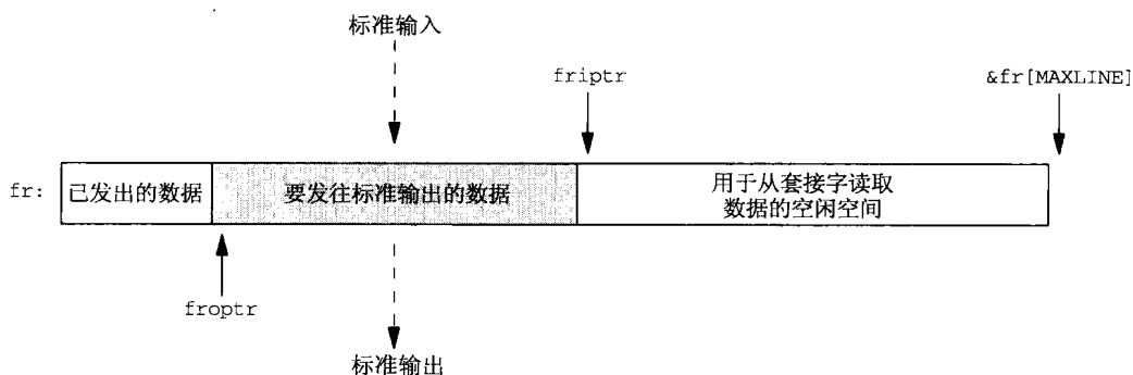
图16-2 容纳从套接字到标准输出的数据的缓冲区
