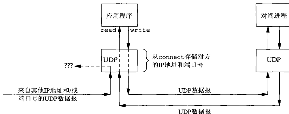
图8-15 已连接UDP套接字
