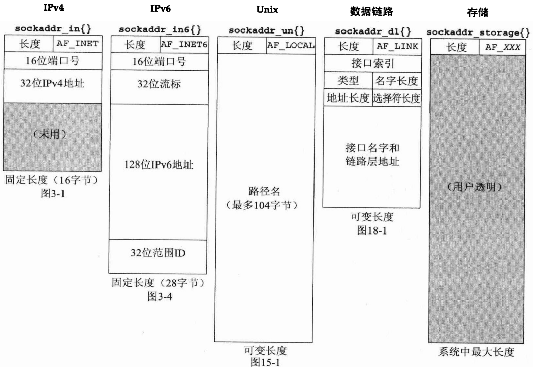
图3-6 不同套接字地址结构的比较
