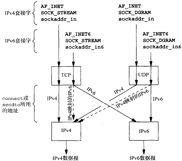
图12-4 根据地址类型和套接字类型处理客户请求
