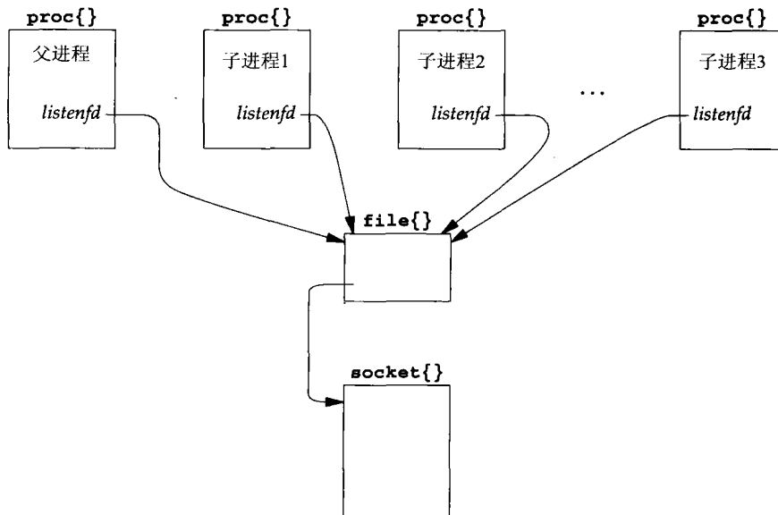
图30-13 proc、file和socket这三个结构之间的关系
