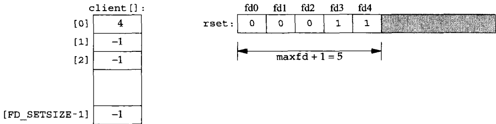
图6-17 第一个客户连接建立后的数据结构
