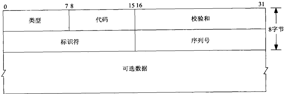
图28-1 ICMPv4和ICMPv6回射请求和回射应答消息的格式
