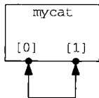
图15-7 使用 socketpair 创建流管道后的 mycat 进程
