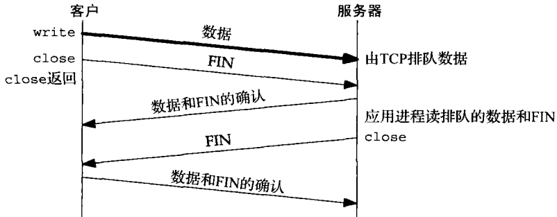
图7-7 close的默认操作：立即返回
