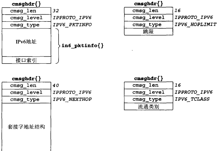
图22-21 IPv6分组信息的辅助数据
