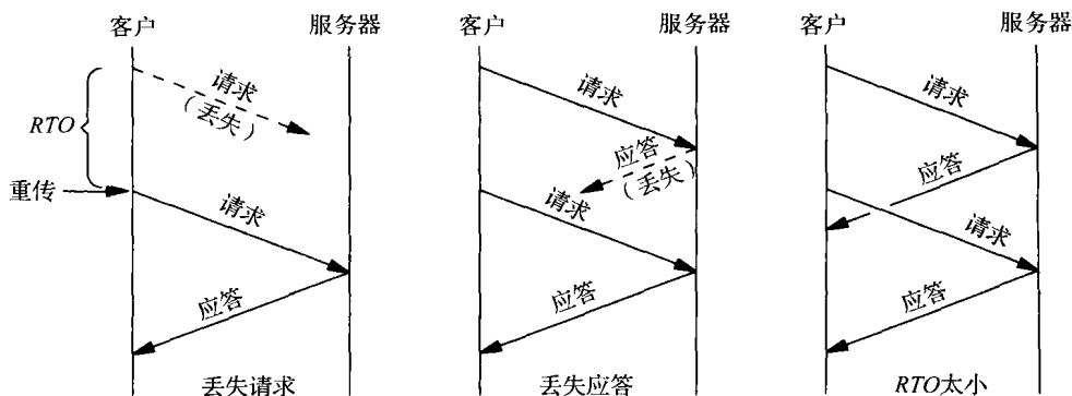
图22-5 重传定时器期满时的3种情形
