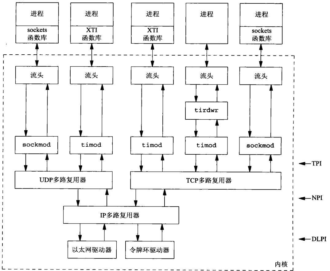
图31-3 TCP/IP基于流的某种可能的实现
