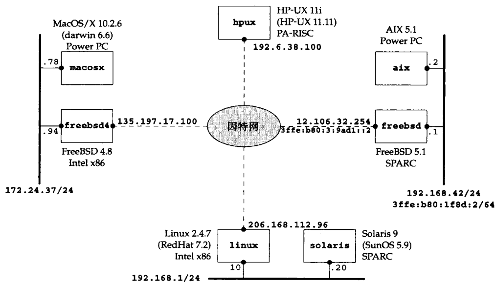
用于正文中大多数示例的主机和网络
