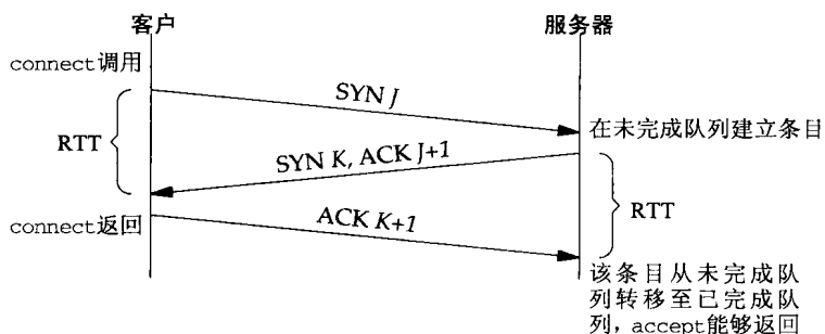
图4-8 TCP三路握手和监听套接字的两个队列
