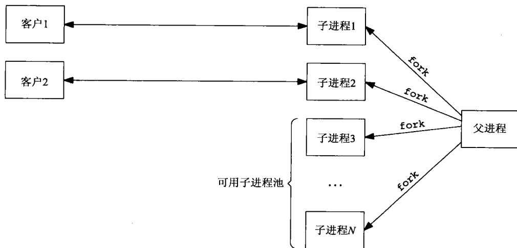
图30-8 服务器预先派生子进程
