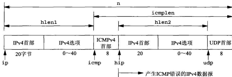
图28-21 处理ICMPv4错误涉及的首部、指针和长度
