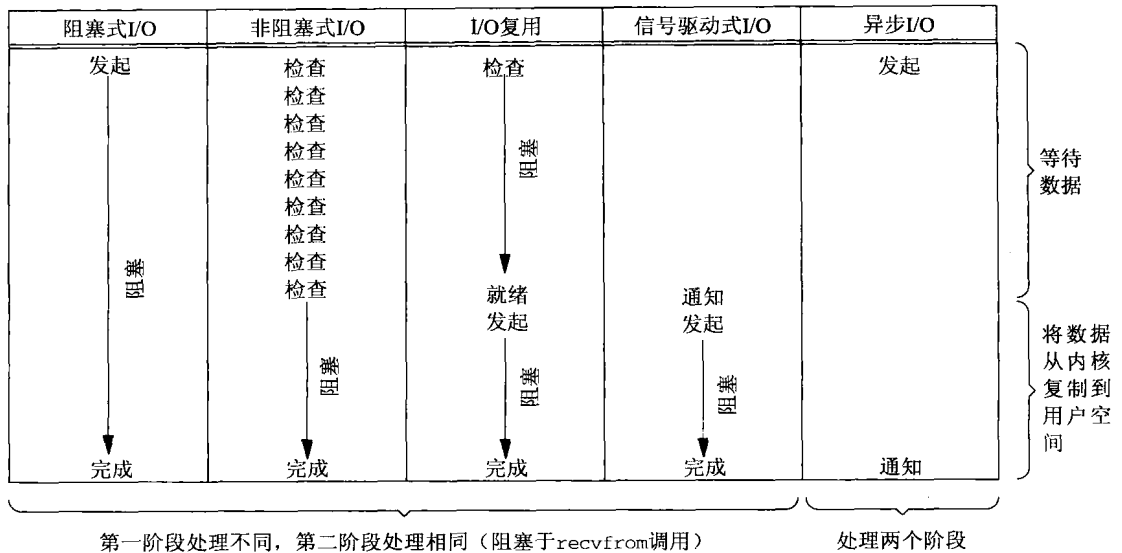
图6-6 5种I/O模型的比较
