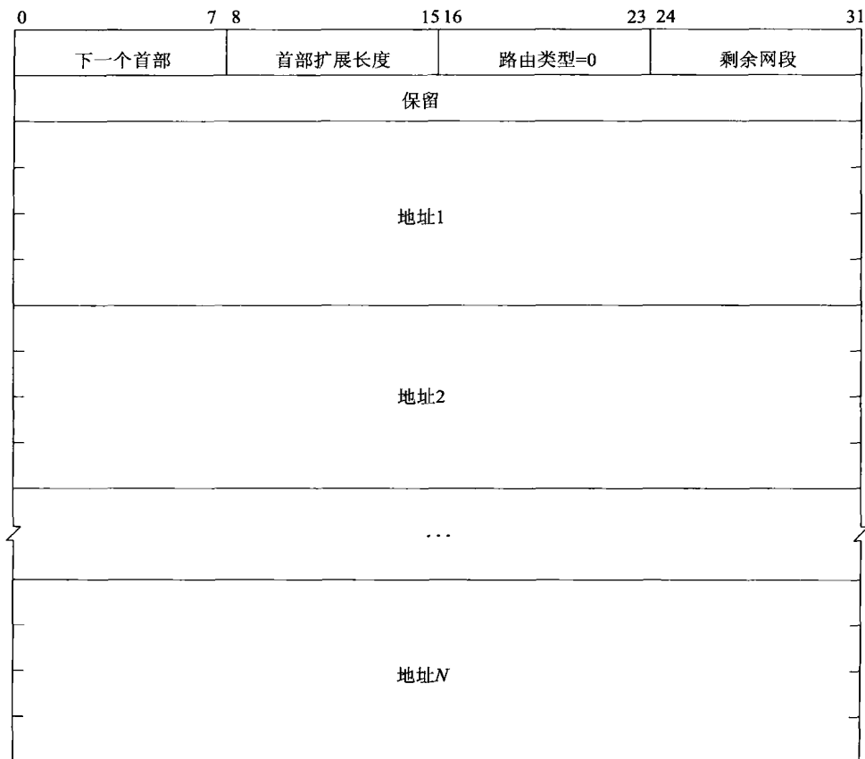
图27-11 IPv6路由首部
