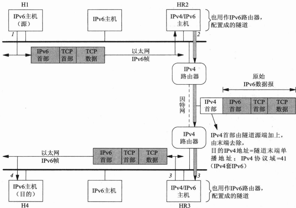
图B-2 6bone上使用的IPv4套IPv6封装
