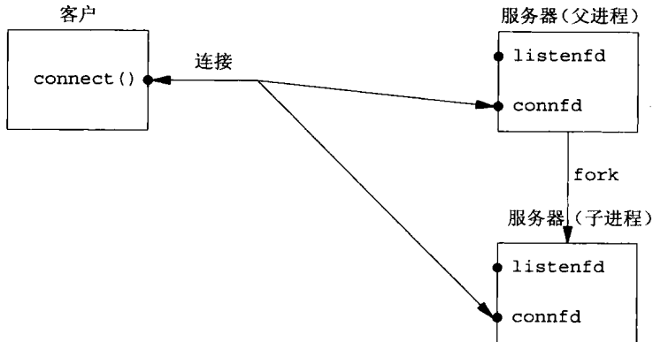
图4-16 fork返回后客户/服务器的状态
