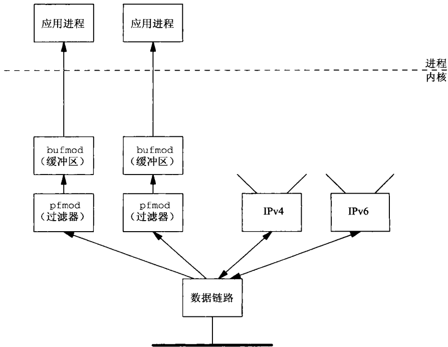
图29-2 使用DLPI、pfmod和bufmod捕获分组
