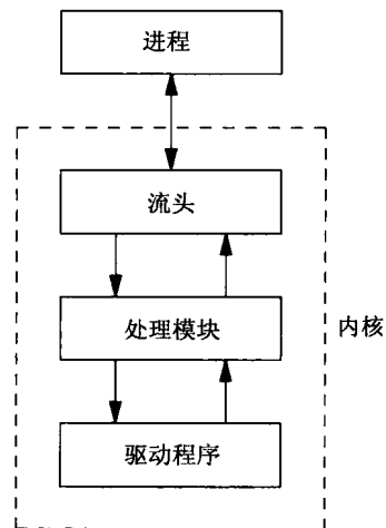
图31-2 压入一个处理模块的某个流
