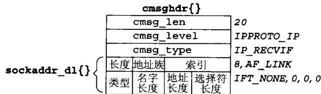
图22-3 IP_RECVIF返回的辅助数据对象
