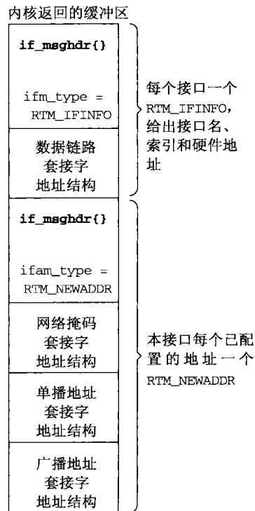
图18-13 由sysctl的CTL_NET/AF_ROUTE/NET_RT_IFLIST命令返回的信息
