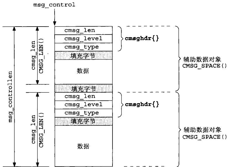
图14-12 包含两个辅助数据对象的辅助数据
