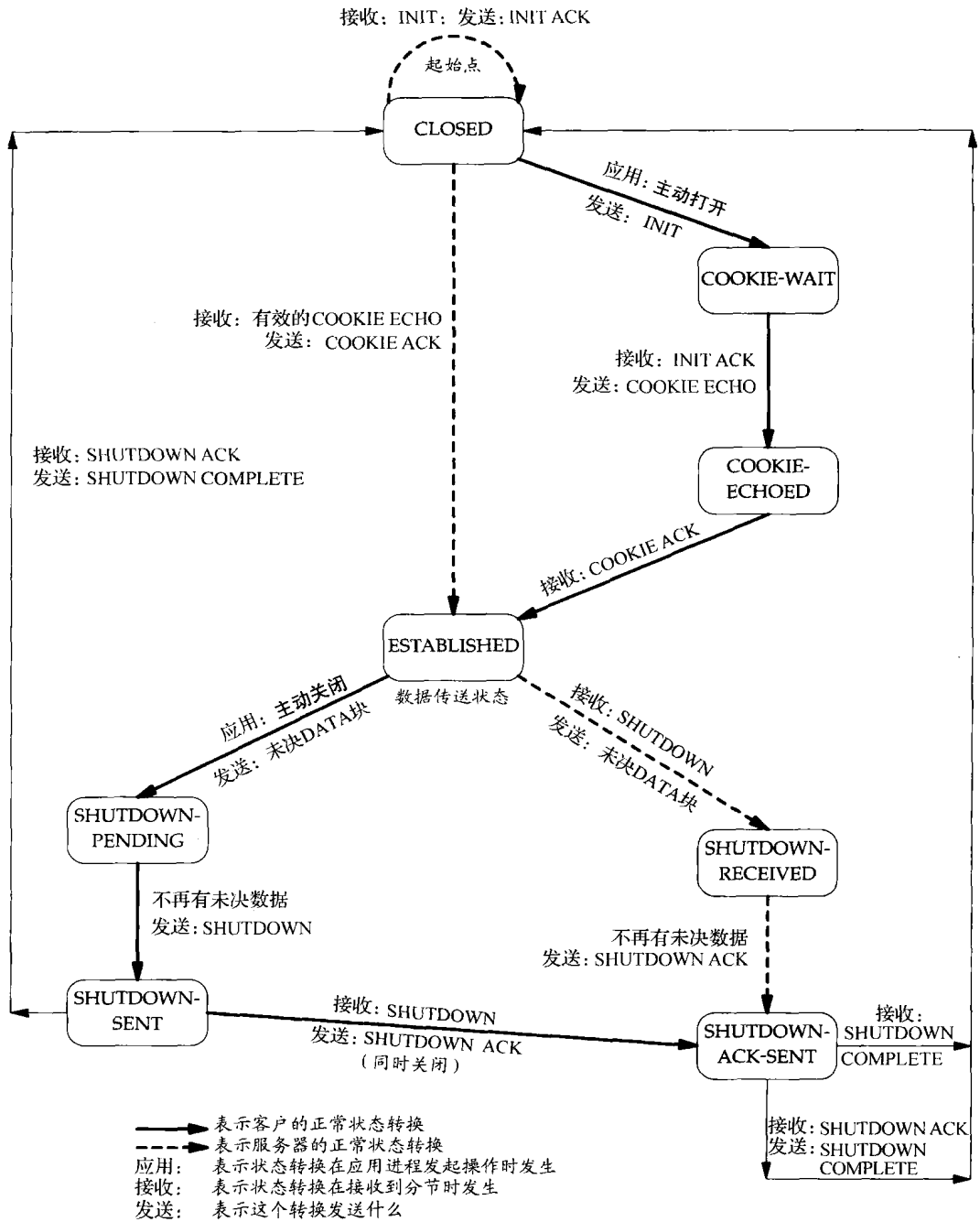
图2-8 SCTP状态转换图
