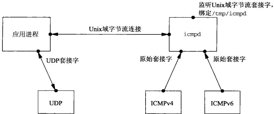
图 28-27 应用进程创建自身的 UDP 套接字和到 icmpd 的 Unix 域连接
