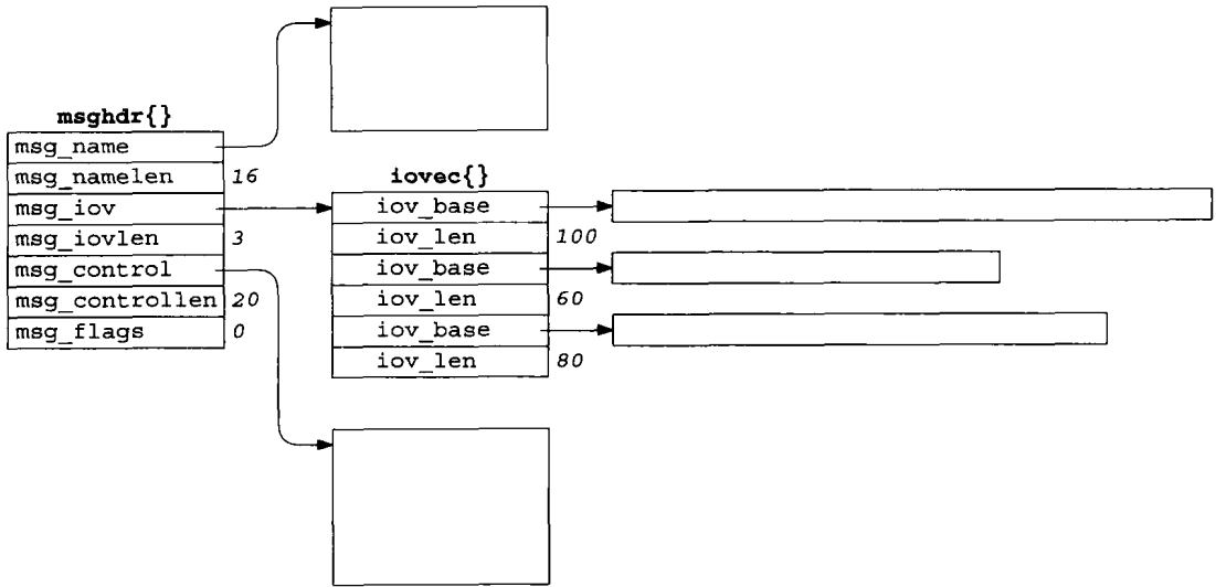
图14-8 对一个UDP套接字调用recvmsg时的数据结构
