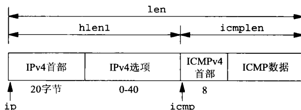
图28-9 处理ICMPv4应答涉及的首部、指针和长度
