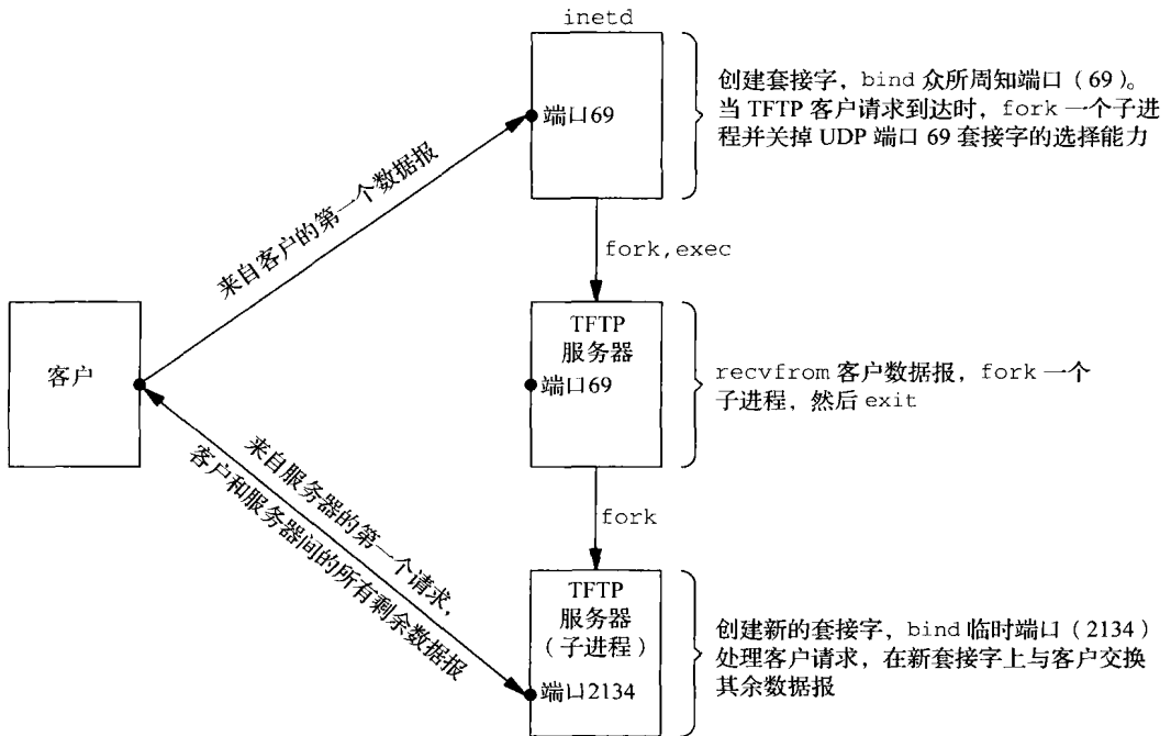
图22-20 由inetd激发的UDP并发服务器所涉及步骤
