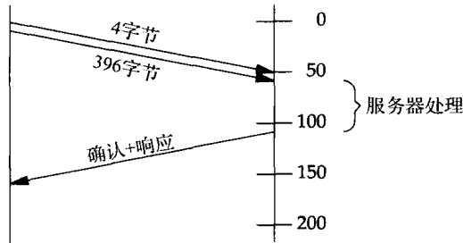
图E-7 通过设置TCP_NODELAY套接字选项避免Nagle算法
