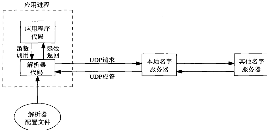
图11-1 客户、解析器和名字服务器的典型关系
