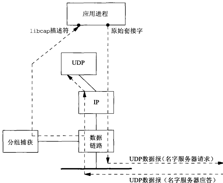
图29-3 检查某个名字服务器是否开启UDP校验和的应用程序
