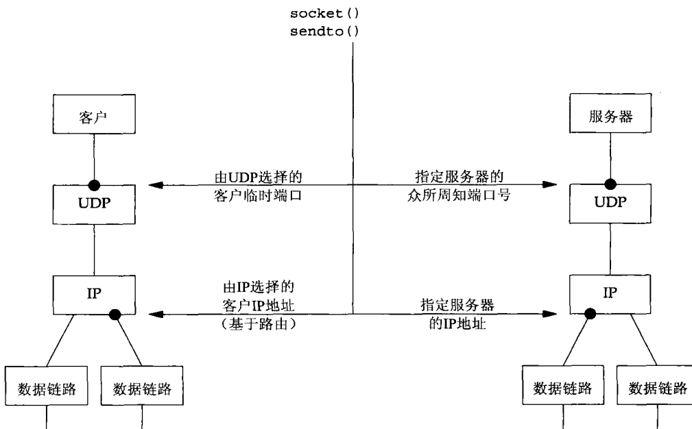
图8-11 从客户角度总结UDP客户/服务器
