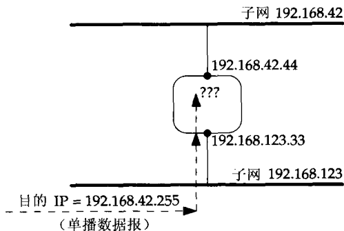
图20-2 路由器转发子网定向广播分组吗?
