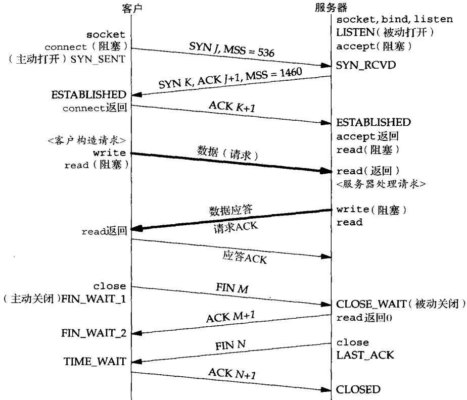
图2-5 TCP连接的分组交换
