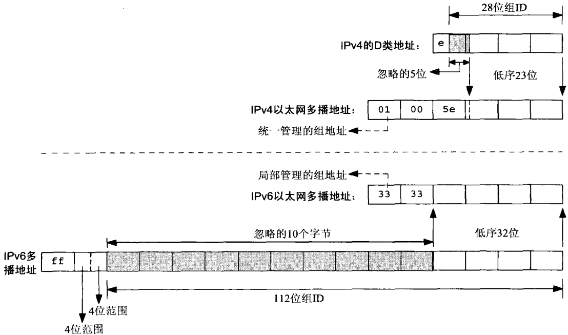
图21-1 IPv4和IPv6多播地址到以太网地址的映射
