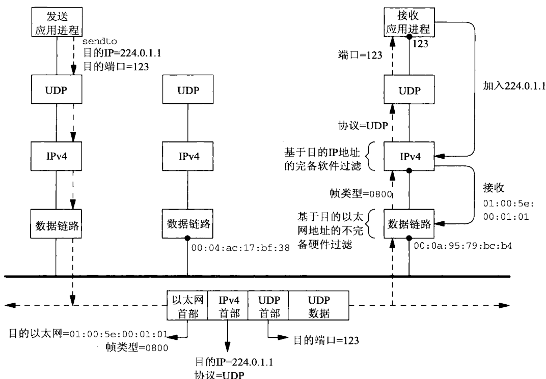
图21-4 UDP数据报多播示例
