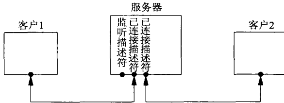
图6-18 第二个客户建立连接后的TCP服务器
