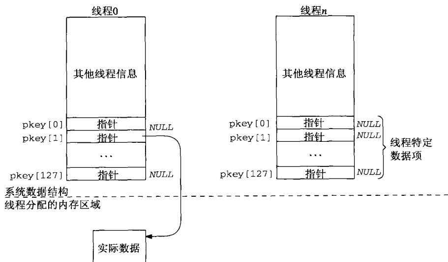
图26-9 把malloc到的内存区和线程特定数据指针相关联
