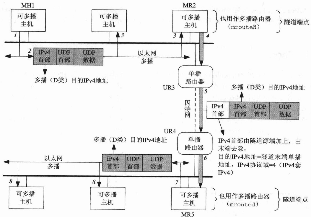
图B-1 MBone上使用的IPv4套IPv4封装
