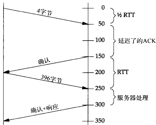
图E-6 Nagle算法与延滞ACK的交互情况
