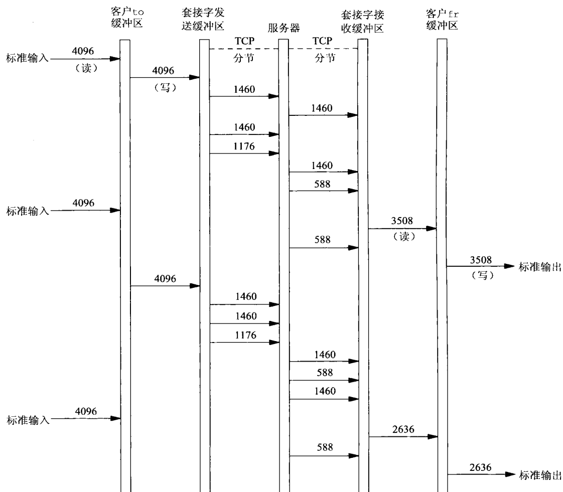
图16-8 非阻塞式I/O例子的时间线
