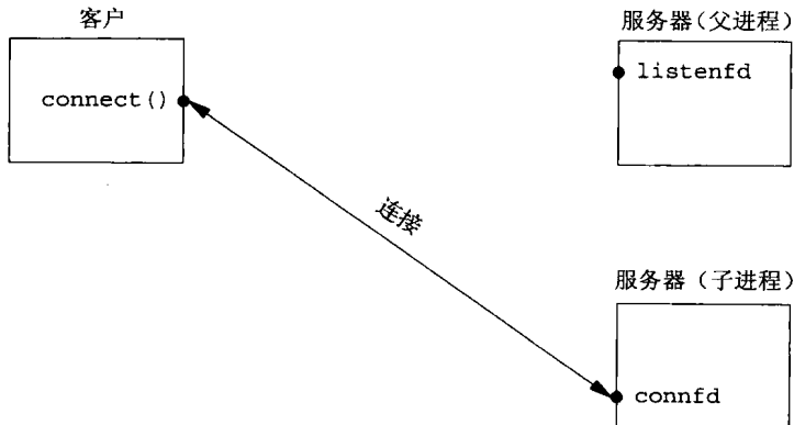
图4-17 父子进程关闭相应套接字后客户/服务器的状态
