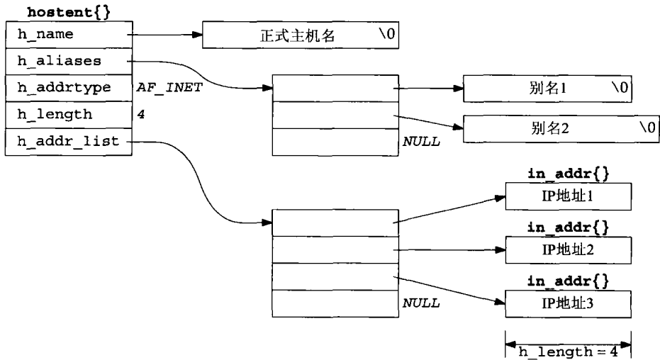
图11-2 hostent结构和它所包含的信息
