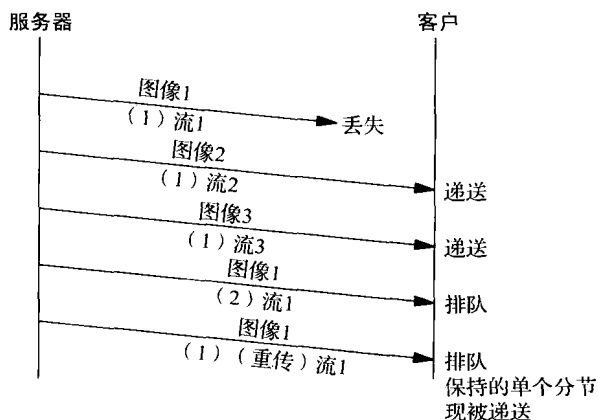
图10-6 在3个SCTP流上发送3幅图像
