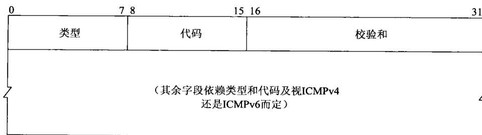
图A-14 ICMPv4和ICMPv6消息的格式
