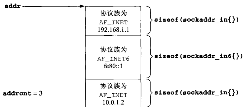
图9-4 SCTP调用所需的紧凑地址列表格式
