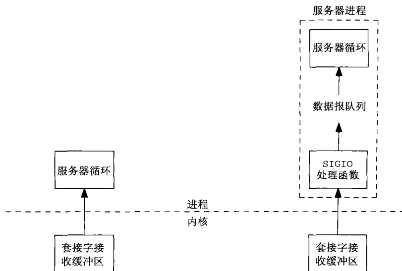
图25-1 构建一个UDP服务器的两种方式
