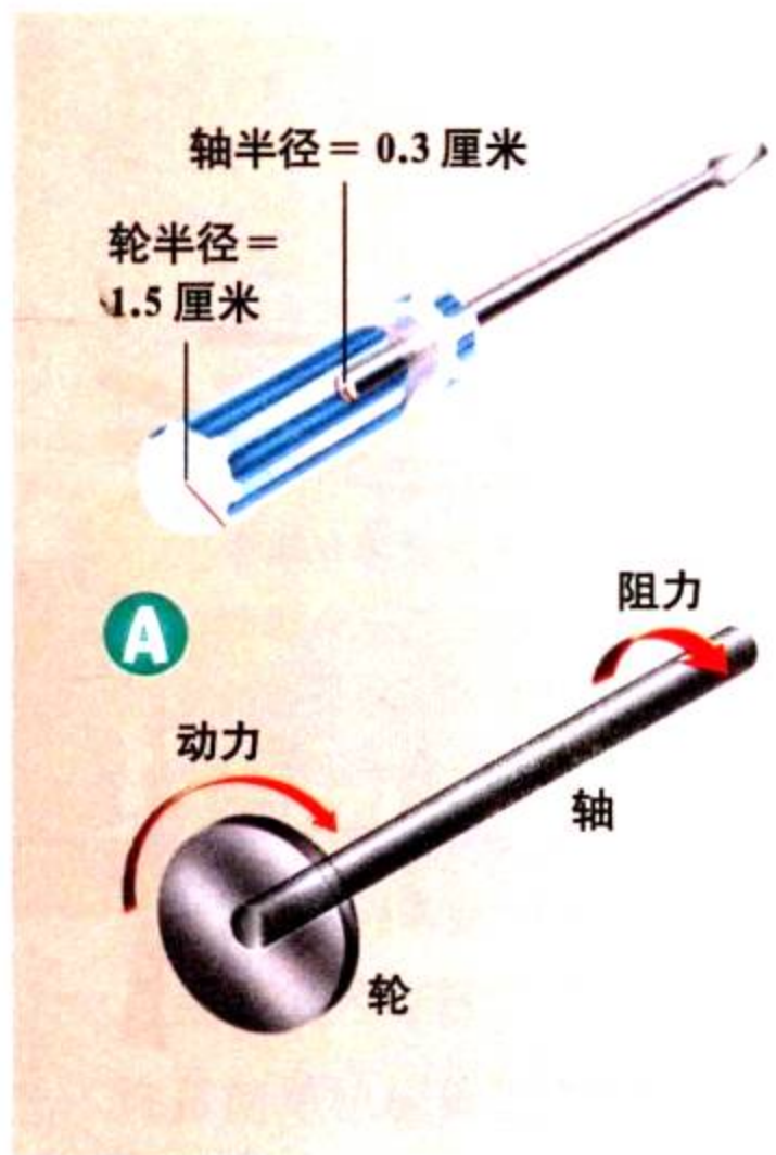
图 4-17 图 A 所示的螺丝刀，是轮转动轴。然而，如图 B 所示，游船的明轮却是轴转动轮。
