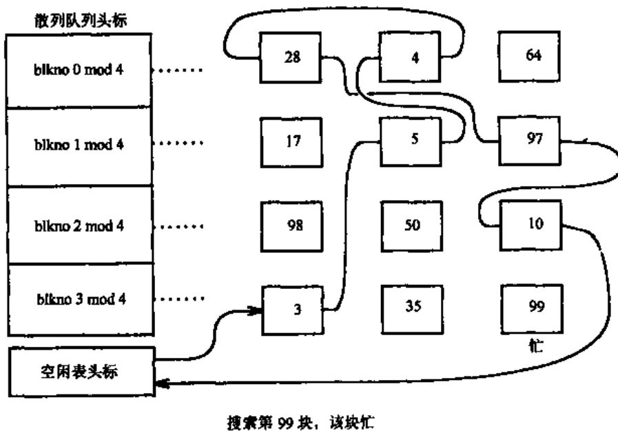
图 3-11 缓冲分配的第五种情况
