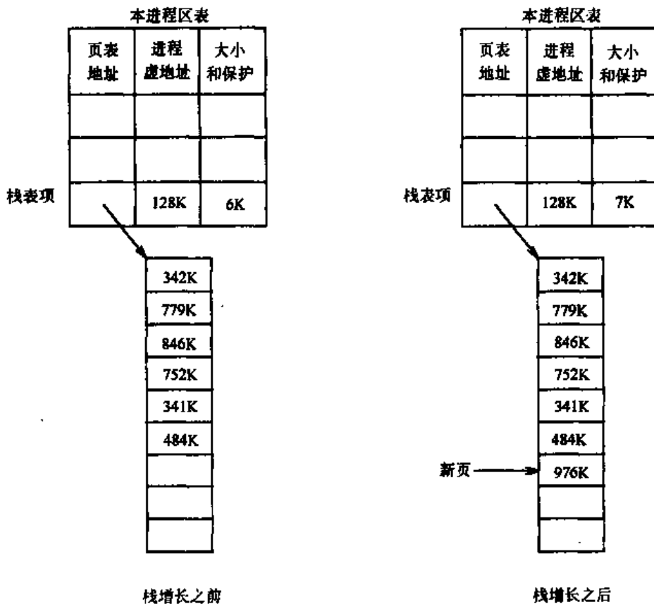
图 6-22 栈区增长 1K 字节
