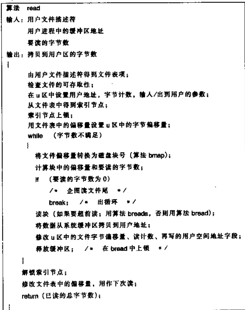
图 5-5 读文件的算法
