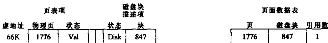
图 9-23 页面被换入内存之后
