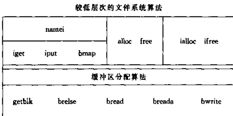
图 4-1 文件系统算法
