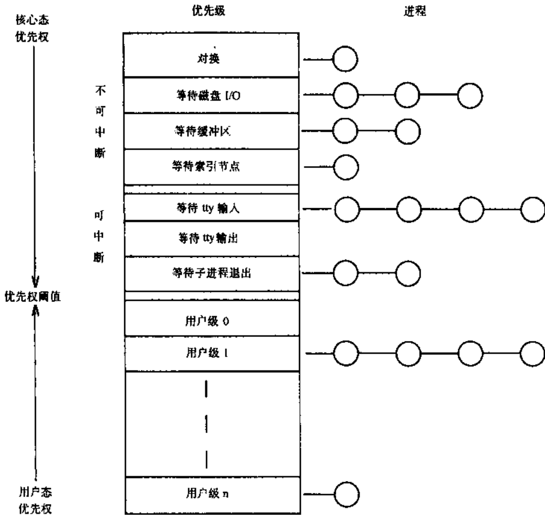
图 8-2 进程优先权的范围
