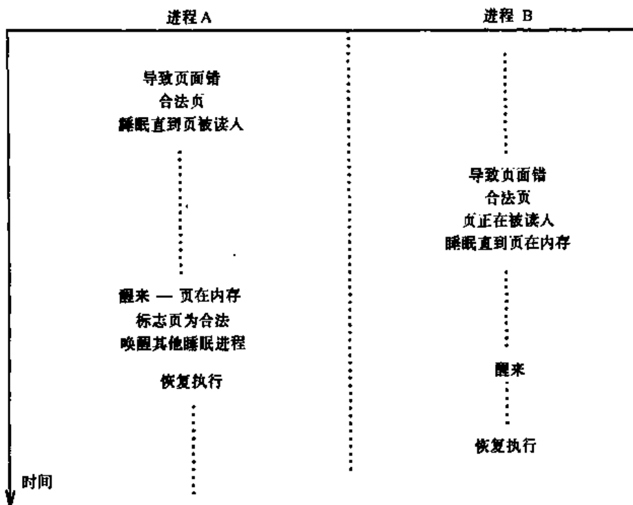
图 9-24 同一页面上的二重错
