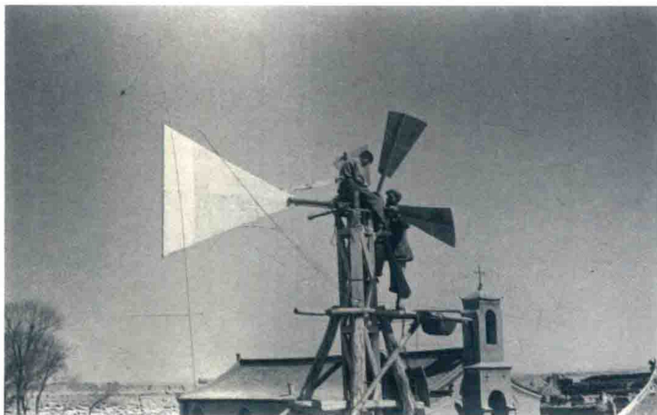
◎1949年，阳早与刘德英在三边牧场安装寒春设计的风车
