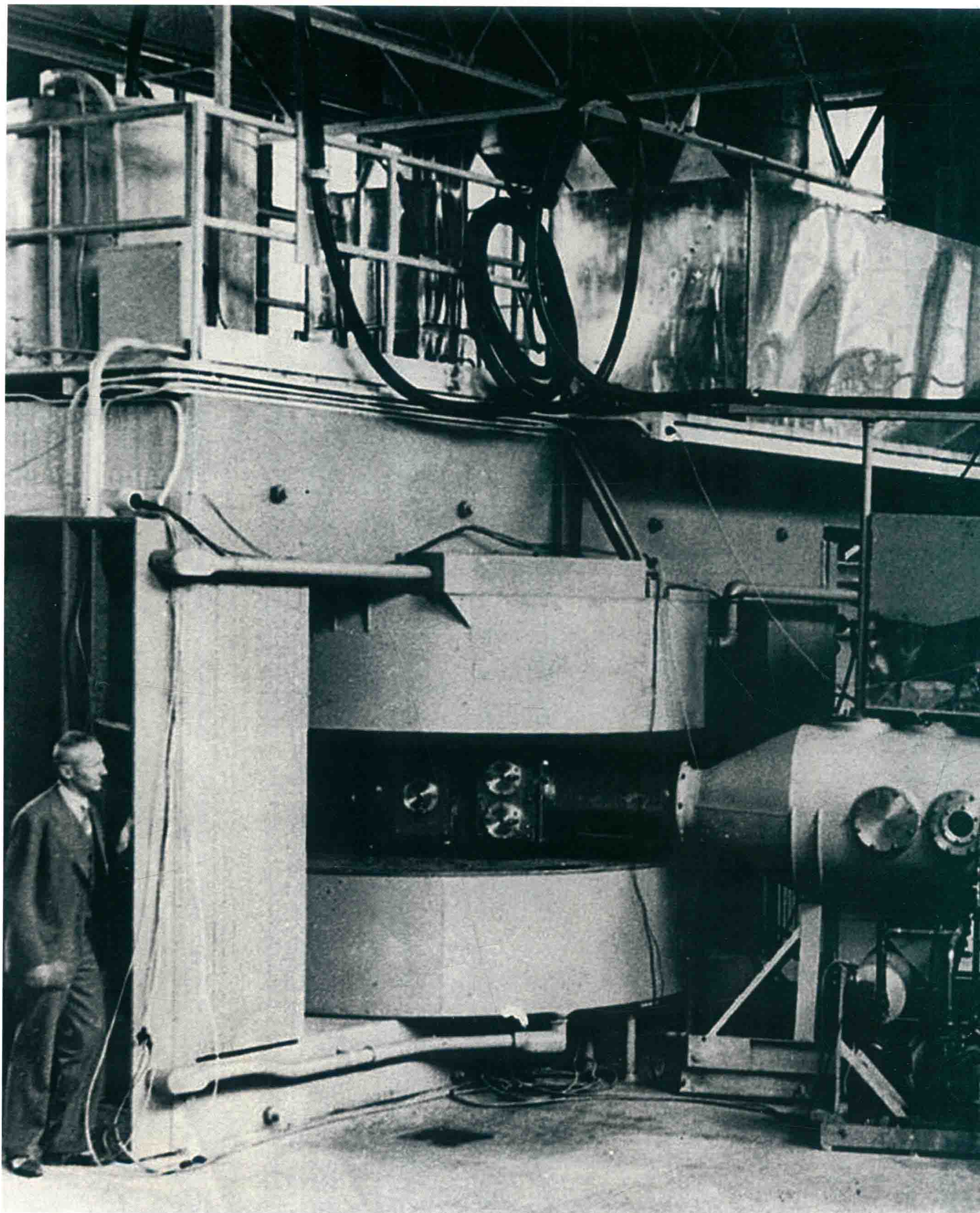
©1939年的加速器（图片来源：网络）
