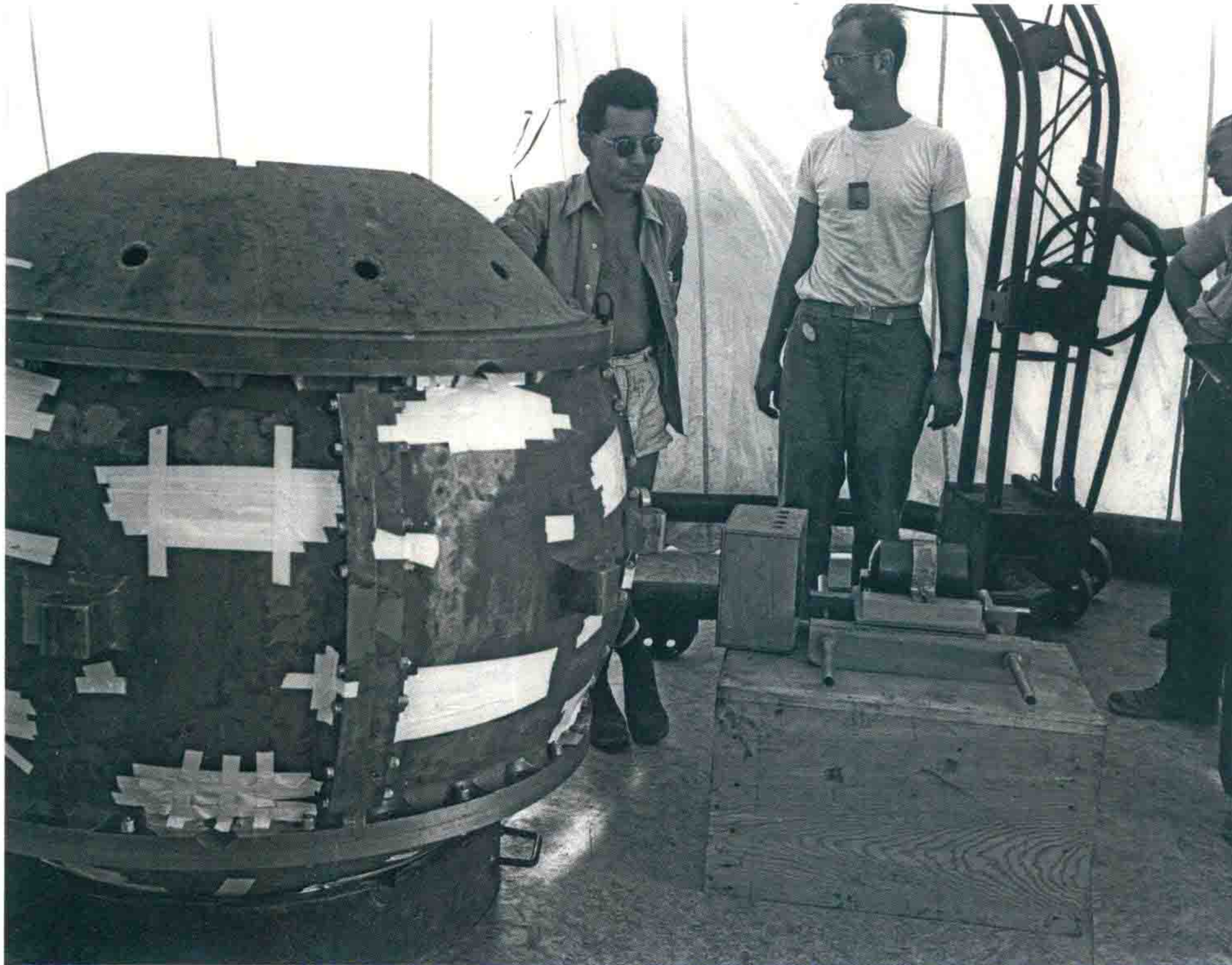
◎中间穿T恤的哈里·达里安是原子辐射的第一个受害者（图片来源：网络）
