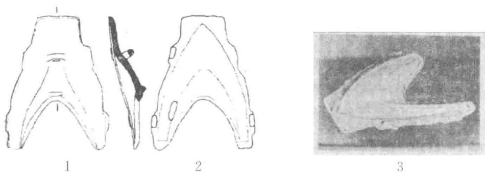
图三十 金代出土的铜犁范
