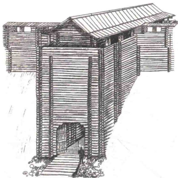
图 2-8 11~13 世纪姆斯克城堡内城大门复原图
