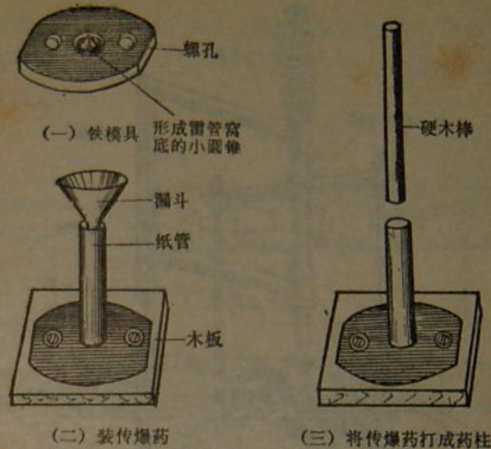
第15图 装传爆药
