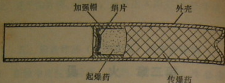
第12图 雷管
