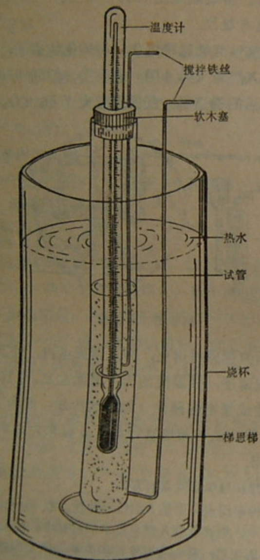
第7图 测量凝固点装置
