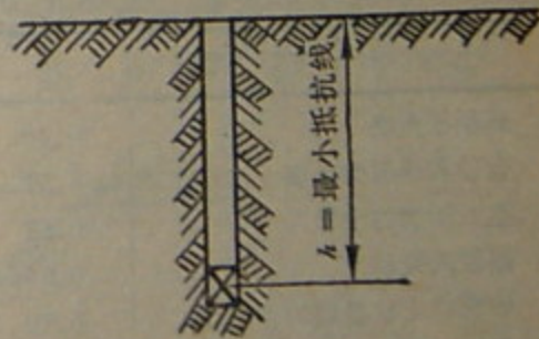
第64图 最小抵抗线等于装药入土深度
