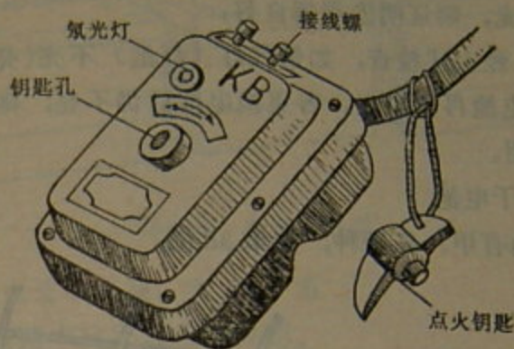
第37图 MFD-25型发爆器
