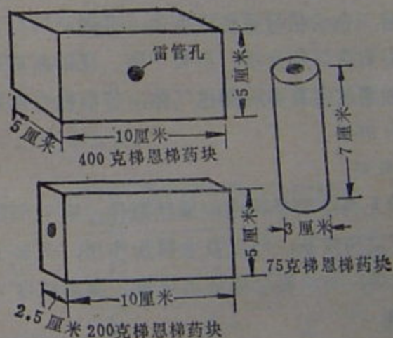
第2图 梯恩梯药块
