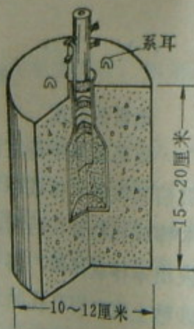
第87图 混凝土雷
