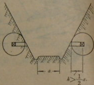
第45图 爆破两侧侧坡装药的配置
