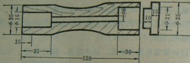
附12图 弹柄与木质弹盖
