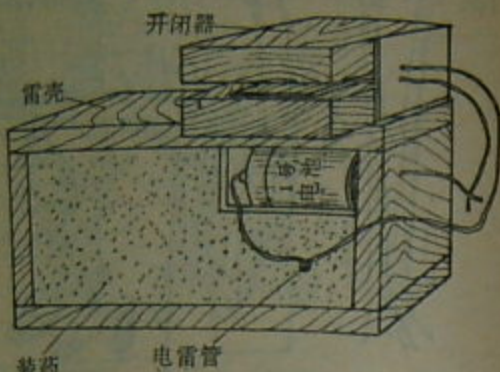
第120图 木壳防坦克地雷
