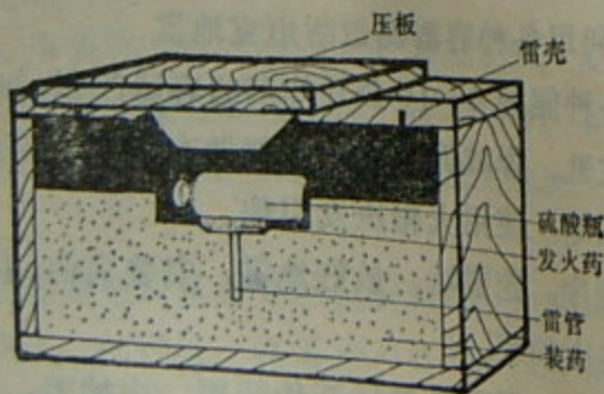
第124图 化学发火的防坦克地雷
