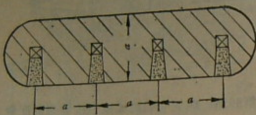
第62图 装药设置在桥墩厚度1/2深药洞中
