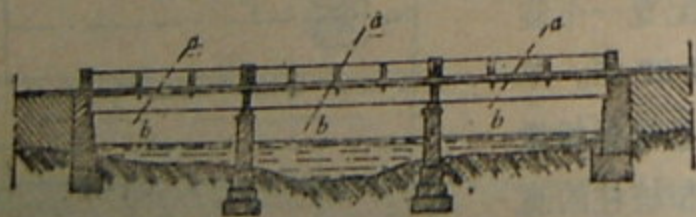
第53图 爆破上部结构时的破坏位置
