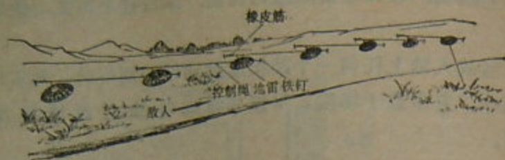
第111图 橡皮筋连环雷群
