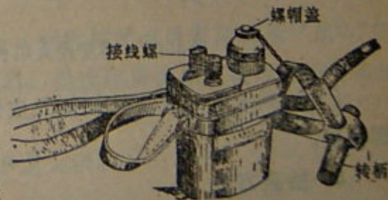
第35图 25发打火机
