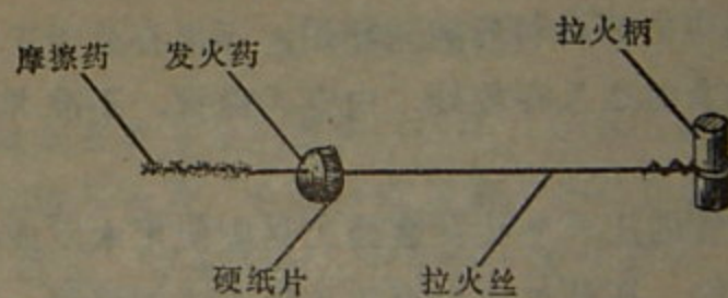
第27图 拉火管的拉火具
