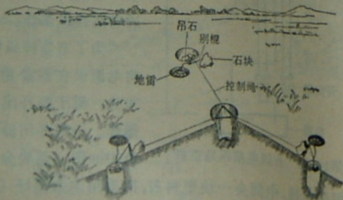
第109图 三连环雷群
