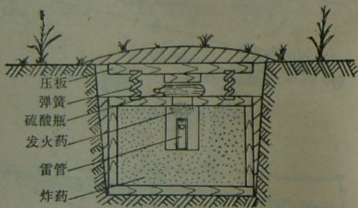
第103图 化学发火雷
