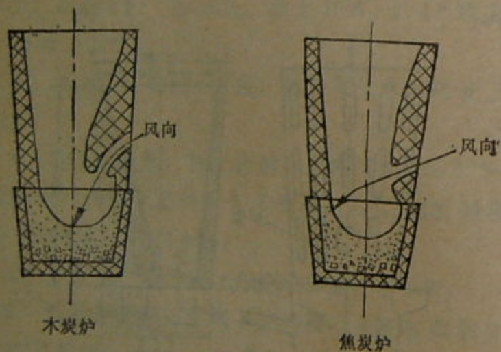
附 9 图 风口方位示意图
