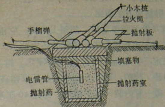
第128图 土坑抛射手榴弹
