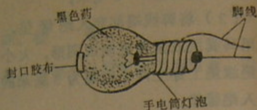
第21图 用小灯泡改装的电点火具
