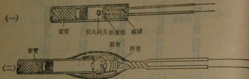
第22图 电雷管的装配
