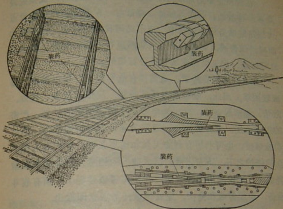
第47图 铁道的爆破
