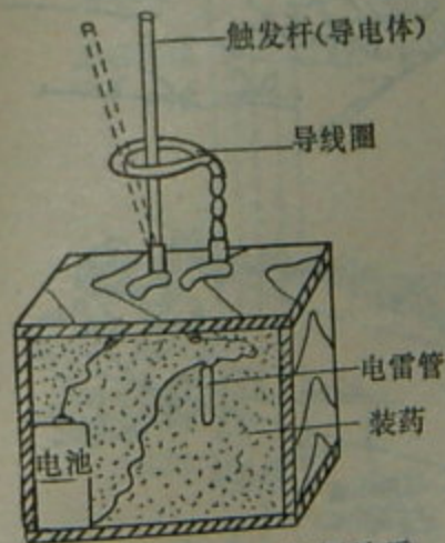
第105图 防探地雷
