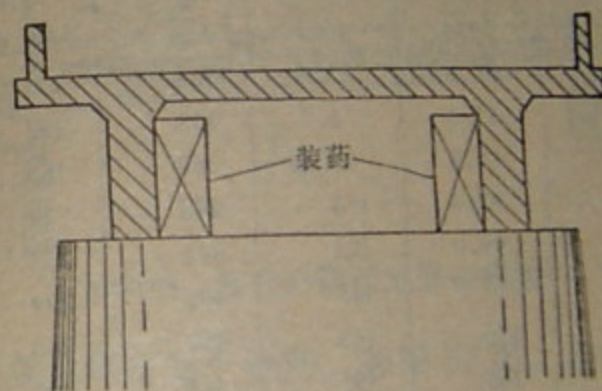
第55图 装药配置在桥墩上
