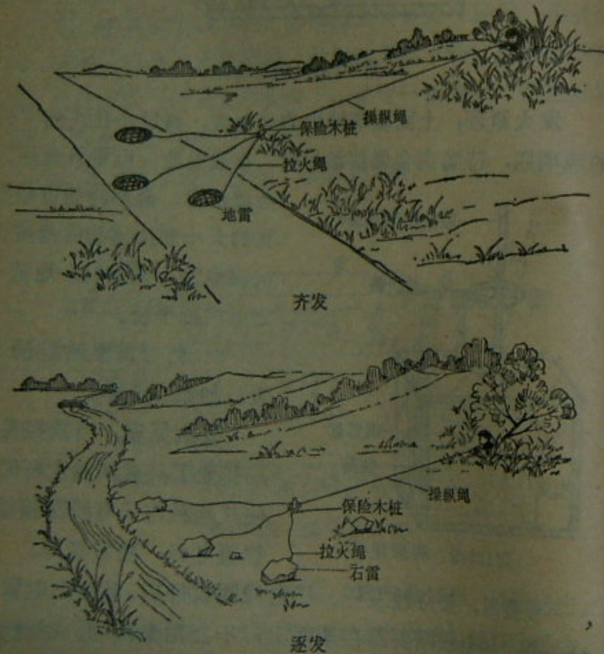
第106图 拉发地雷群
