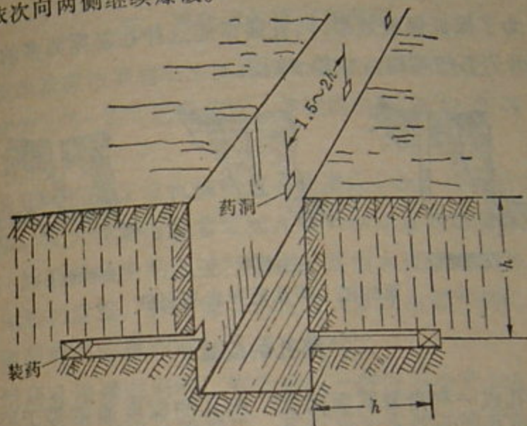
第68图 开设小沟松散冻土装药的配置
