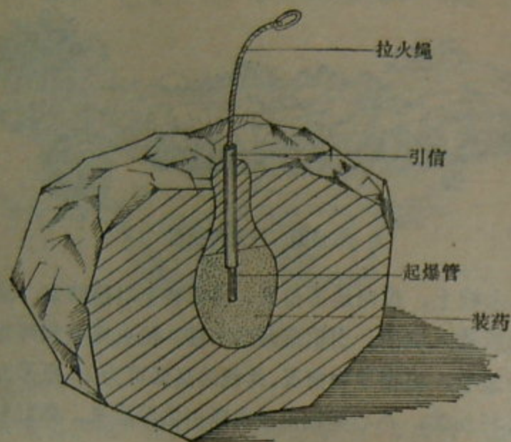
第84图 石雷
