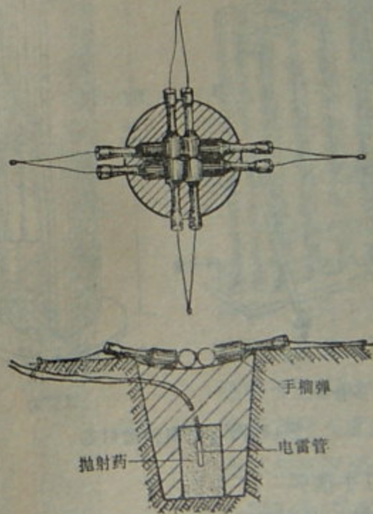
第129图 没有抛射板的抛射手榴弹
