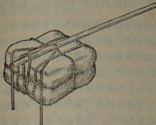
第75图 放于履带上的装药
