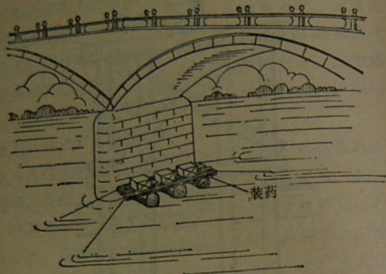
第49图 用筏配置固定装药
