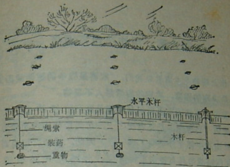
第71图 冰下装药的设置
