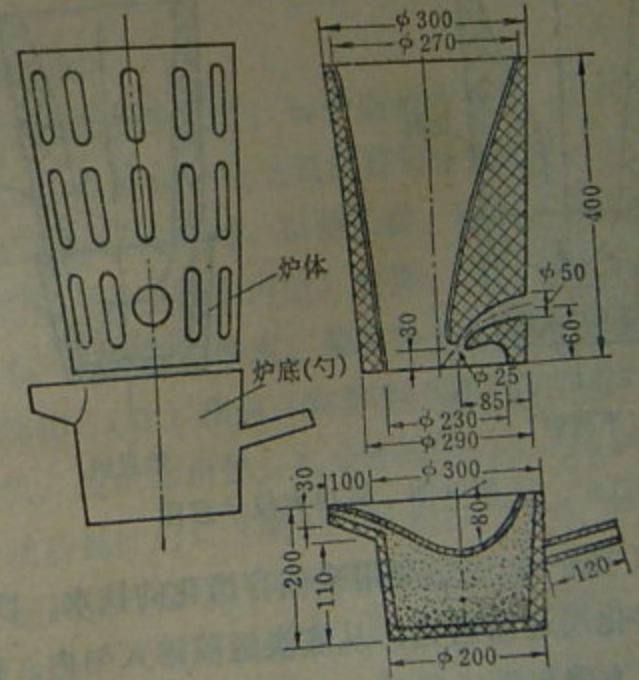
附8图 化铁炉的结构
