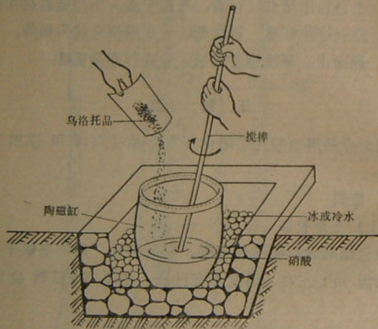
第 8 图 乌洛托品的硝化
