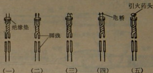
第20图 电点火具的制作
