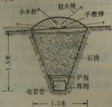
第127图 对空掷石雷
