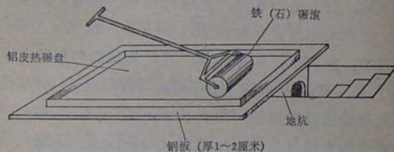
第1图 热碾设备
