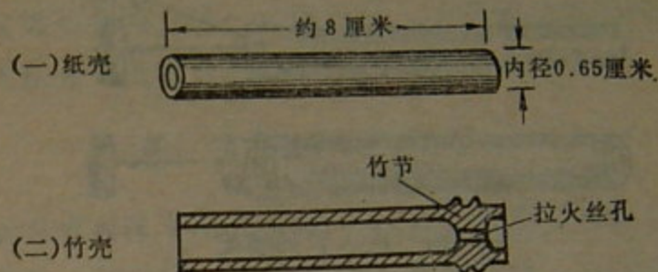
第26图 拉火管的外壳
