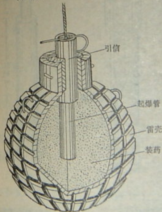
第79图 铸铁雷
