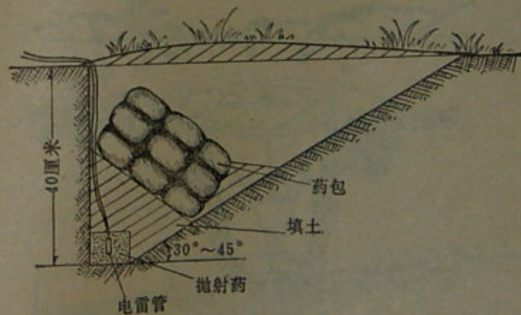
第96图 抛射单个药包
