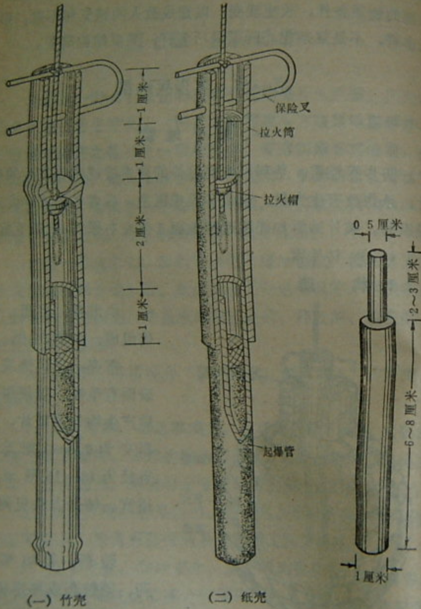
第80图 火帽拉发引信
