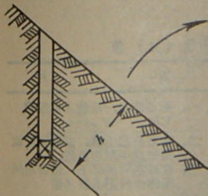
第63图 土、石的主要飞散方向
