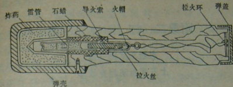
附14图 有雷管装硝铵炸药手榴弹
