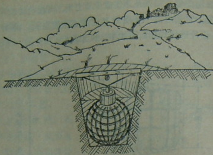
第97图 踏转雷
