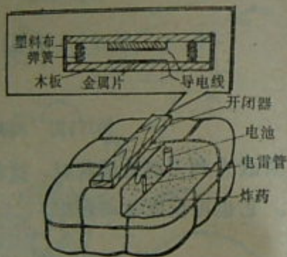
第121图 塑料布防坦克地雷
