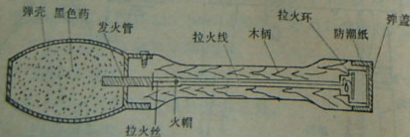
附13图 无雷管装黑色药手榴弹
