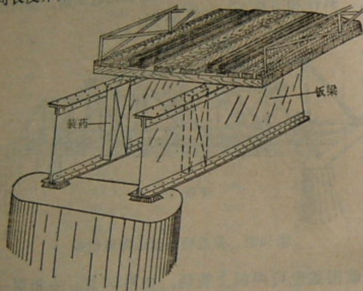
第58图 爆破钣梁装药的配置
