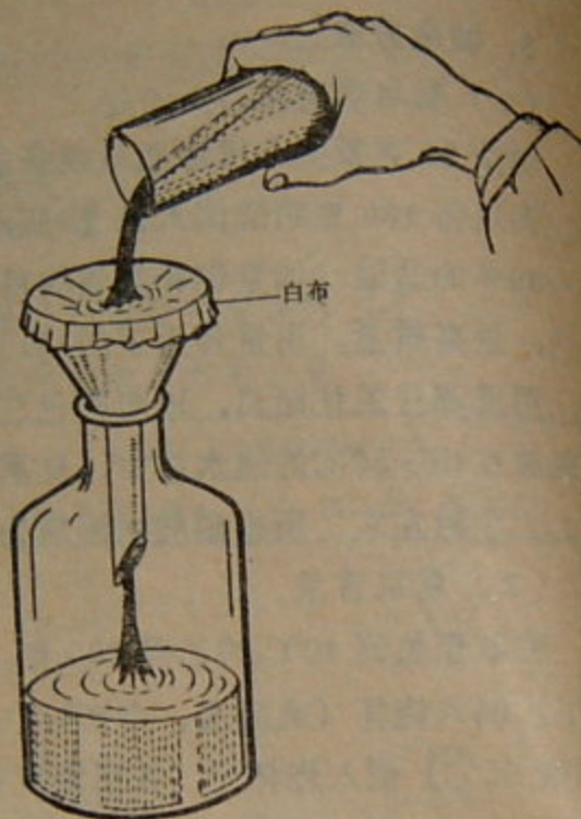
第11图 雷汞的过滤
