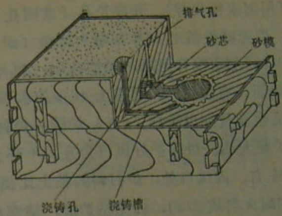
附7图 砂模
