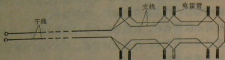
第33图 复式串联线路
