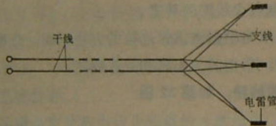
第34图 并联线路
