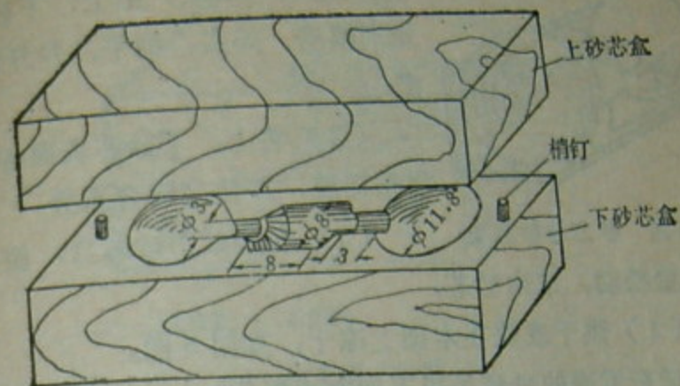
附3图 砂芯盒
