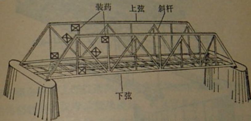
第56图 靠近桥脚附近爆破桁梁
