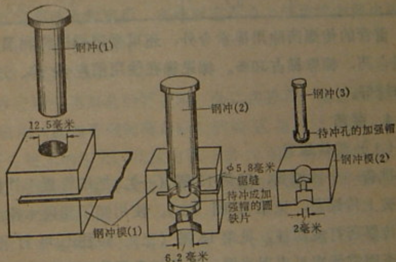
第14图 加强帽的冲制
