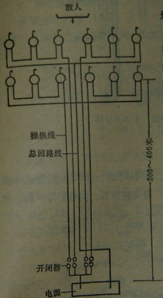
第107图 有线电操纵地雷群
