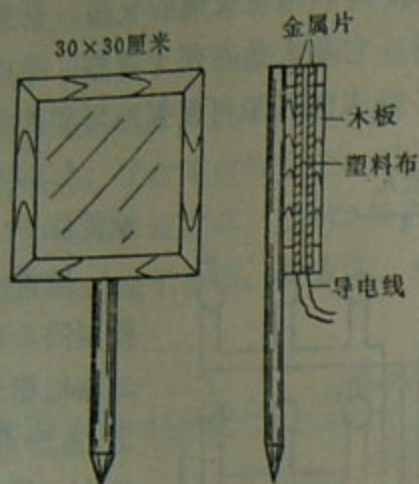
第108图 子弹开闭器
