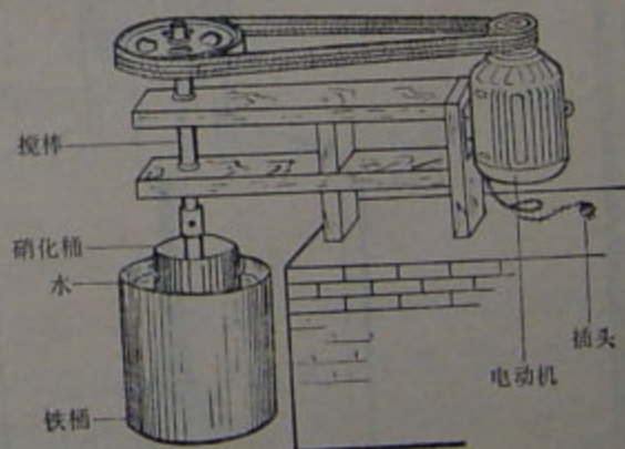
第 3 图 土硝化设备
