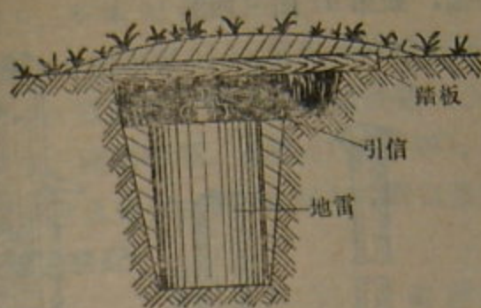
第 89 图 压发引信地雷的设置
