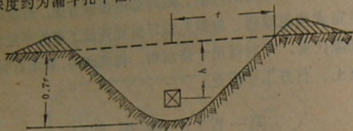
第65图 漏斗孔
