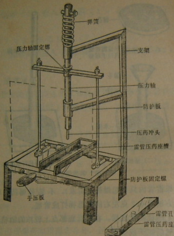
第16图 铁压力机
