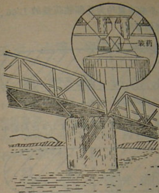
第59图 时间仓促时爆破钢桥装药的配置
