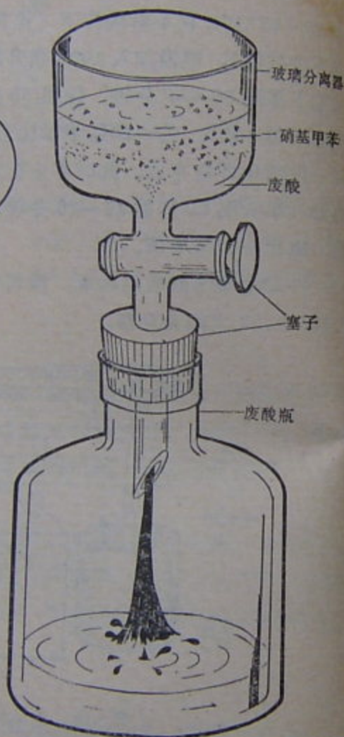
第5图 对硝化液的分离
