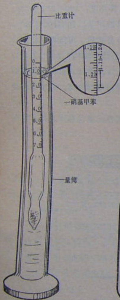
第4图 测一硝基甲苯比重
