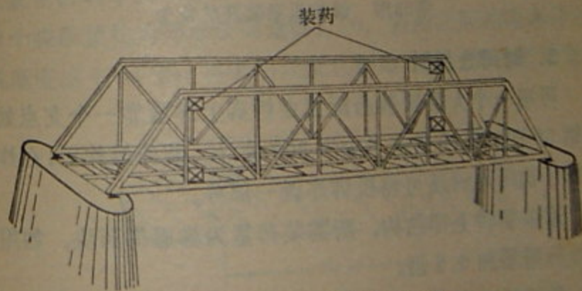
第57图 用四个装药爆破桁梁
