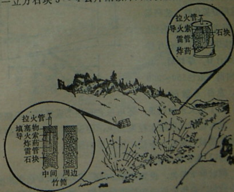
第94图 滚雷
