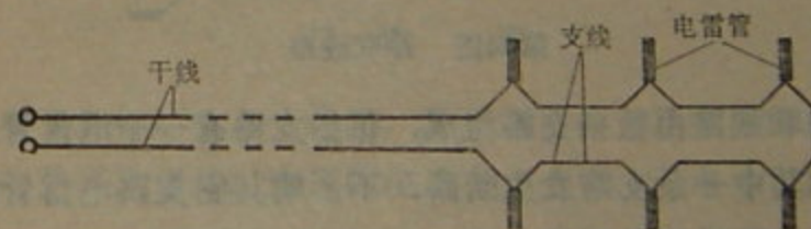
第32图 串联线路
