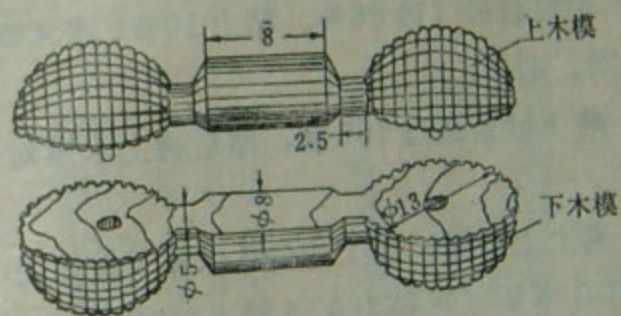
附4图 木模
