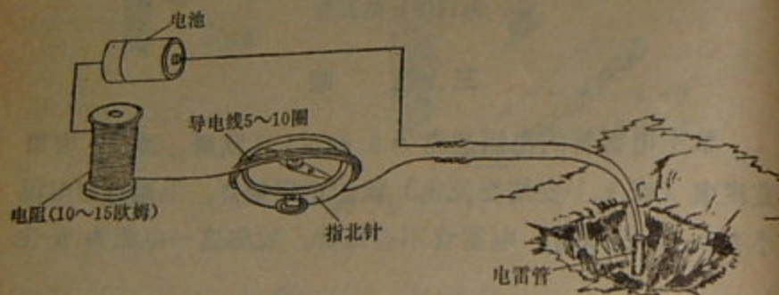
第19图 用指北针检查电雷管
