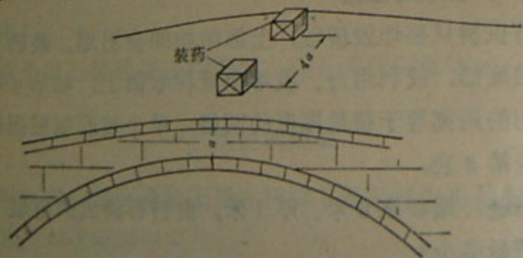
第50图 爆破拱顶装药的配置
