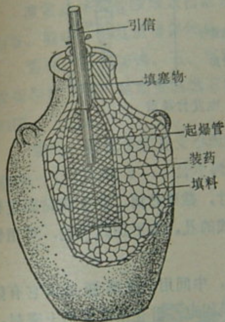
第92图 容器地雷
