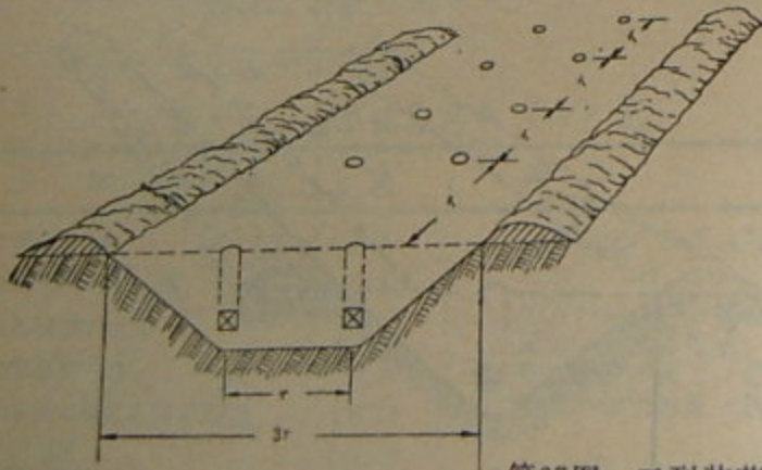
第67图 二列装药的配置
