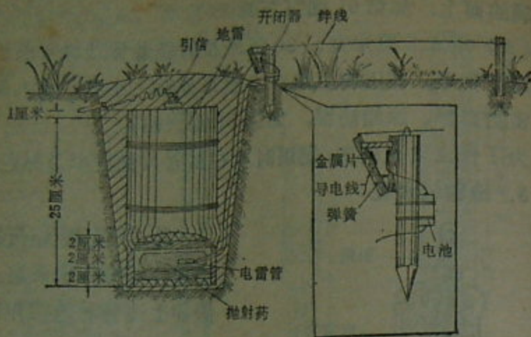
第93图 电发竹跳雷
