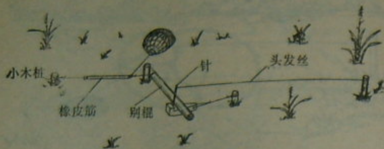
第102图 头发丝雷
