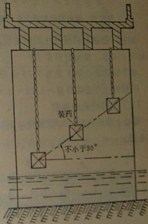
第51图 爆破钢筋混凝土桥墩装药的配置
