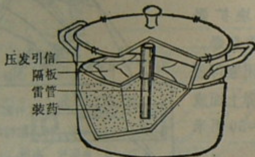
用铝锅改制的防坦克地雷 第123图 容器防坦克地雷
