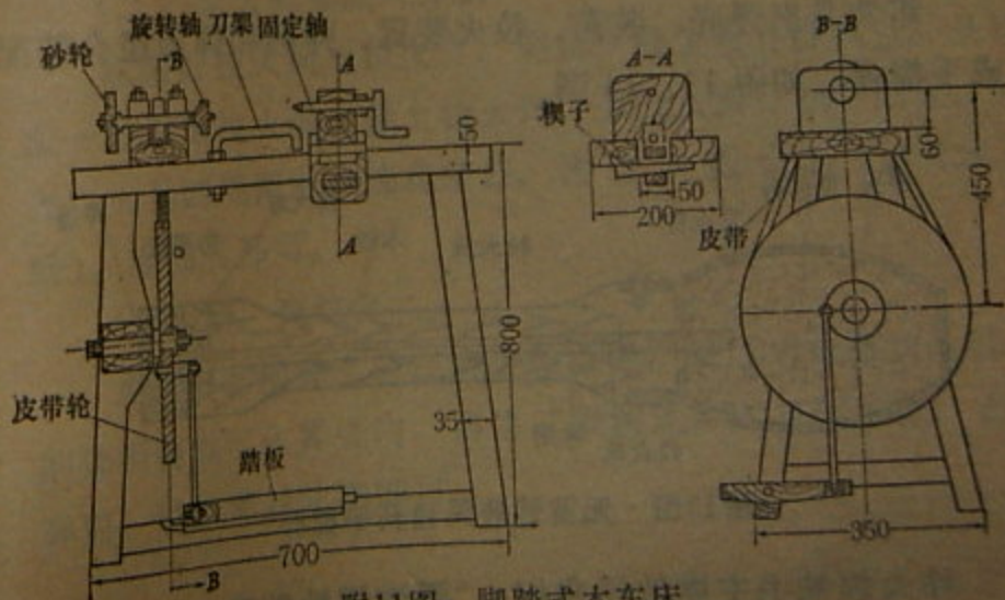
附11图 脚踏式木车床
