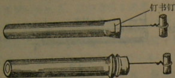
第28图 拉火管的装配
