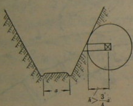
第44图 爆破一侧侧坡装药的配置
