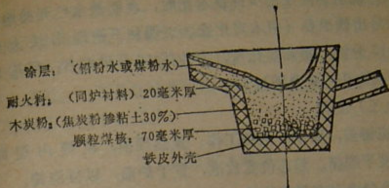
附 10 图 炉底（勺）
