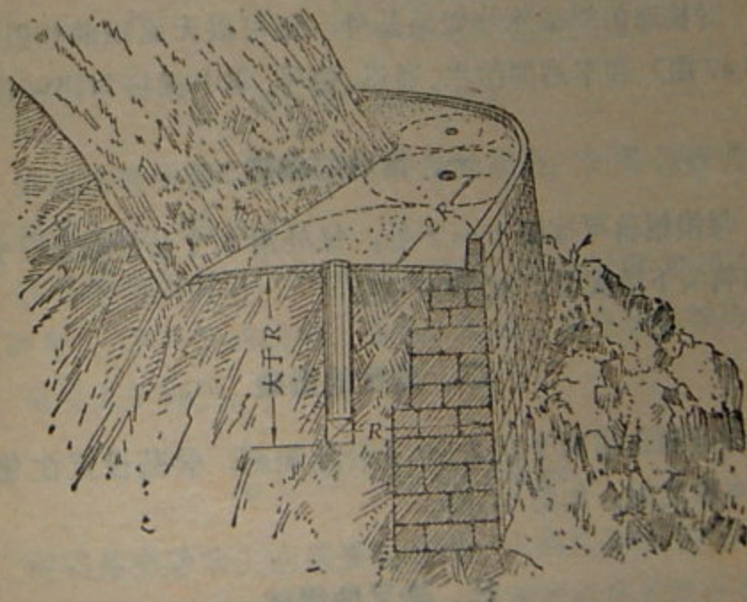
第46图 爆破山腹道挡土墙装药的配置
