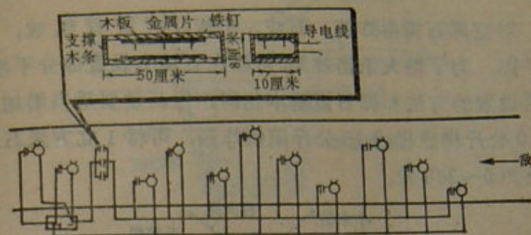
第126图 电发雷群
