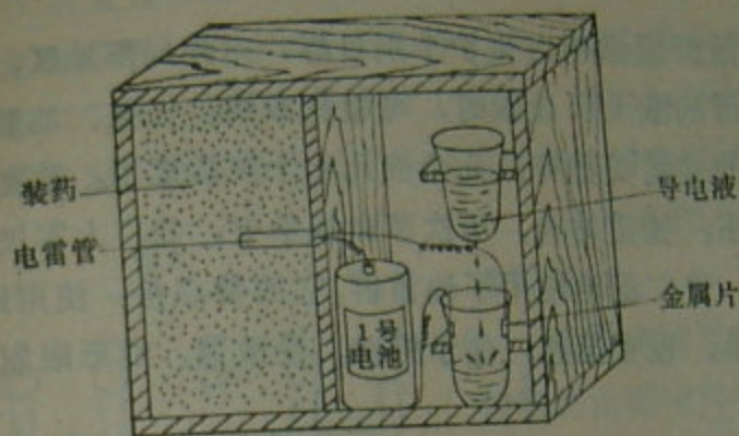
第104图 延期地雷
