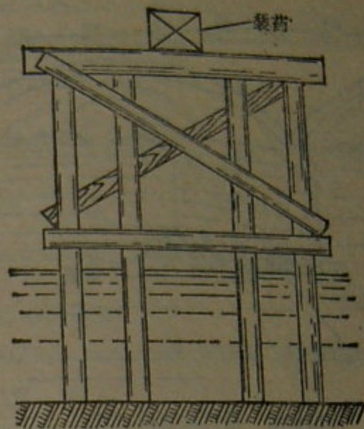
第48图 爆破木桥装药的配置
