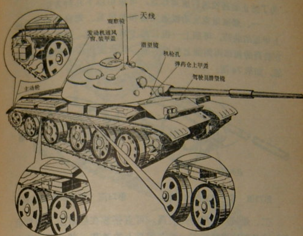
第72图 爆破敌坦克的装药投送位置
