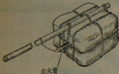
第73图 带一根木棍的装药
