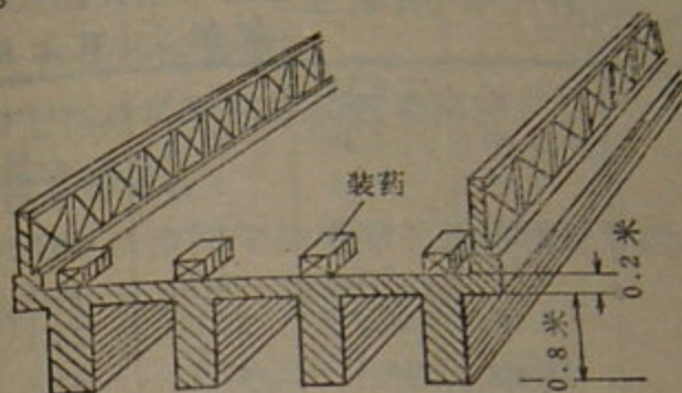
第54图 装药配置在桥面上
