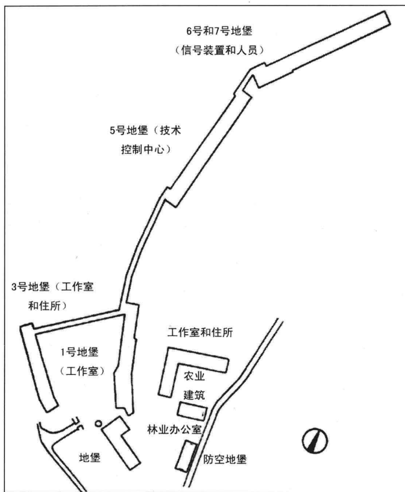
Ziegenberg的地堡建筑群
