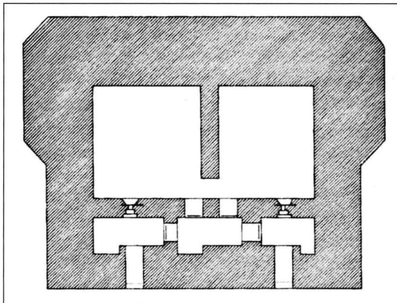
102V型“双人房”式地堡，B版
