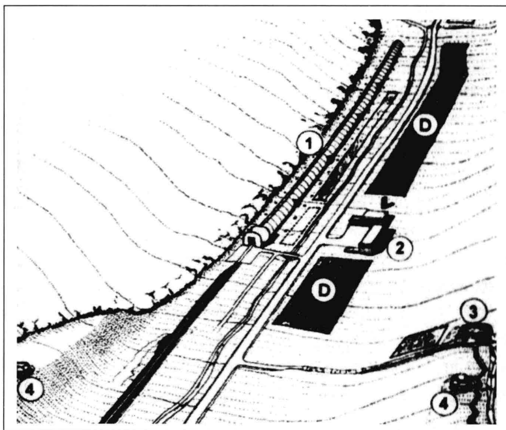
一位画家描绘出的对Frysztak（Kuhn之后）受保护火车侧线的印象。管状列车棚完整无缺。①.管状混凝土列车棚；②.机器房和泵房；③.混凝土地堡；④.混凝土防护穹顶；D. Frysztak村。
