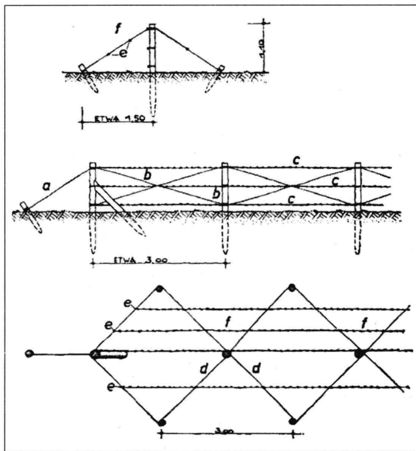
“佛兰德斯篱墙”作为一个战地障碍物的施工方法（出自1942年，第II部分）。a.后锚；b.由拉紧的平滑金属丝支撑的中部支柱；c.水平长度的带刺铁丝网，接近地面以阻挡任何人从下面爬进来；d.小型支柱的带有细金属丝的横向锚固装置；e.带刺软铁丝网的横向长度；f.敌人位置。
