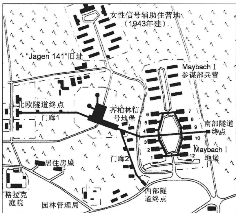
Maybach I 布局图
