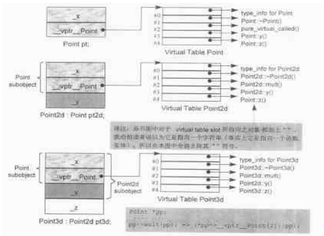
图 4.1 Virtual Table 的布局：单一继承情况
