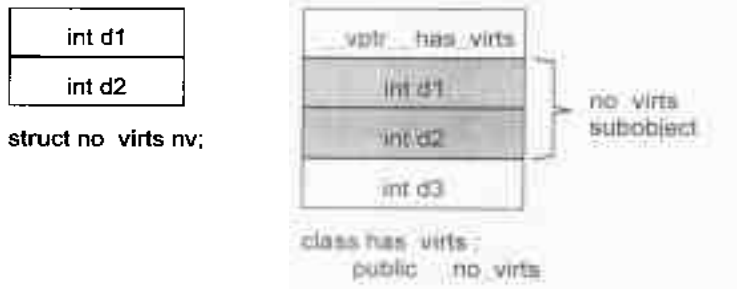
图 3.2b Vptr 被放在 class 的前端
