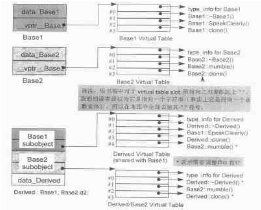
图 4.2 Virtual Table 的布局：多重继承情况。 (译注：右下角的三个星号，就是下页的三种情况)
