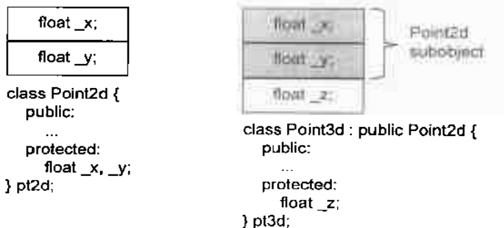
图 3.1b 单一继承而且没有 virtual function 时的数据布局
