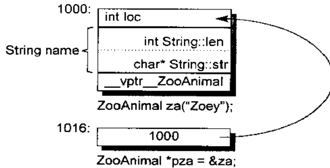
图 1.4 独立 (非派生) class 的 object 布局和 pointer 布局
