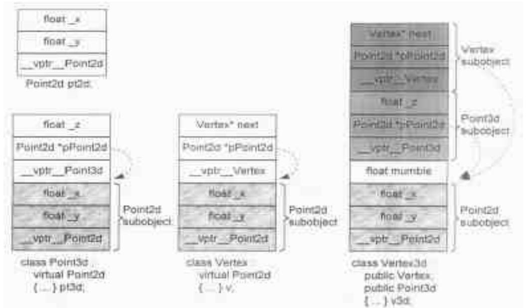
图 3.5a 虚拟继承, 使用 Pointer Strategy 所产生的数据布局 (译注: 原书图 3.5a 把 Vertex 写为 Vertex2d , 与书中程序代码不符, 所以我全部改为 Vertex )
