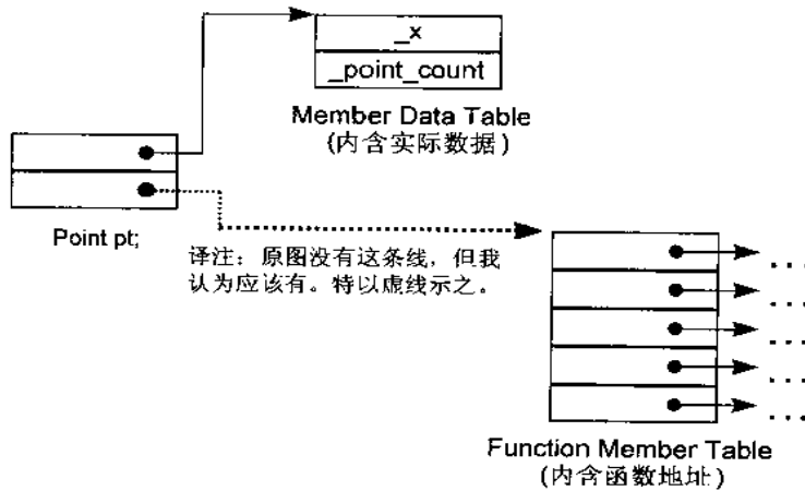
图 1.2 Member Table 对象模型 (Member Table Object Model)
