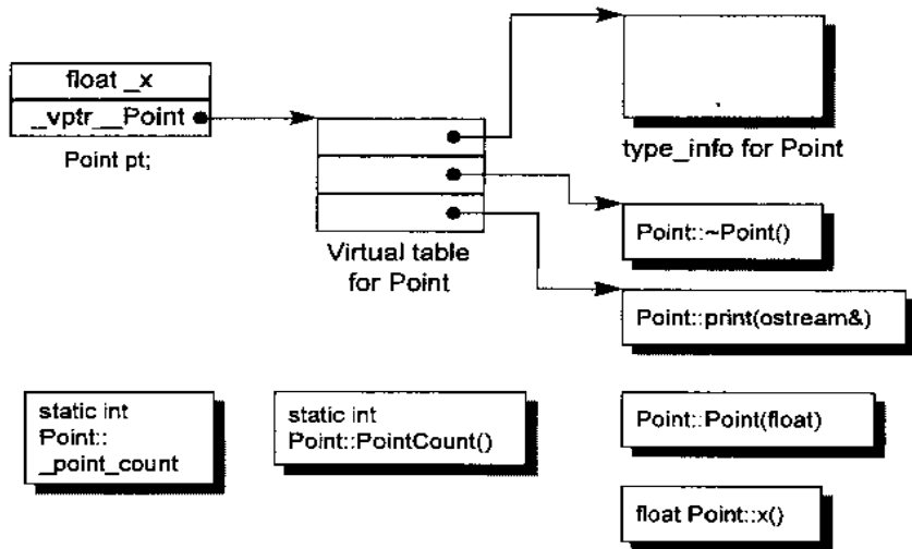
图 1.3 C++ 对象模型 (C++ Object Model)
