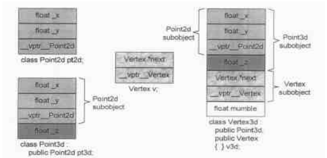
图 3.4 数据布局: 多重继承 (Multiple Inheritance)
