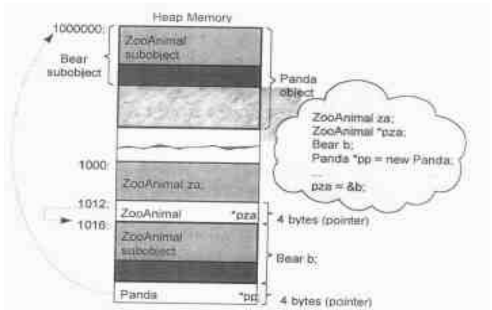
图 1.6 依次定义得到的内存布局
