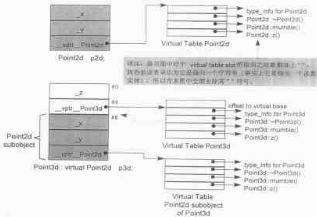
图 4.3 Virtual Table 布局：虚拟继承情况。（译注：我个人对于图右下的两个 vtbls 内容感到相当疑惑。至少，mumble() 应该是 Point2d::mumble() 而非 Point3d::mumble()）
