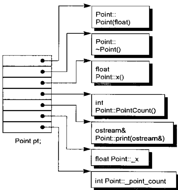
图 1.1 简单对象模型 (Simple Object Model)
