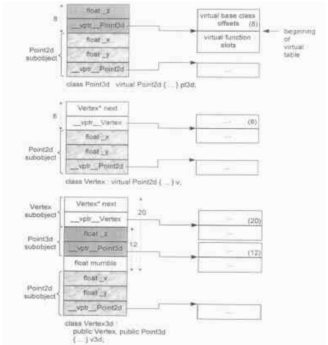
图 3.5b 虚拟继承，使用 Virtual Table Offset Strategy 所产生的数据布局（译注：原书图 3.5b 把 Vertex 写为 Vertex2d ，与书中程序代码不符，所以我全部改为 Vertex ）
