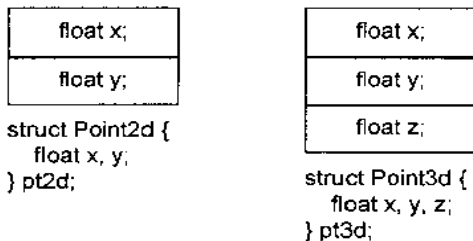
图 3.1a 个别 structs 的数据布局
