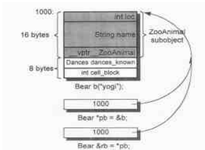
图 1.5 Derived class 的 object 和 pointer 布局
