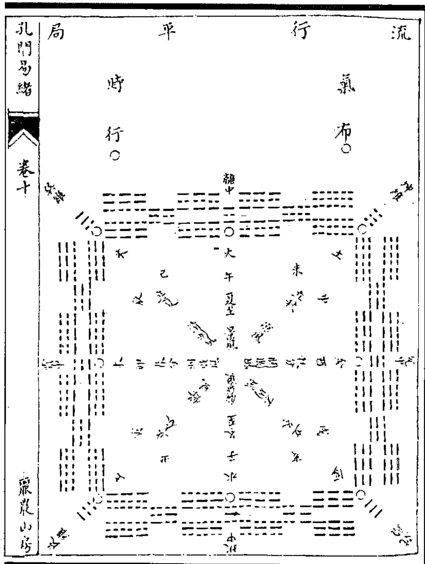
图 318 流行平局图
