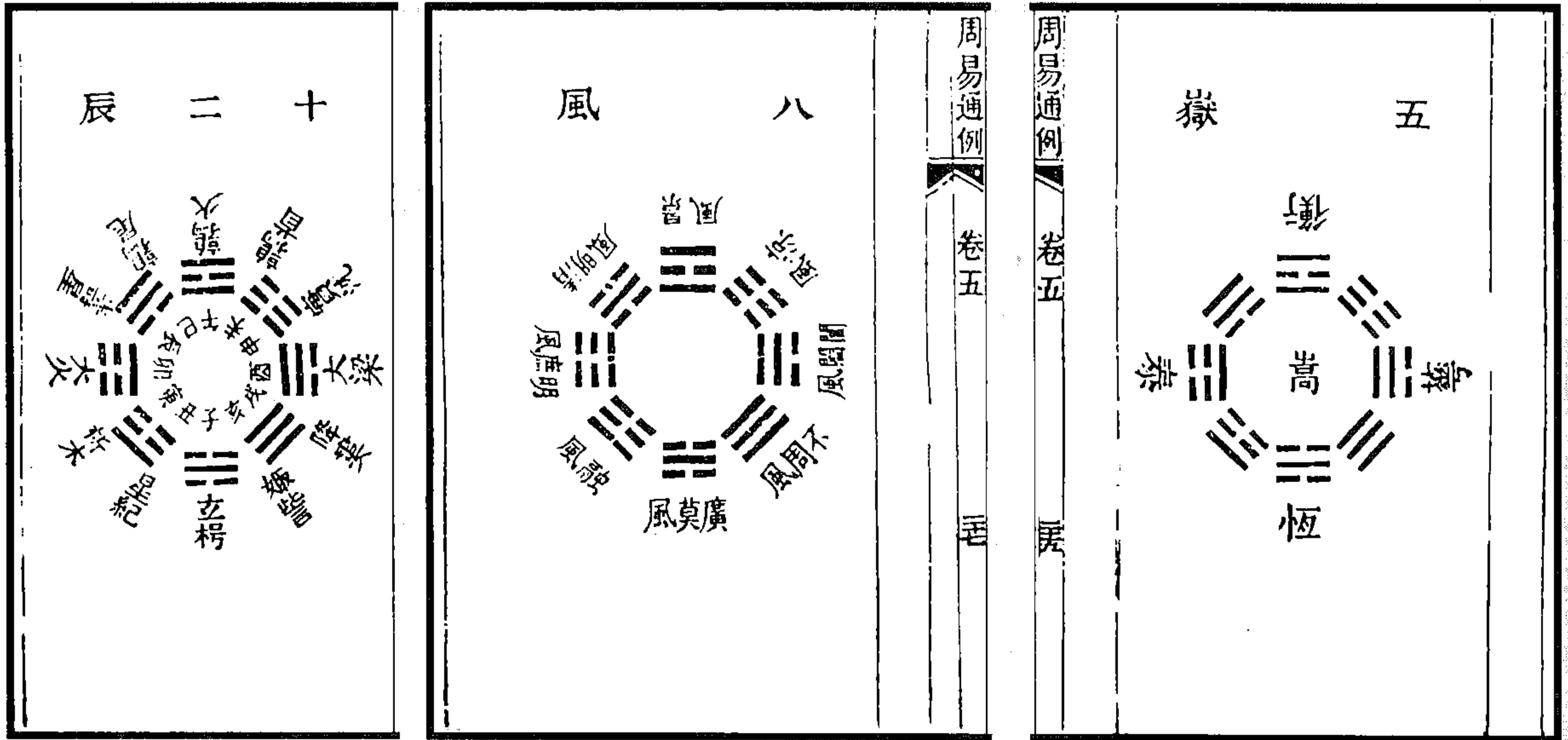
图 109 十二辰图
