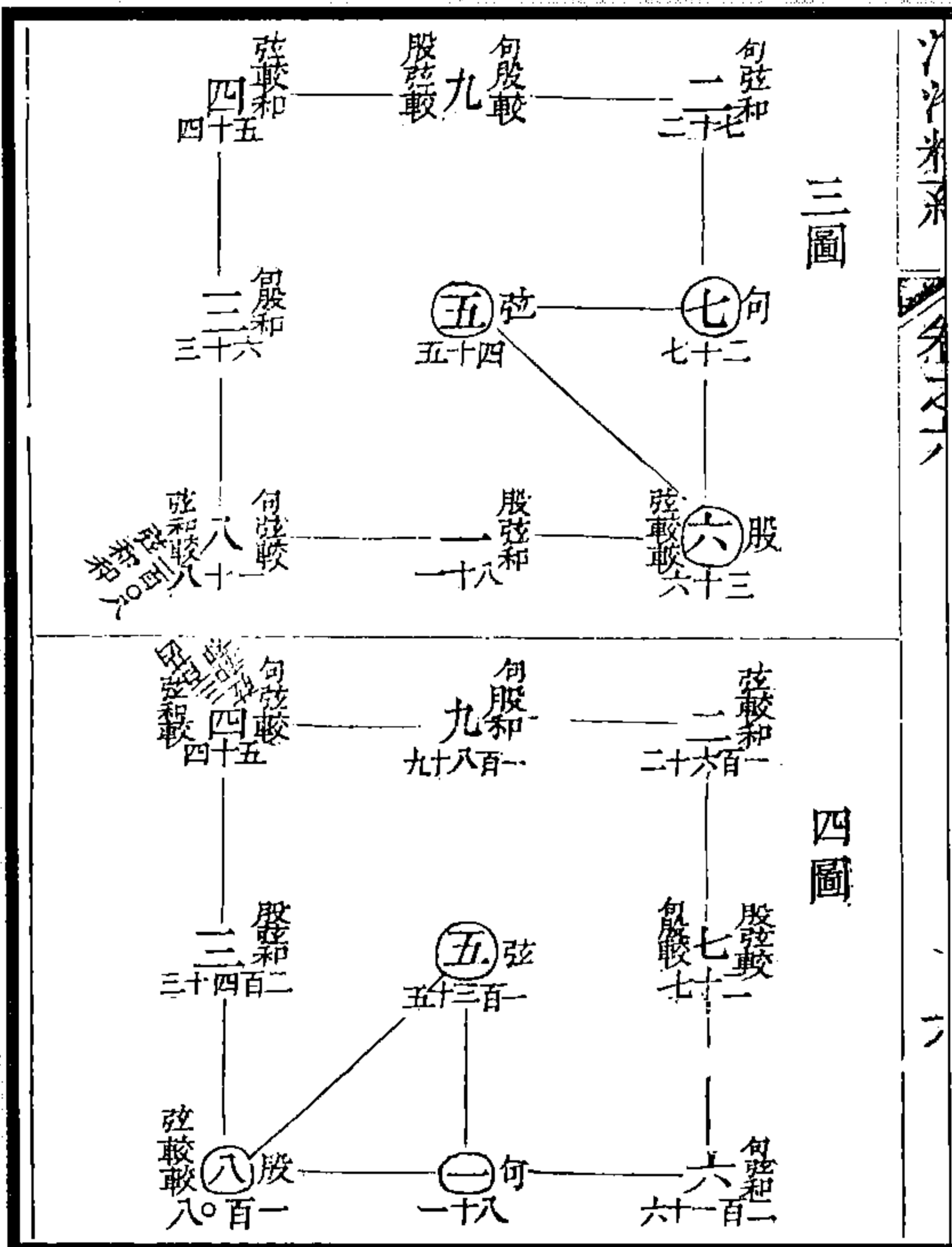
图 101 洛书勾股四图
