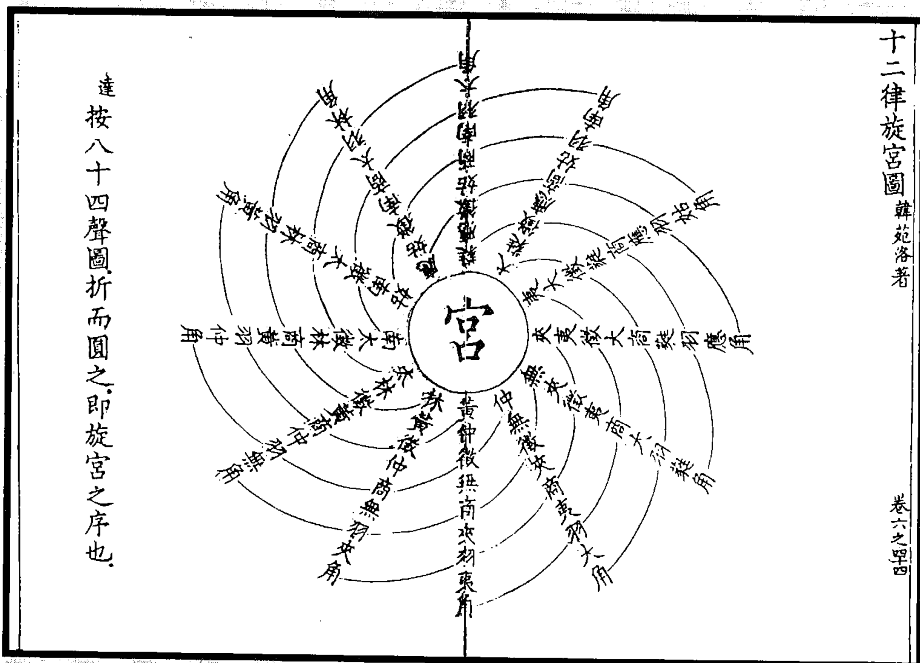
图 52 十二律旋宫图
