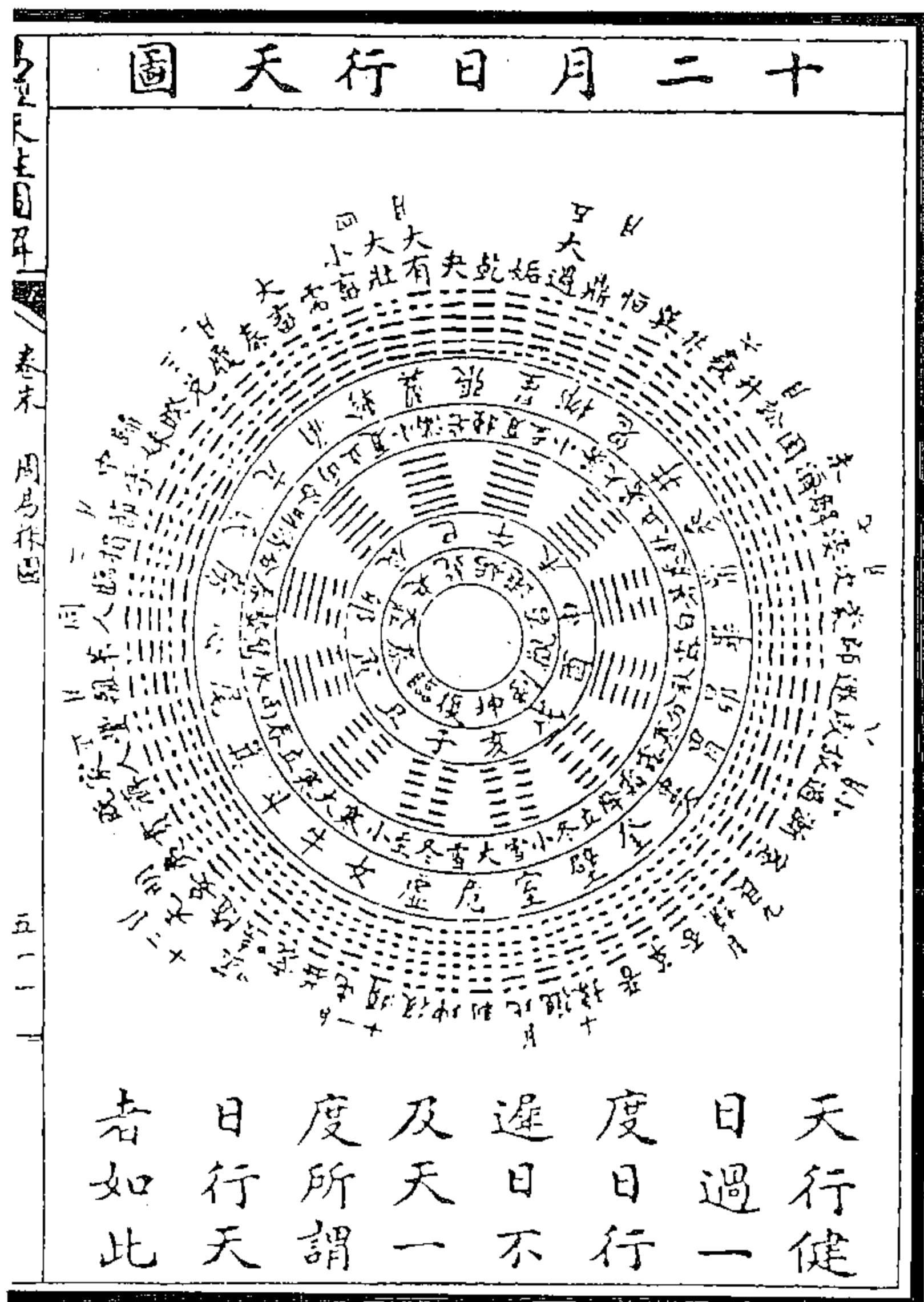
图 426 十二月日行天图
