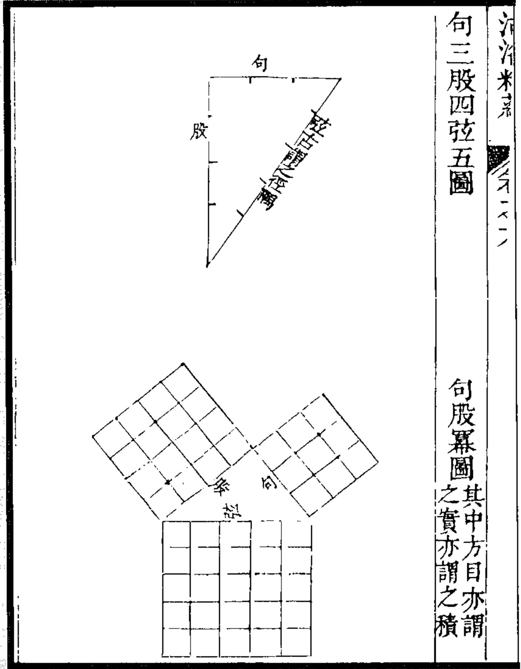
图 99 勾股二图
