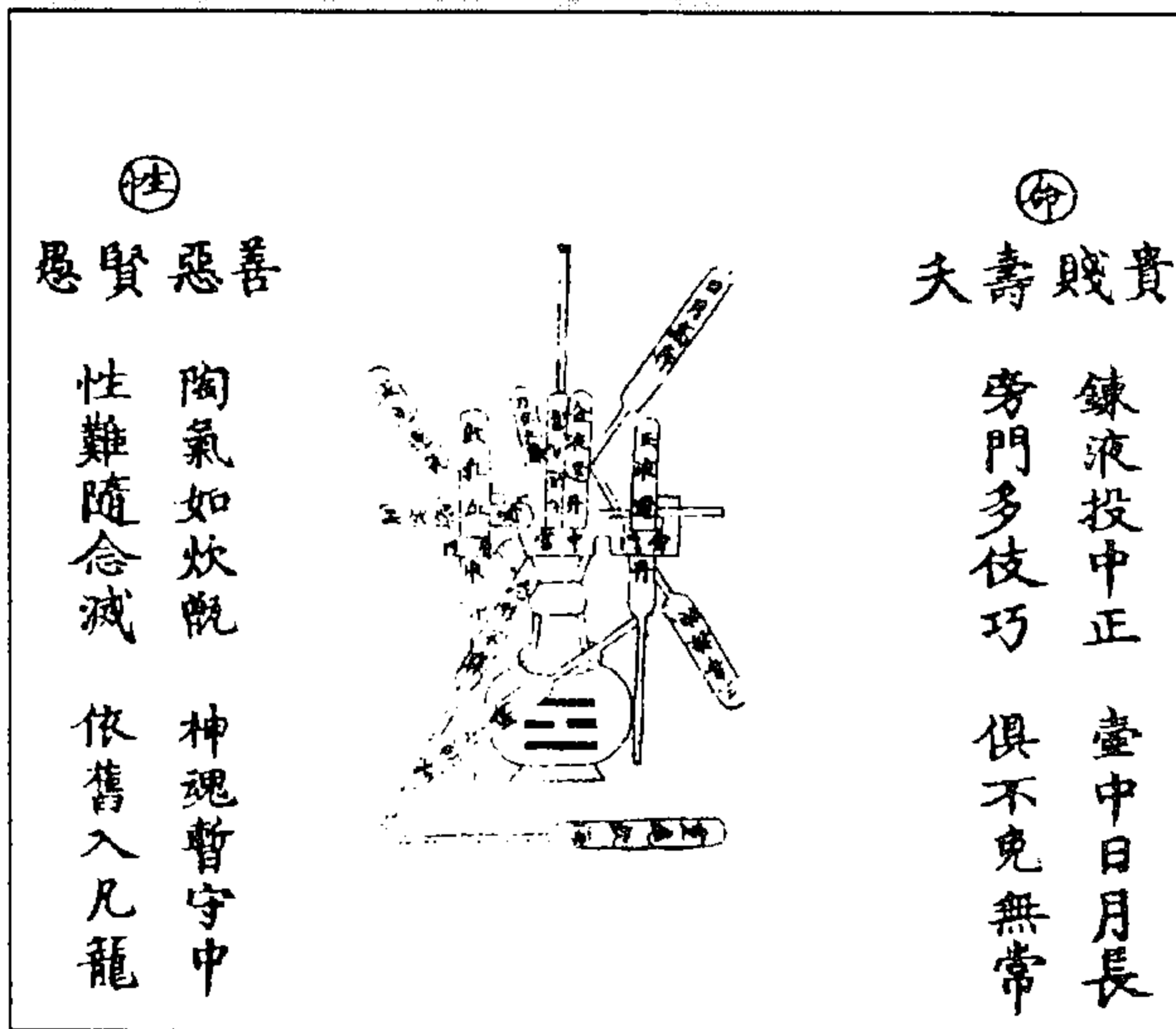
图 37 性命图
