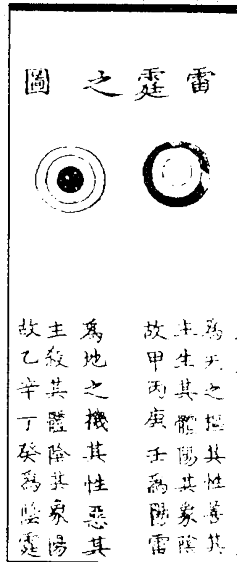
图 119 雷霆图
