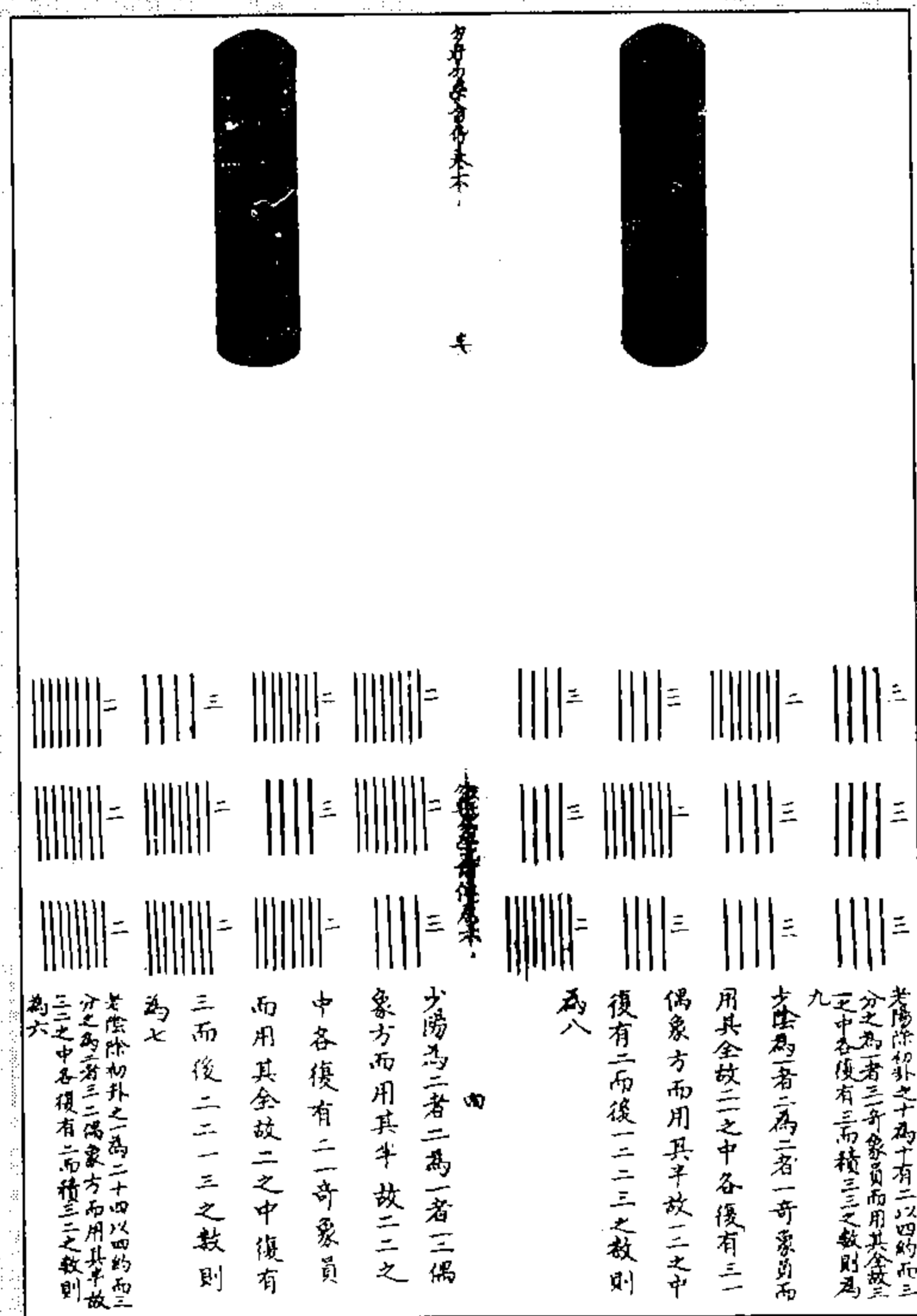
图 21 挂扐筒图
