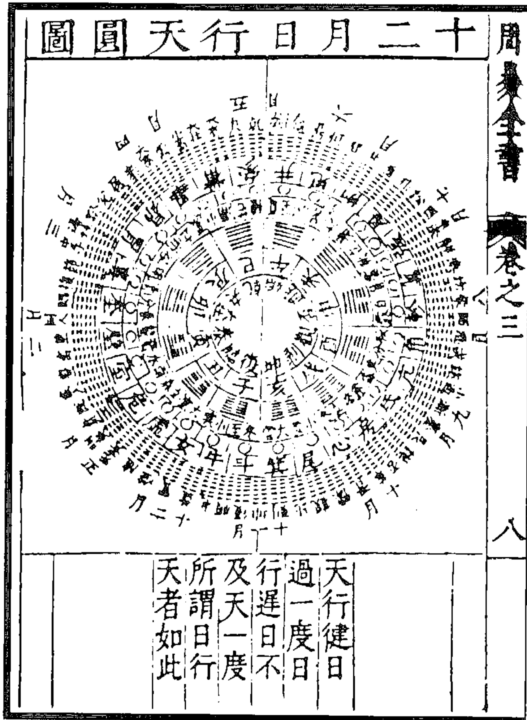
图 280 十二月日行天圆图
