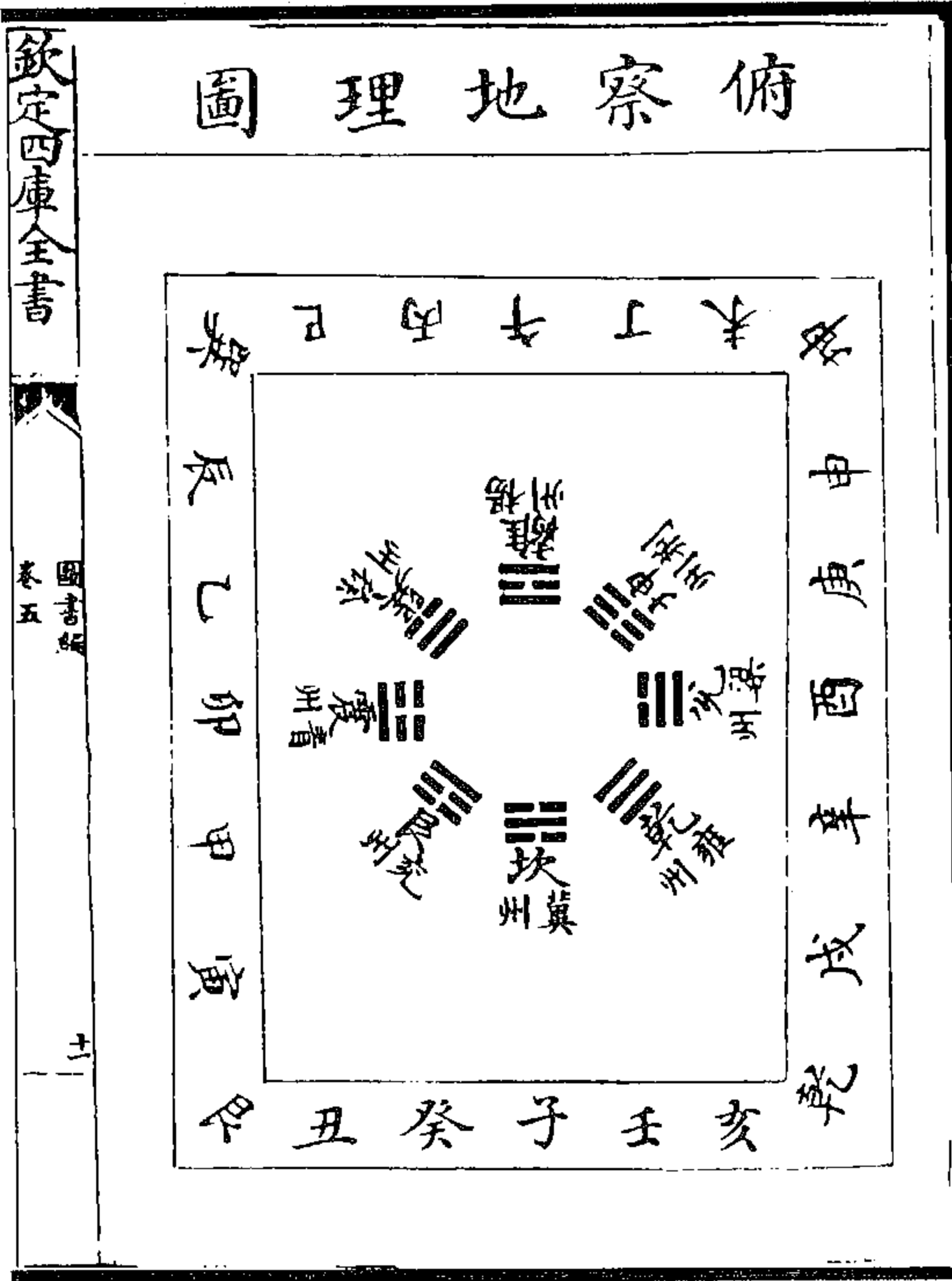
图 53 俯察地理图
