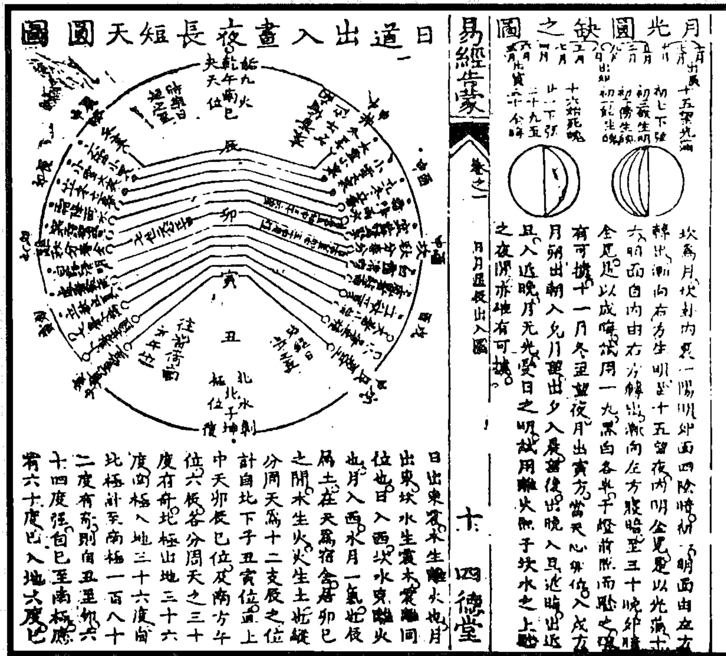
图 81 日道出入昼夜长短天圆图 图 80 月光圆缺图 (赵世迥《易经告蒙》)
