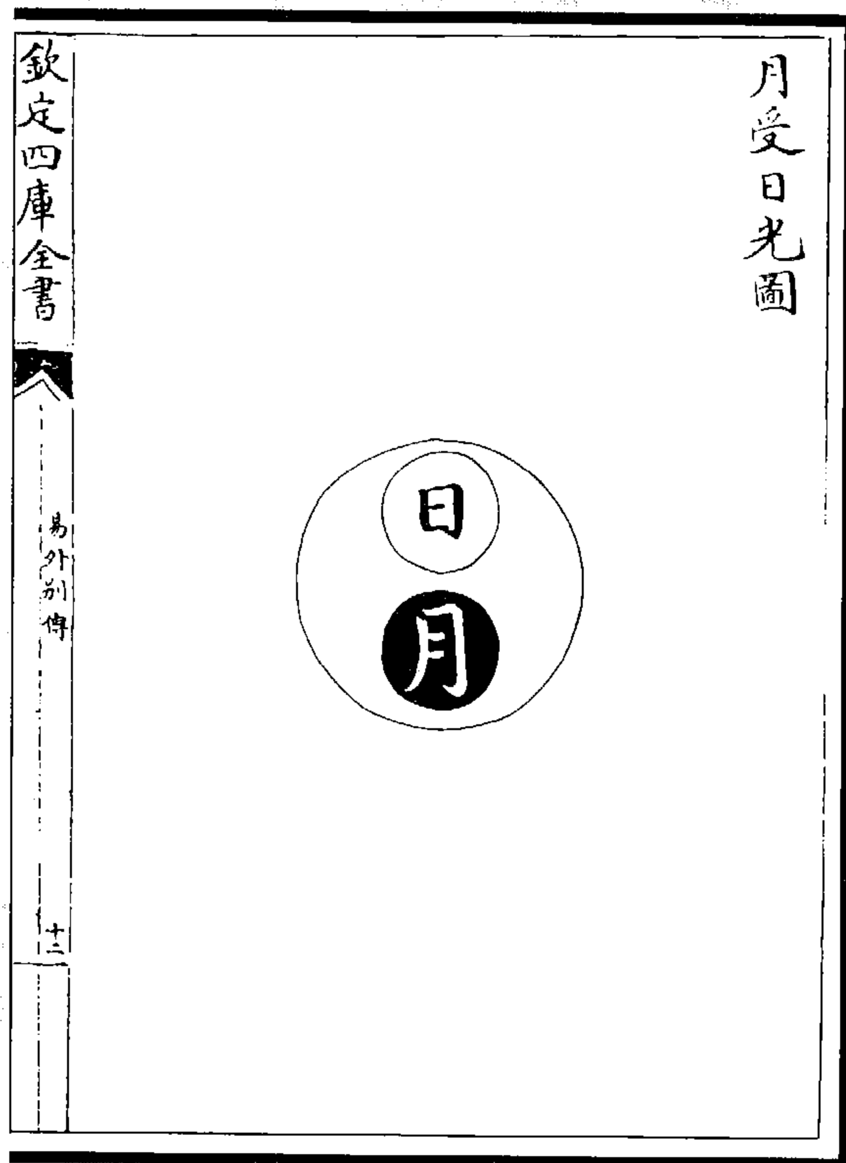
图 146 月受日光图
