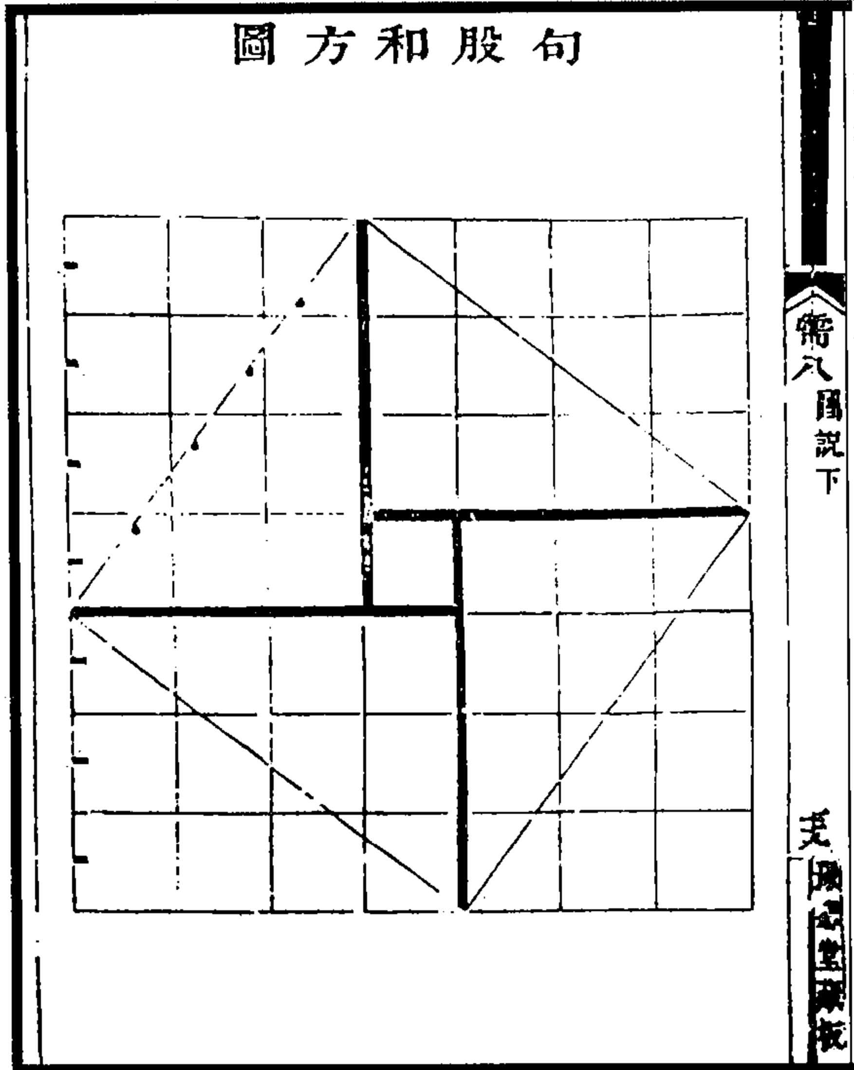
图 175 勾股和方图
