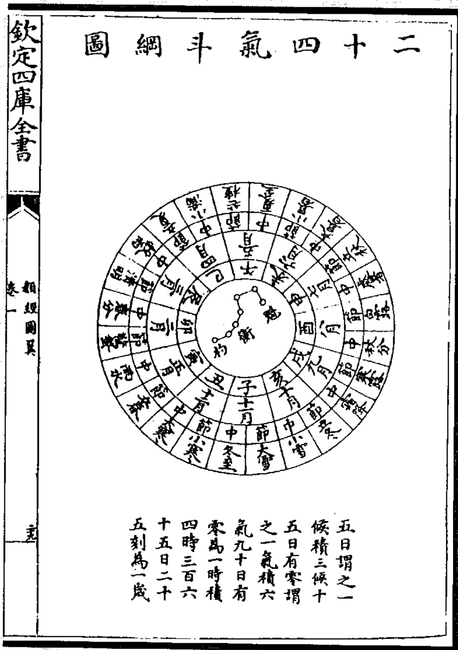
图 28 二十四气斗綱圖 (张介宾《类经图翼》)
