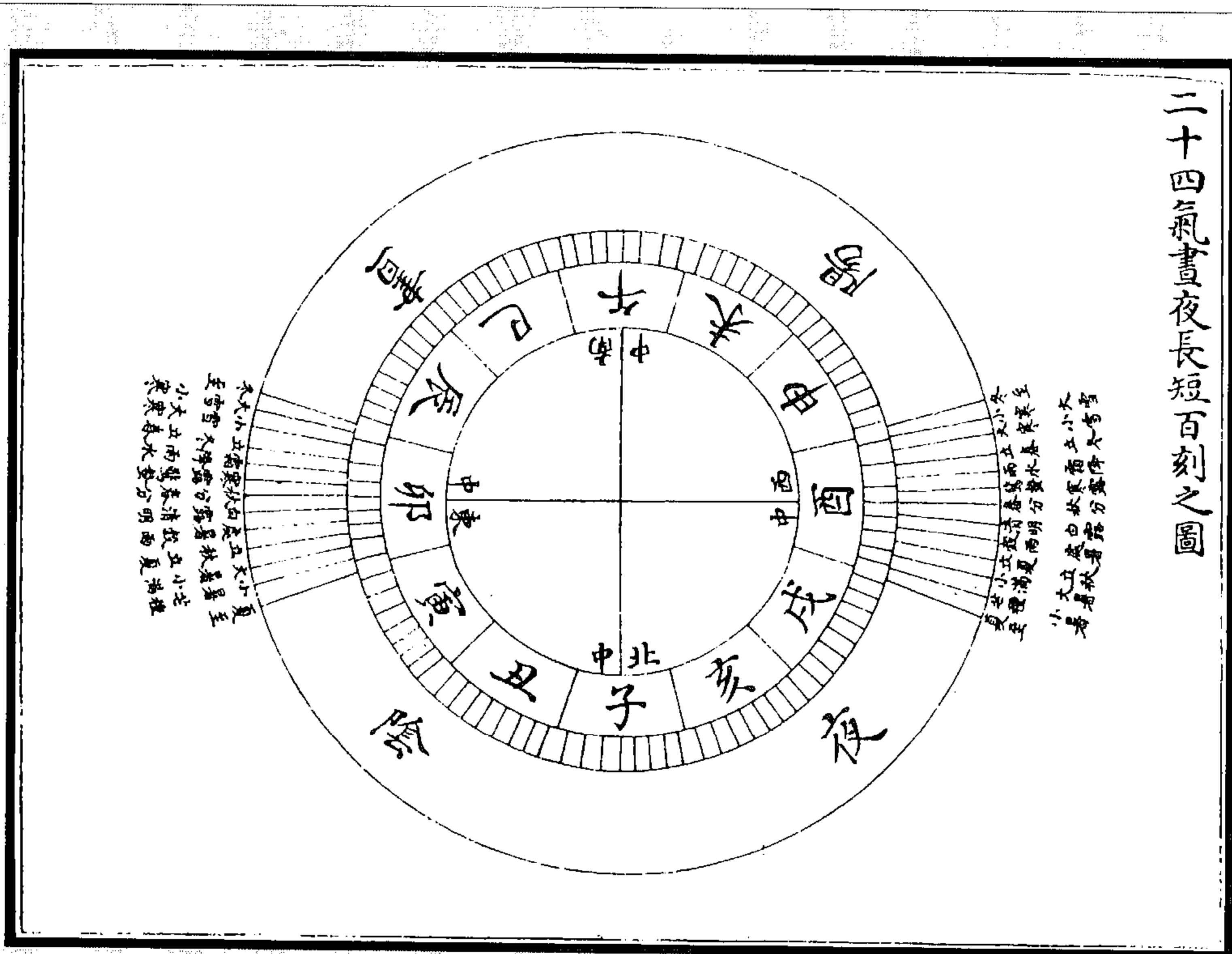
图 27 二十四气晝夜長短百刻之圖 (张介宾《类经图翼》)
