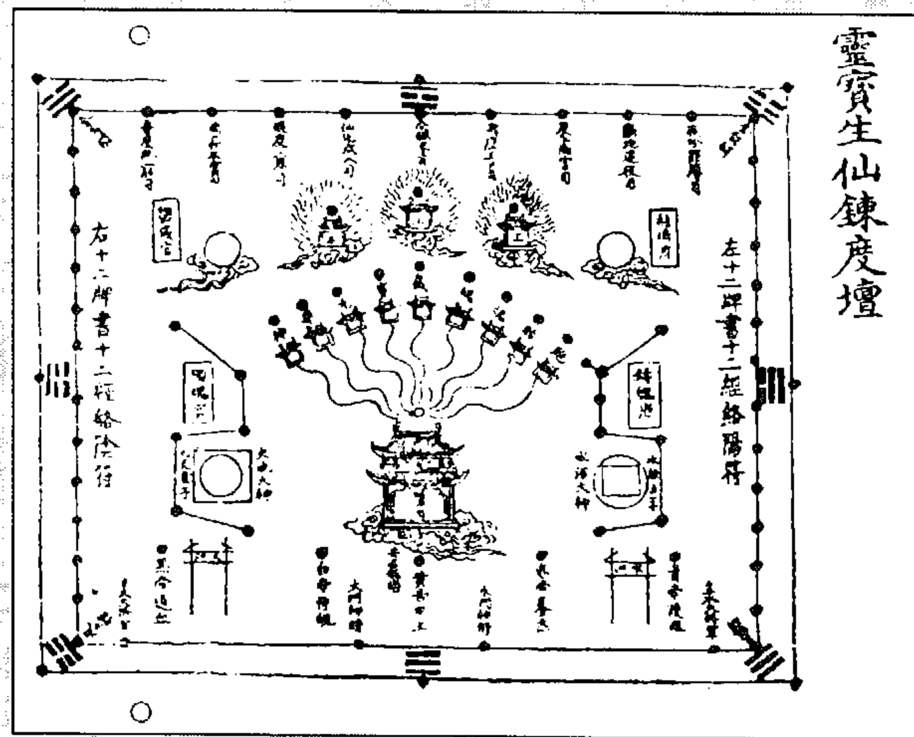
图 115 灵宝生仙炼度坛图
