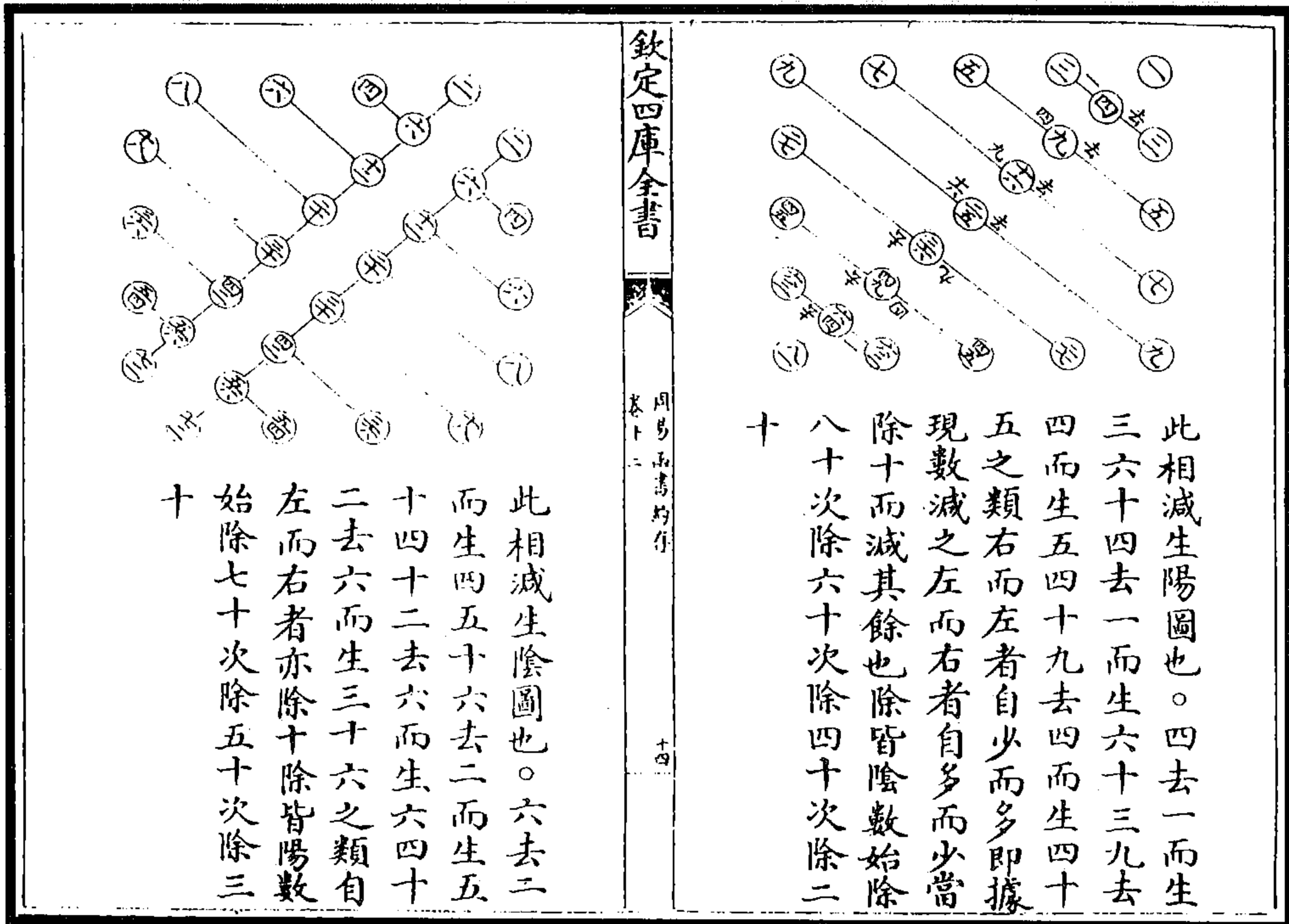
图 110 相減生陰圖
