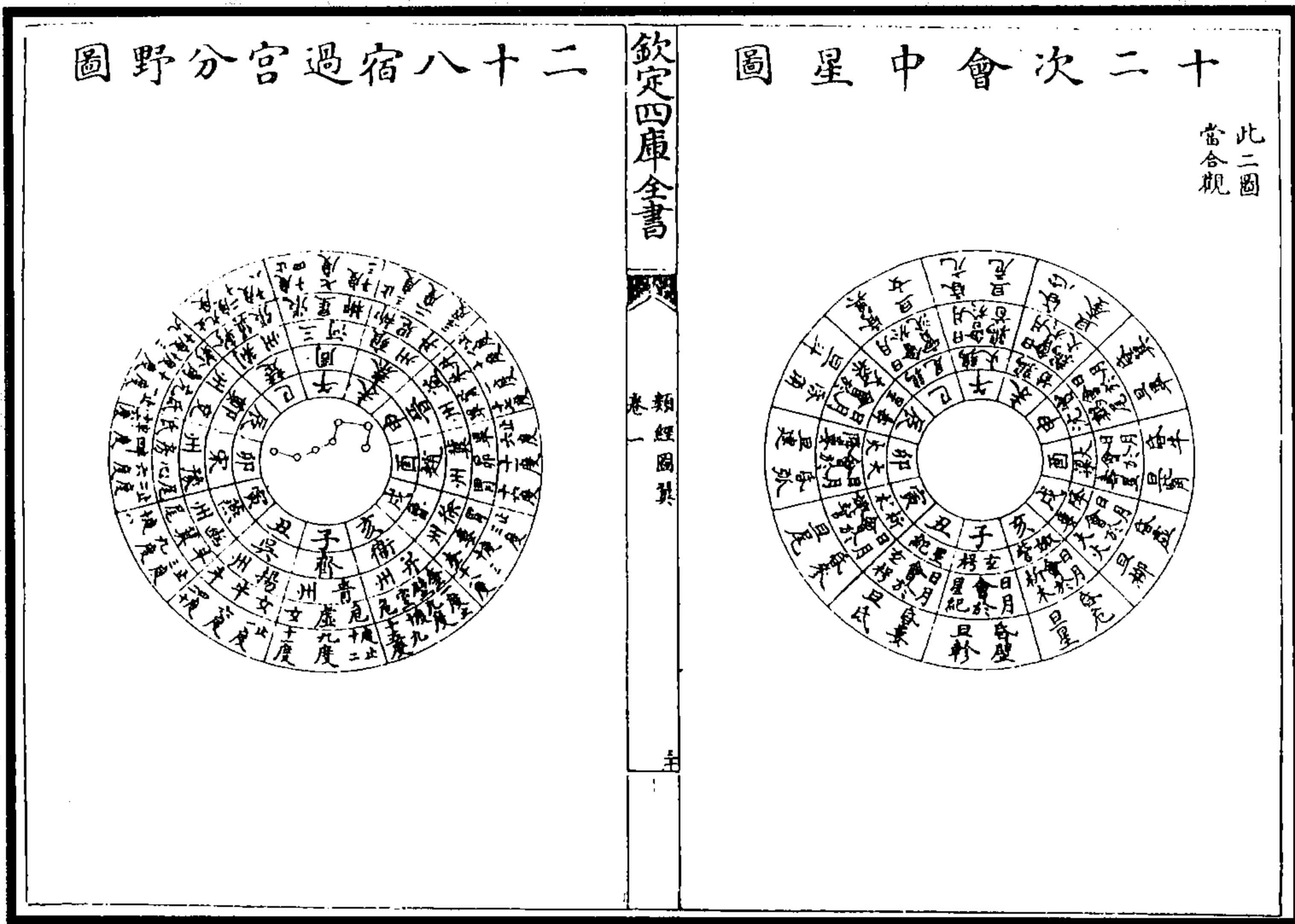
图 30 二十八宿过宫分野图
