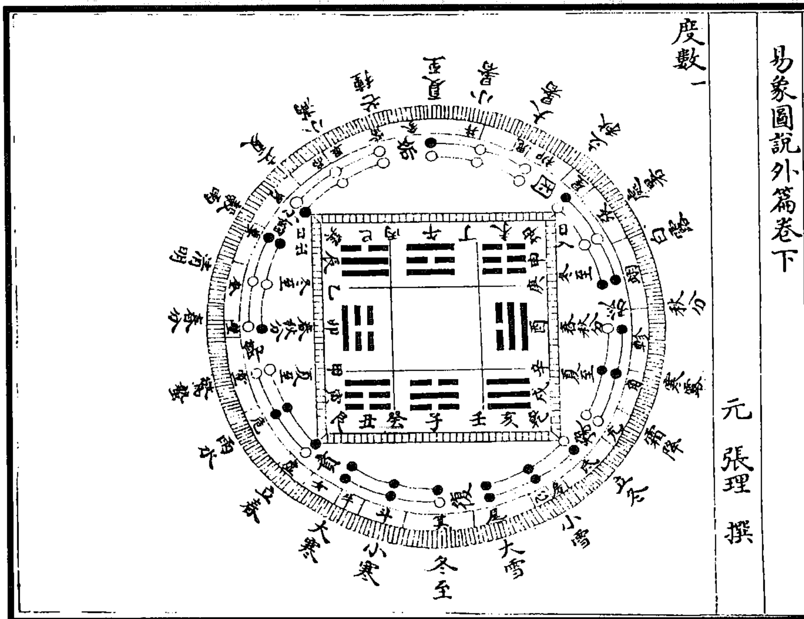
图 43 周天历象气节之图
