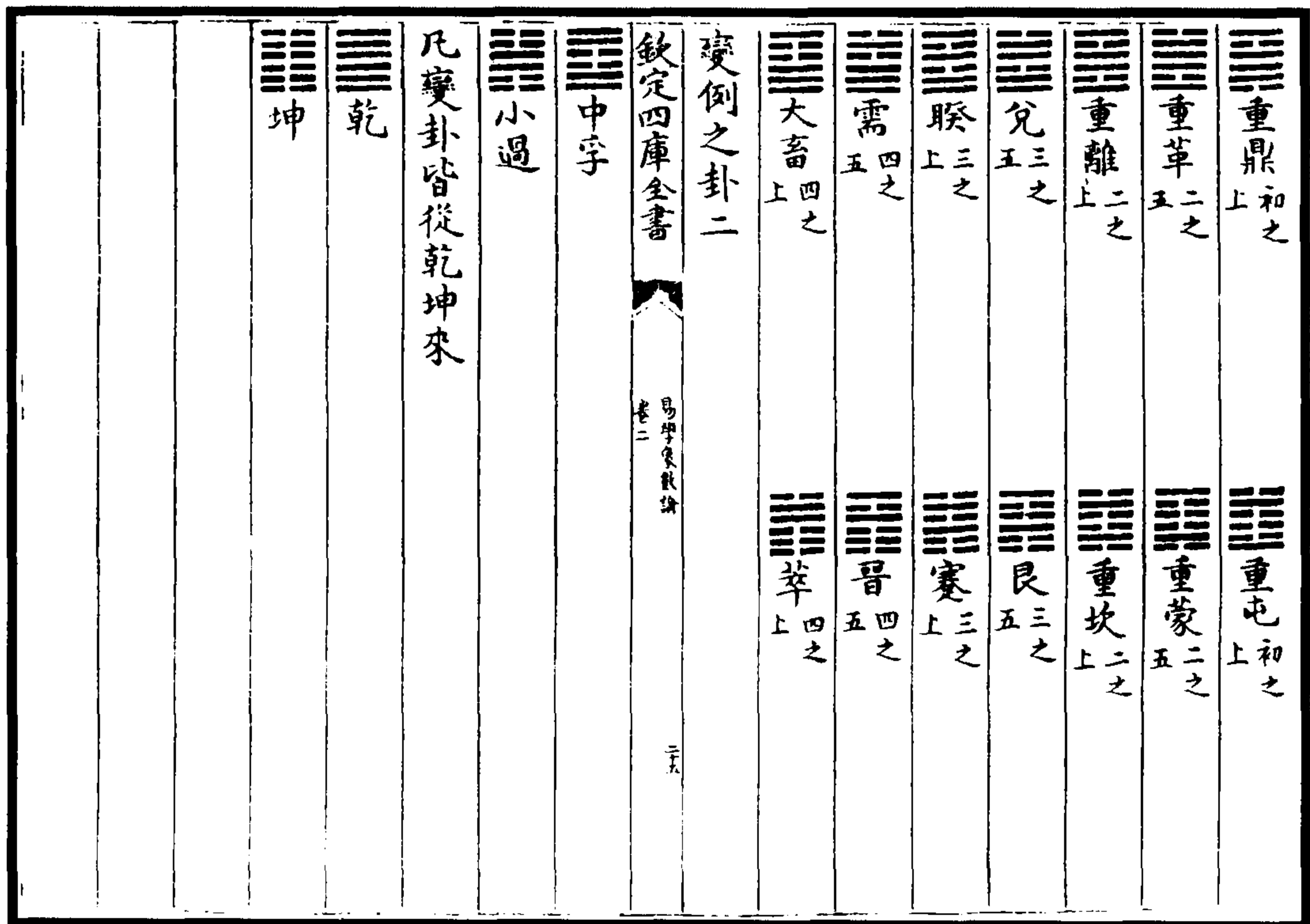
图 70 古卦变图
