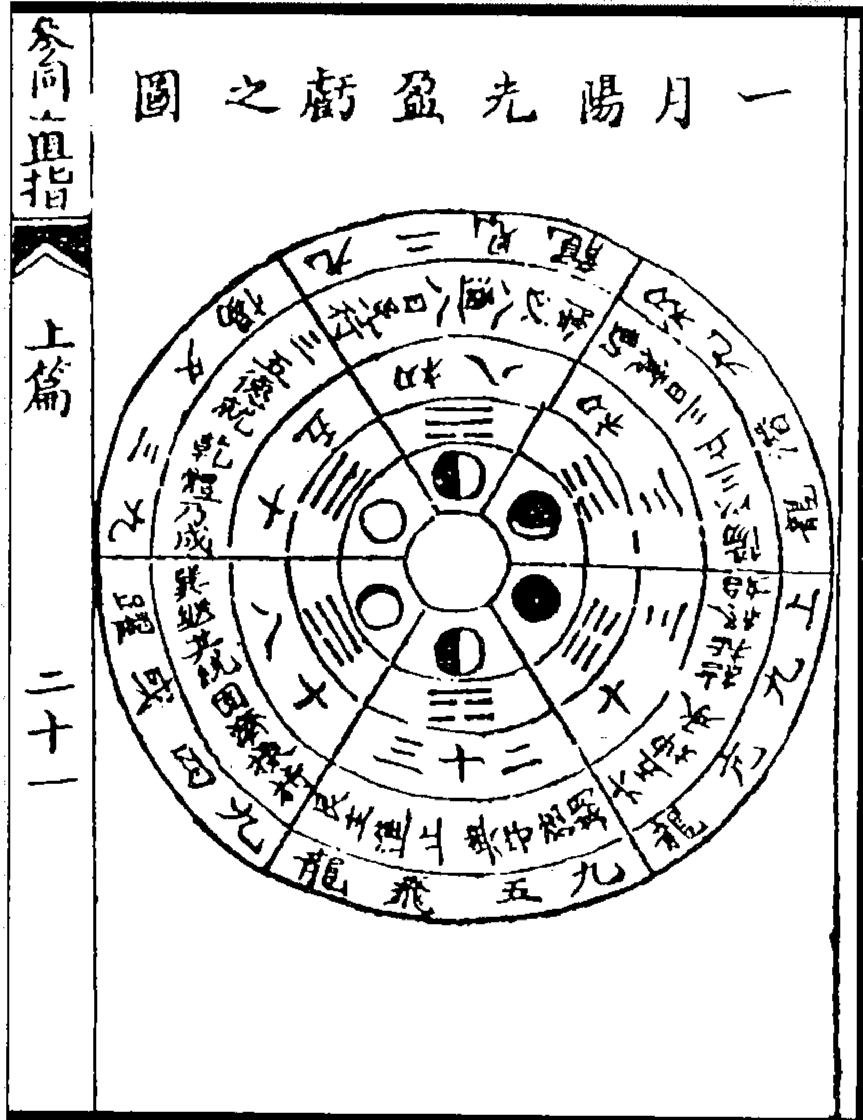
图 92 一月阳光盈亏图
