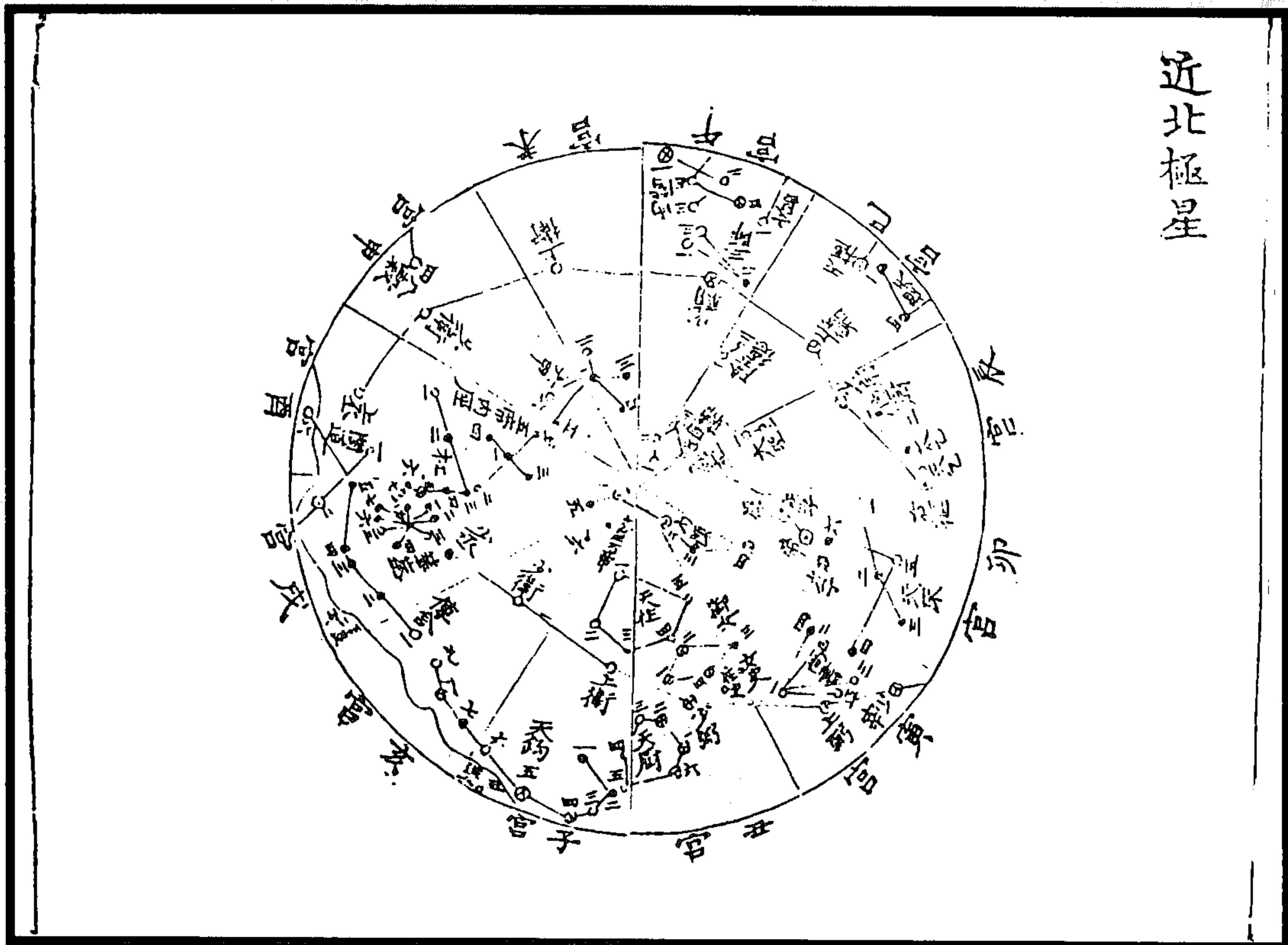
图 110 近北极星图
