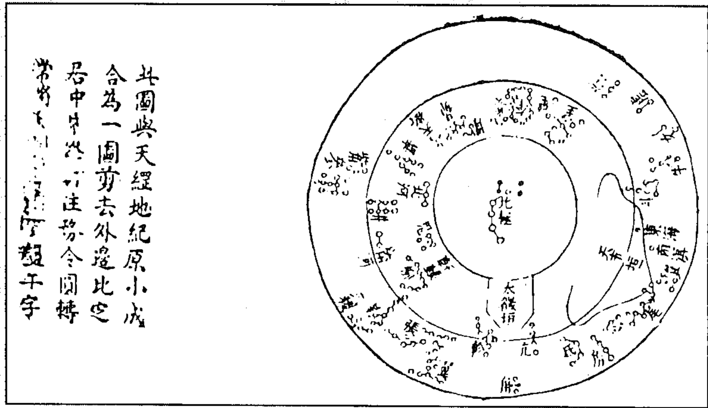
图 70 《易原》卷首天文图 (赵振芳《易原》)
