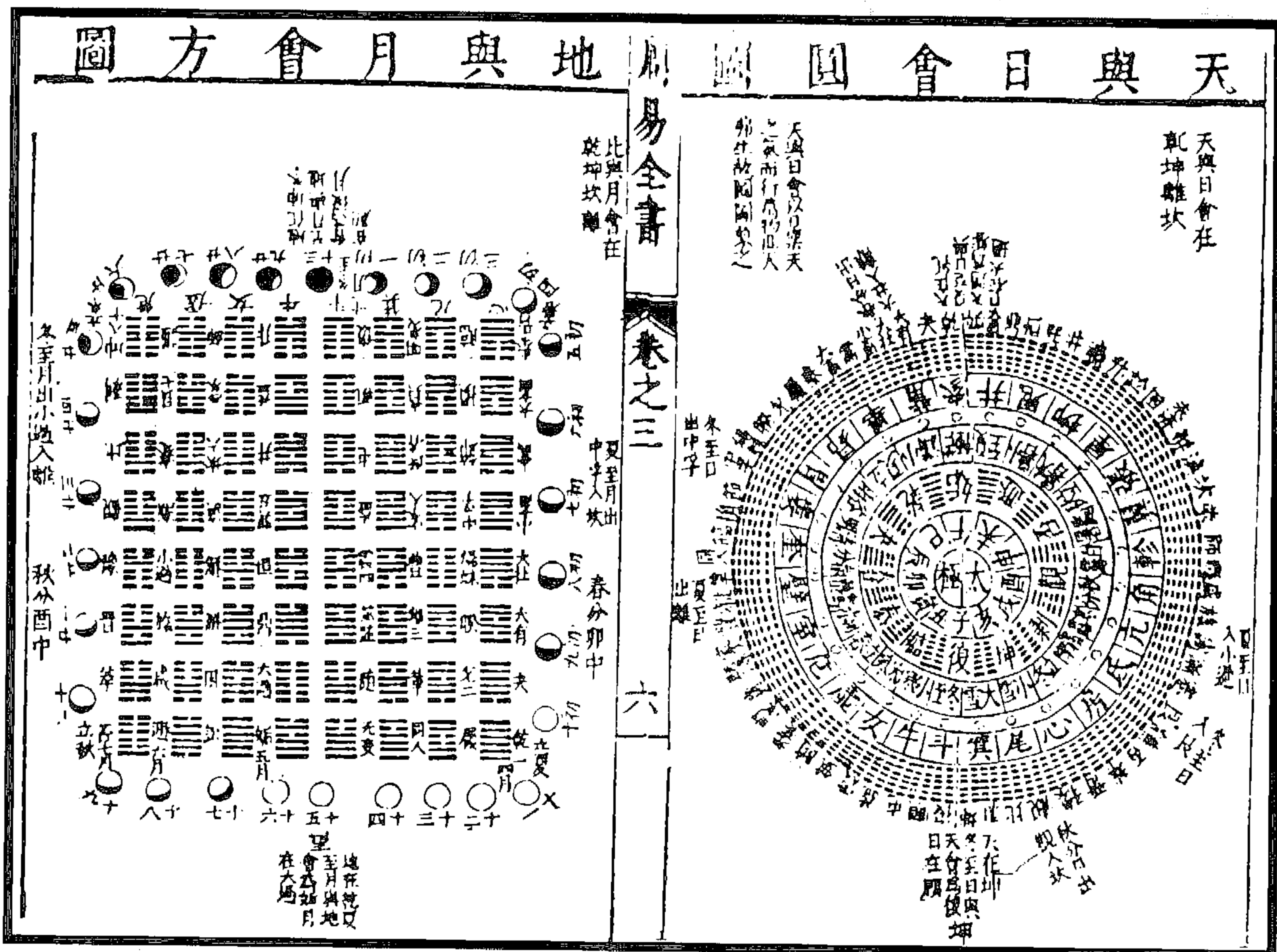
图 282 地与月会方图
