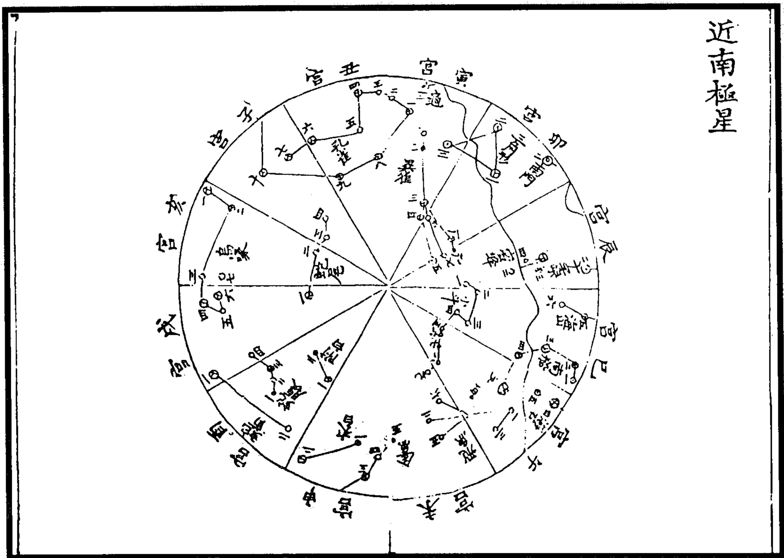
图 113 近南極星图 (戴棠《郑氏爻辰补》)
