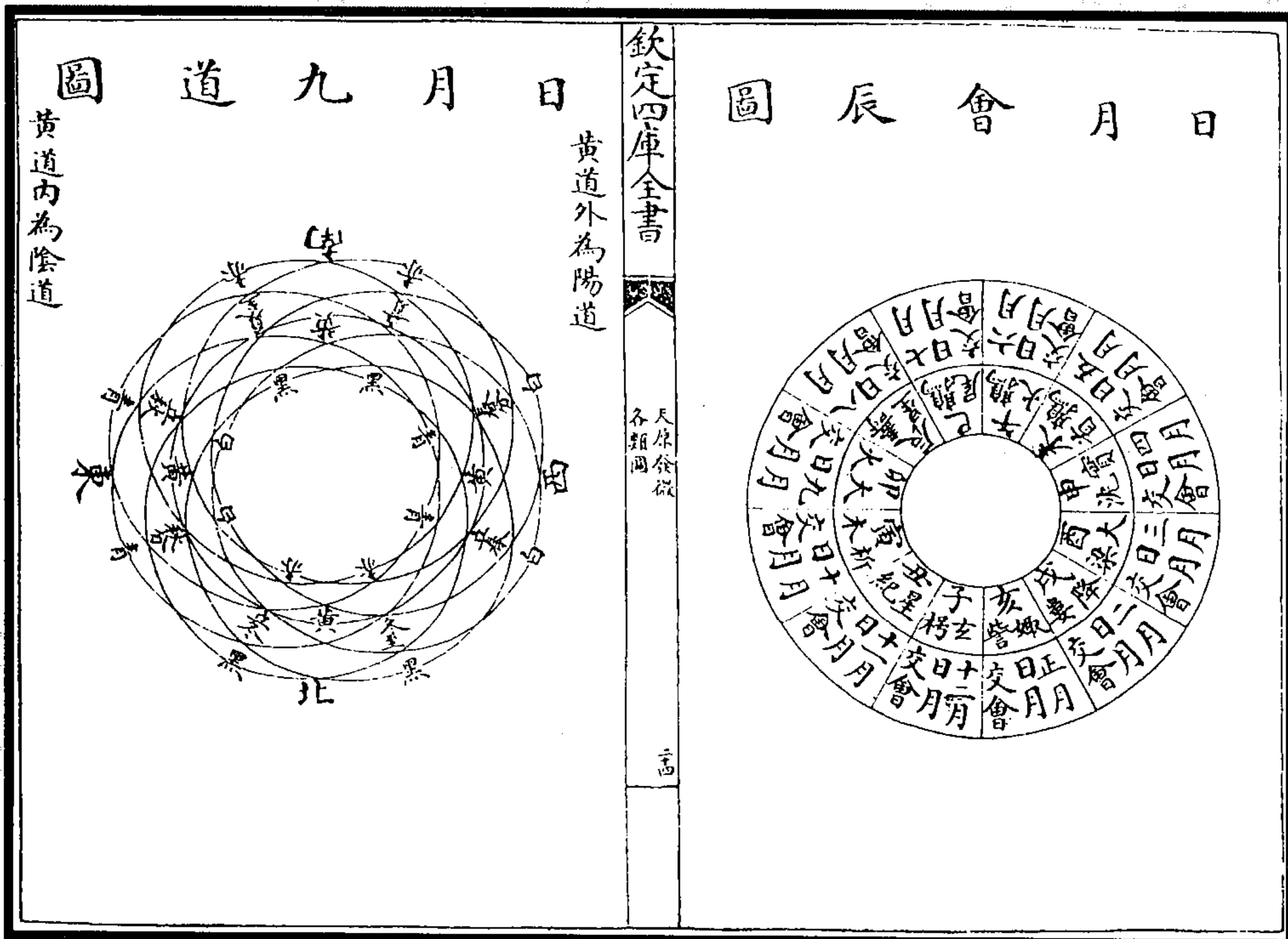
图 51 日月九道图
