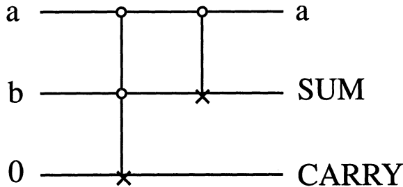
Fig. 6.4 An Adder
