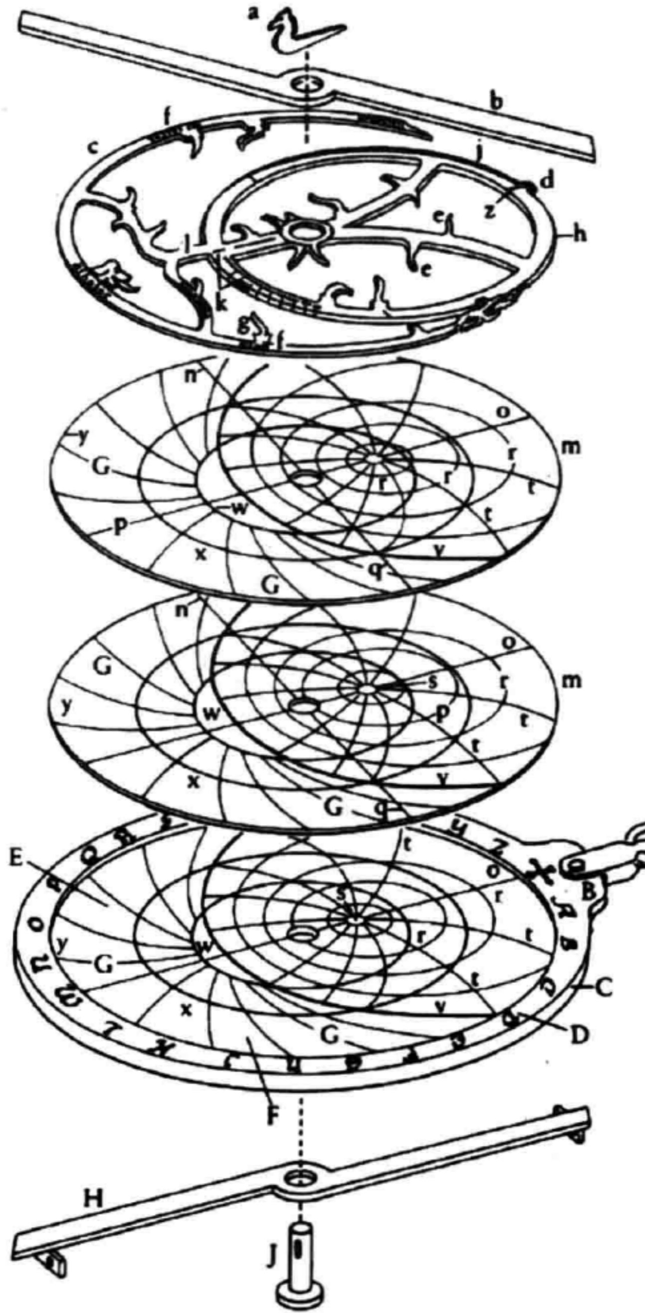
图 11.3 星盘的分解图。最初发表于 J. D. North, Chaucer's Universe , p. 41
