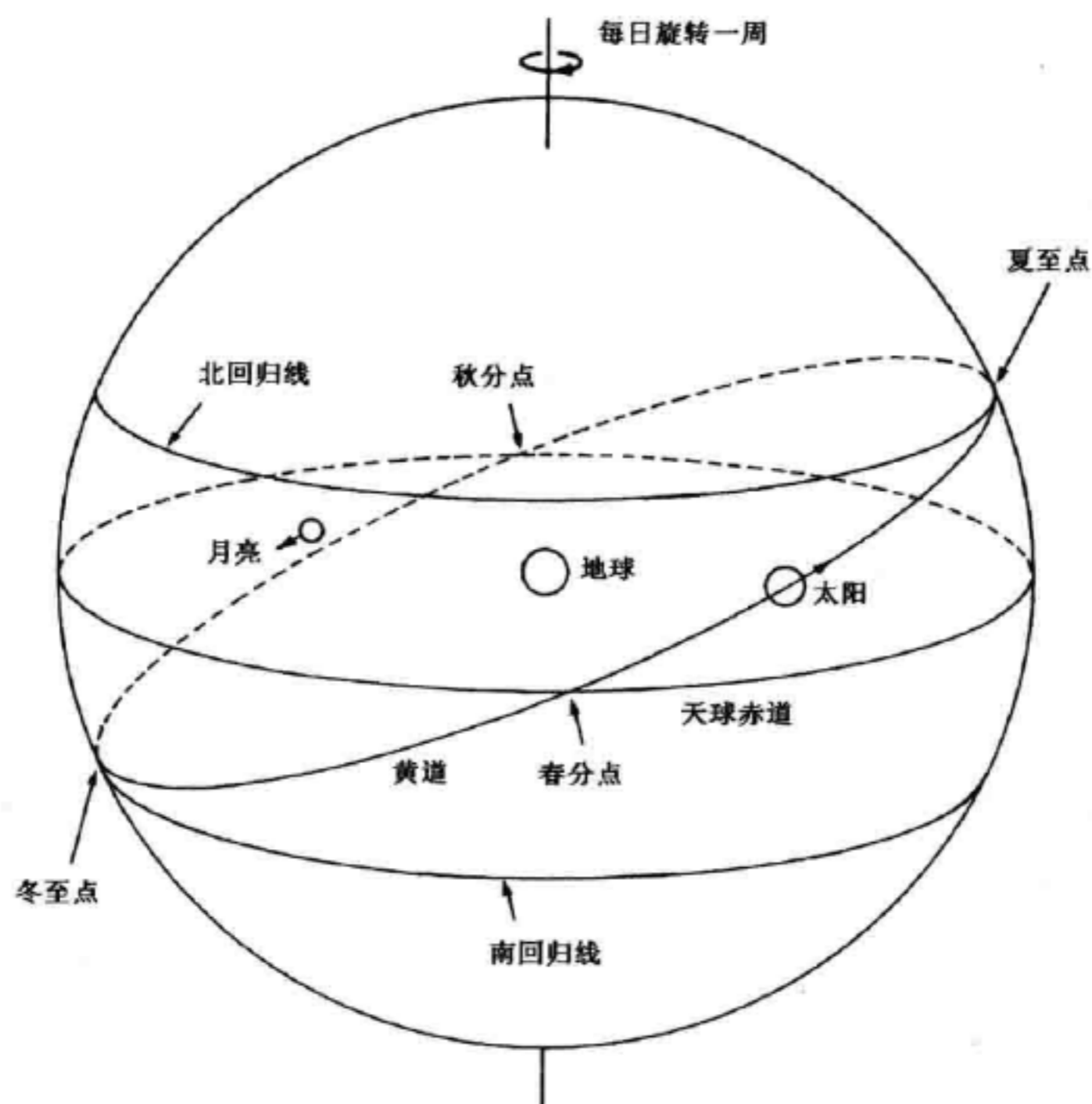
图 5.3 宇宙的两球模型
