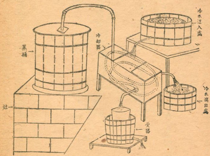
蒸薄荷器的裝置
