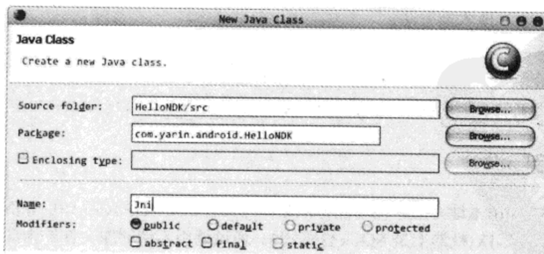
图 16-20 创建 JNI 类
