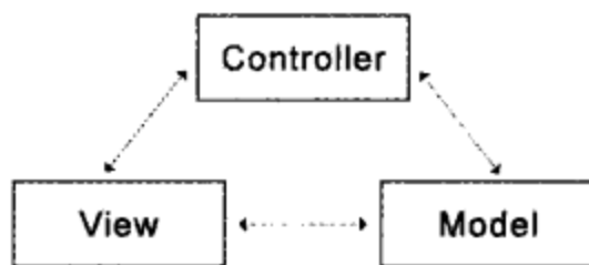
图 14-2 MVC 框架
