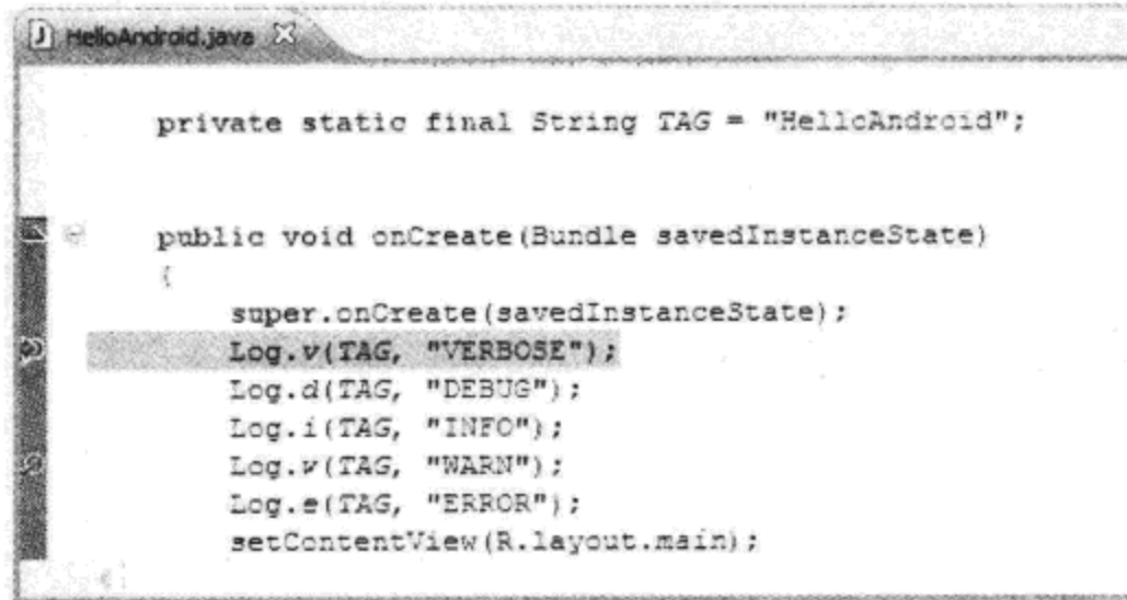
图 2-31 设置“断点”
