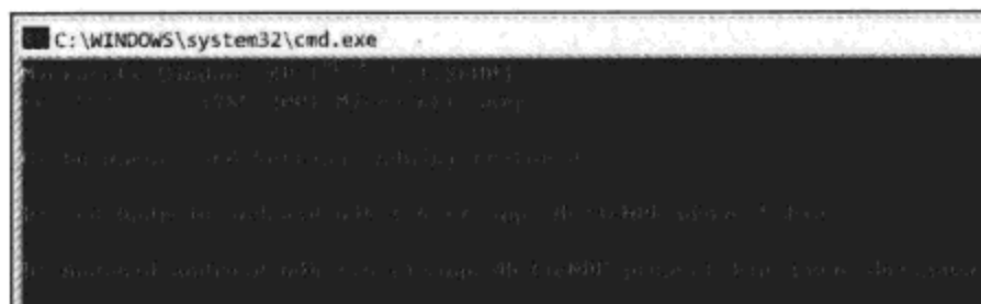
图 16-23 javac 命令
