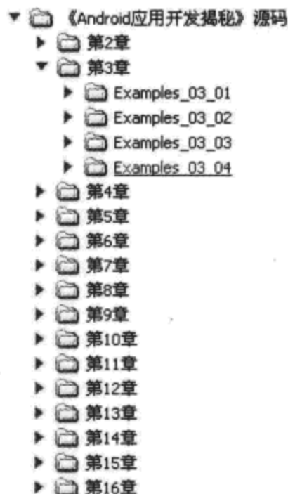
图 1 源码结构图
