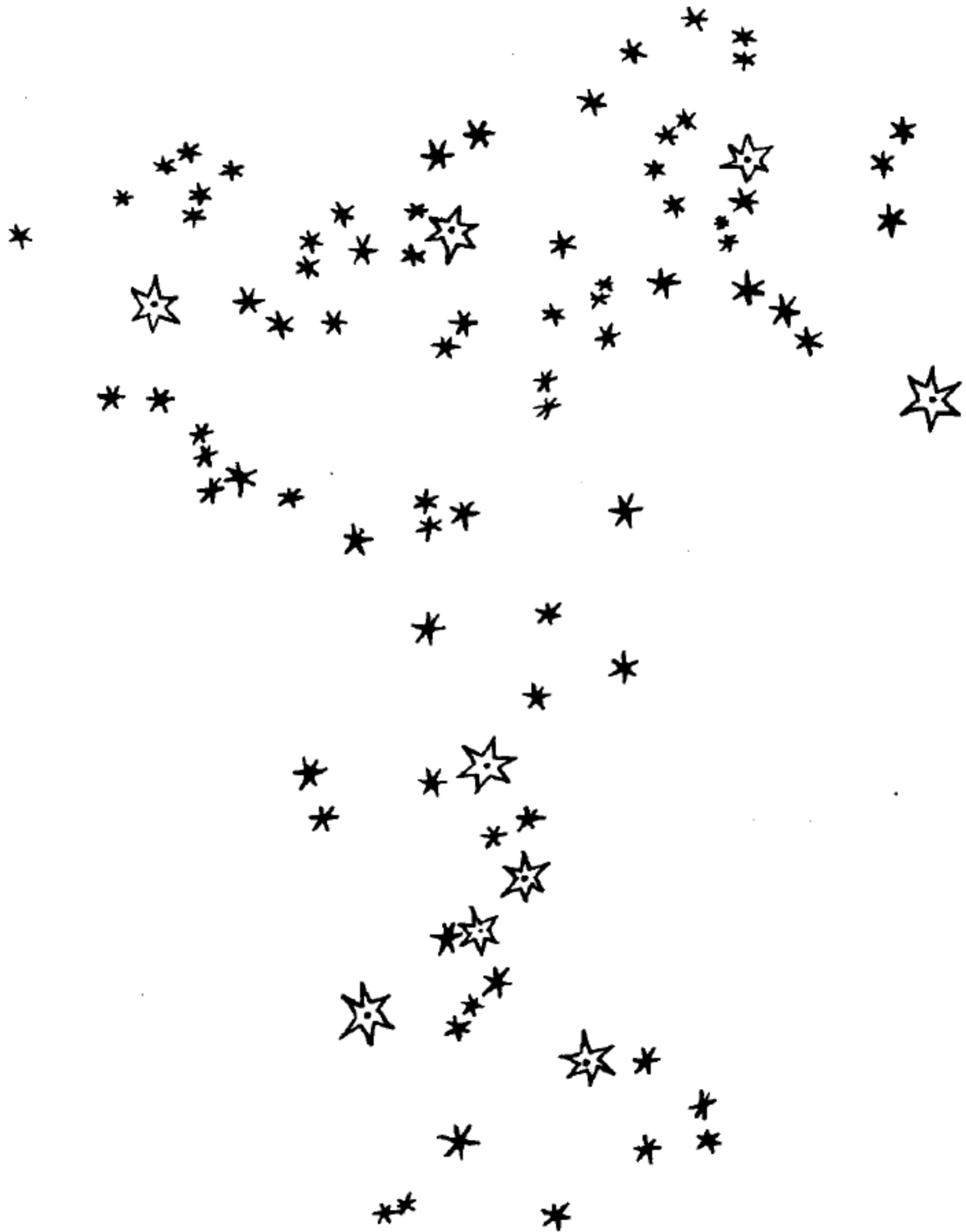
图 17 透过伽利略的望远镜看去，猎户座的腰带和剑所包含的恒星（较小的星）比肉眼所见多 80 颗。
