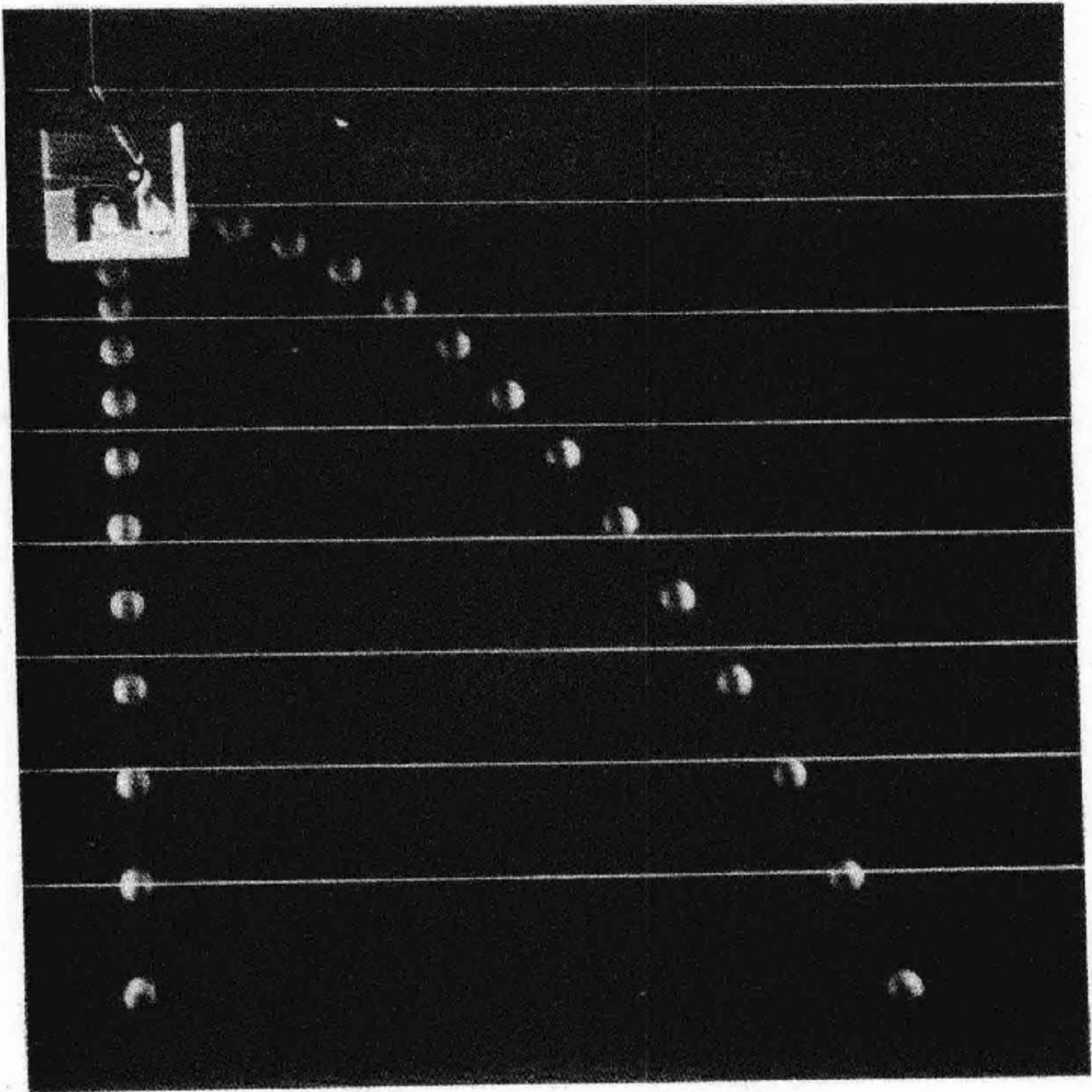
插图 7 这张用频闪观测仪拍摄的照片显示了抛射体运动的竖直分量与水平分量的相互独立性。在 1/30 秒的时间段里，沿抛物线落下的小球与竖直下落的小球所走过的距离完全相同。Berenice Abbott 摄。
