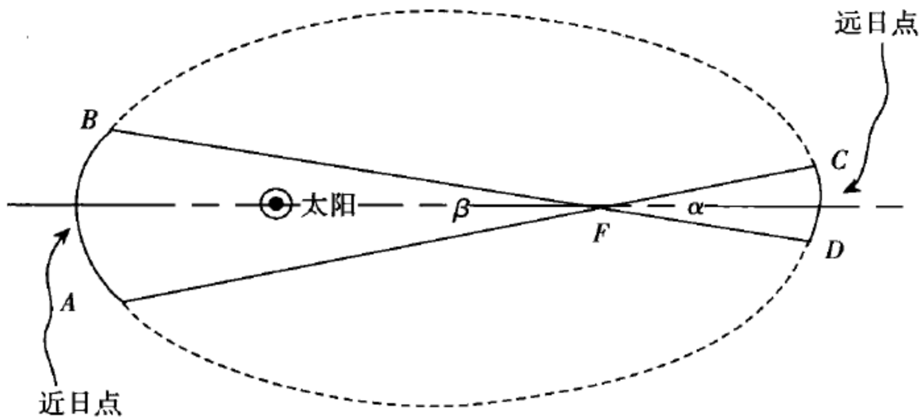
图 28 开普勒的偏心匀速点定律。如果行星在相等时间内相对于空焦点 F 扫过相等的角度，那么它将在相等时间内通过弧 AB 和 CD ，因为角度 \alpha 与 \beta 相等。根据这一定律，行星通过弧 AB （在近日点）时要比通过 CD （在远日点）时运动得更快，一如等面积定律所预言的。然而，这条定律只是一种粗略的近似。但在 17 世纪，某些修正因素被加到这一定律中，使它给出了更为精确的结果。
