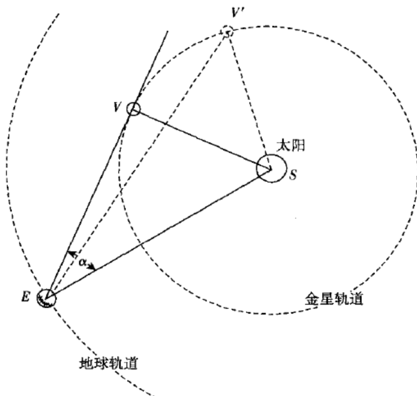
图 12 在哥白尼体系中可以计算出金星与太阳的距离。当角距（即金星与太阳成的角 \alpha ）最大时，从地球到金星的视线（EV）与金星轨道相切，因而垂直于半径 VS。用初等三角学知识很容易计算出 VS 的长度。在其他任何方向，比如 V'，角距都不是最大。
