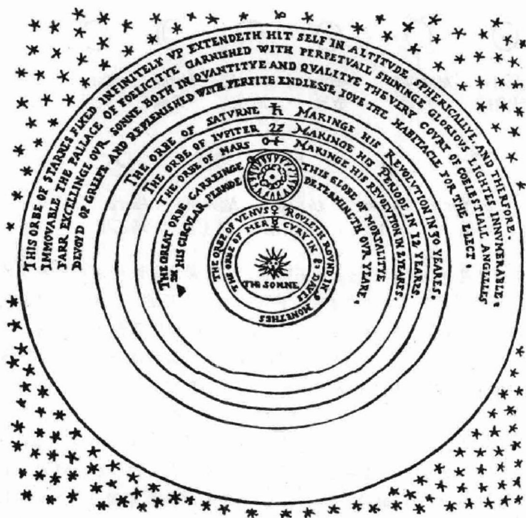
图 8A 这张哥白尼体系图取自托马斯·迪格斯 (Thomas Digges) 的《对天球的完美描绘》(A Perfit Description of the Caelestial Orbes, 1576)。该书对哥白尼的《天球运行论》做了英文节译。迪格斯为该体系增加了一个特征, 那就是使恒星天球变得无限。
