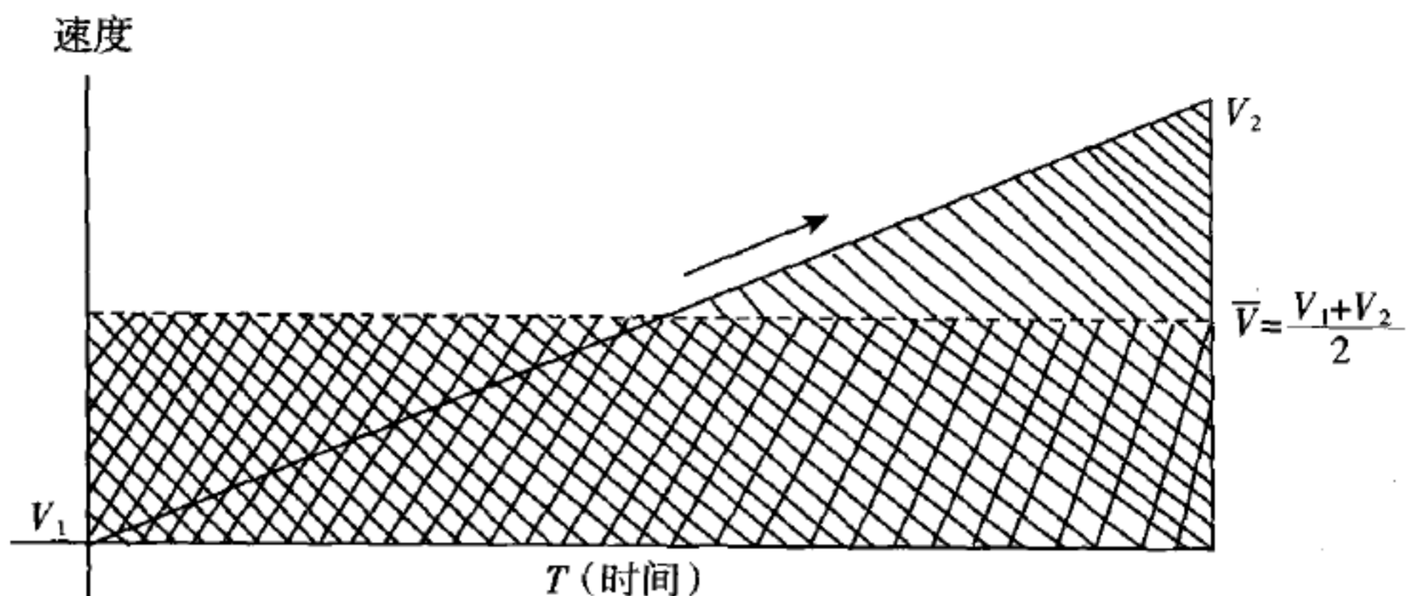
图 19 巴黎的奥雷姆用几何证明了，由初速度 V_1 匀加速运动到末速度 V_2 的物体在时间 T 内走过的距离 D 等于在同样时间内物体以 V_1 和 V_2 的中间速度匀速运动所走过的距离。他认为速度-时间图所包围的面积为距离 D 。匀加速运动将对应一条斜线，而匀速运动则对应一条水平线。前者的面积为三角形面积 1/2T \times V_2 。后者的面积则为矩形面积 T \times 1/2V_2 ，三角形的高是矩形高的两倍。因此，两者的面积相等，即走过的距离相等。
