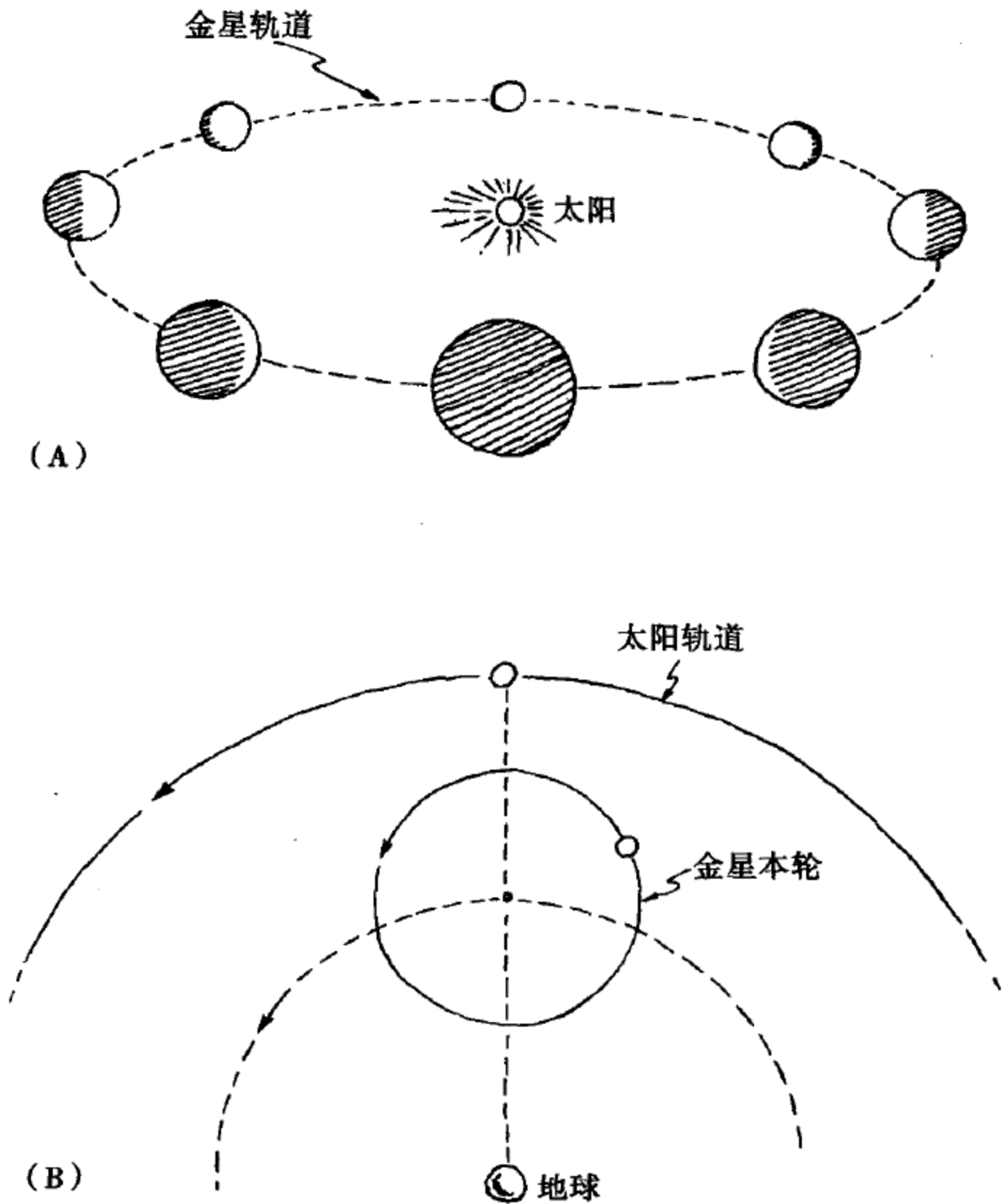
图 18 伽利略首次发现了金星的位相，这是反对古代天文学的有力证据。在 (A) 中，我们可以看到位相的存在符合哥白尼体系，金星相对视直径的变化支持了行星拥有绕日轨道的观念。在 (B) 中，我们可以看出为何这种现象在托勒密体系中不可能出现。
