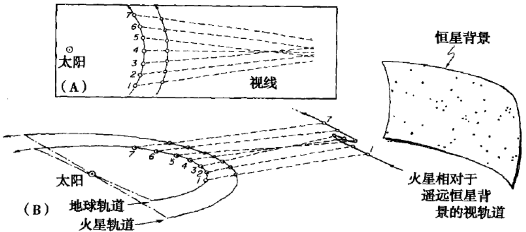
图9 在哥白尼体系中，很容易解释行星的逆行视运动；它实际上是相对速度的问题。这里的视线表明了为什么外行星（即比地球距离太阳更远的行星）看起来会调转方向。它绕太阳运行的速度要慢于地球。
