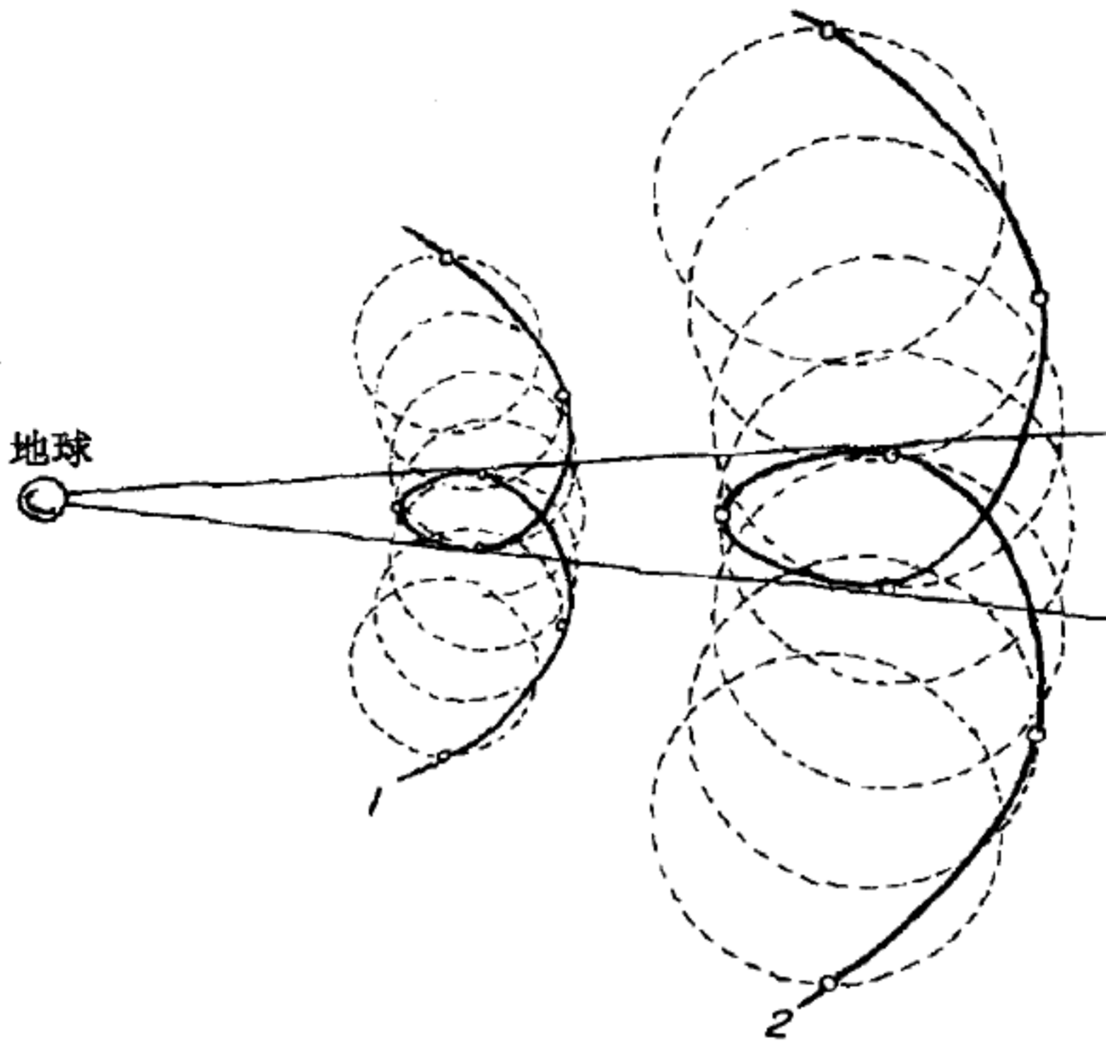
图 13 在托勒密体系中通过测量角度而非距离来预测行星位置。此图显示，如果月球的相对周期相同，那么无论距离如何，观测结果都相同。
