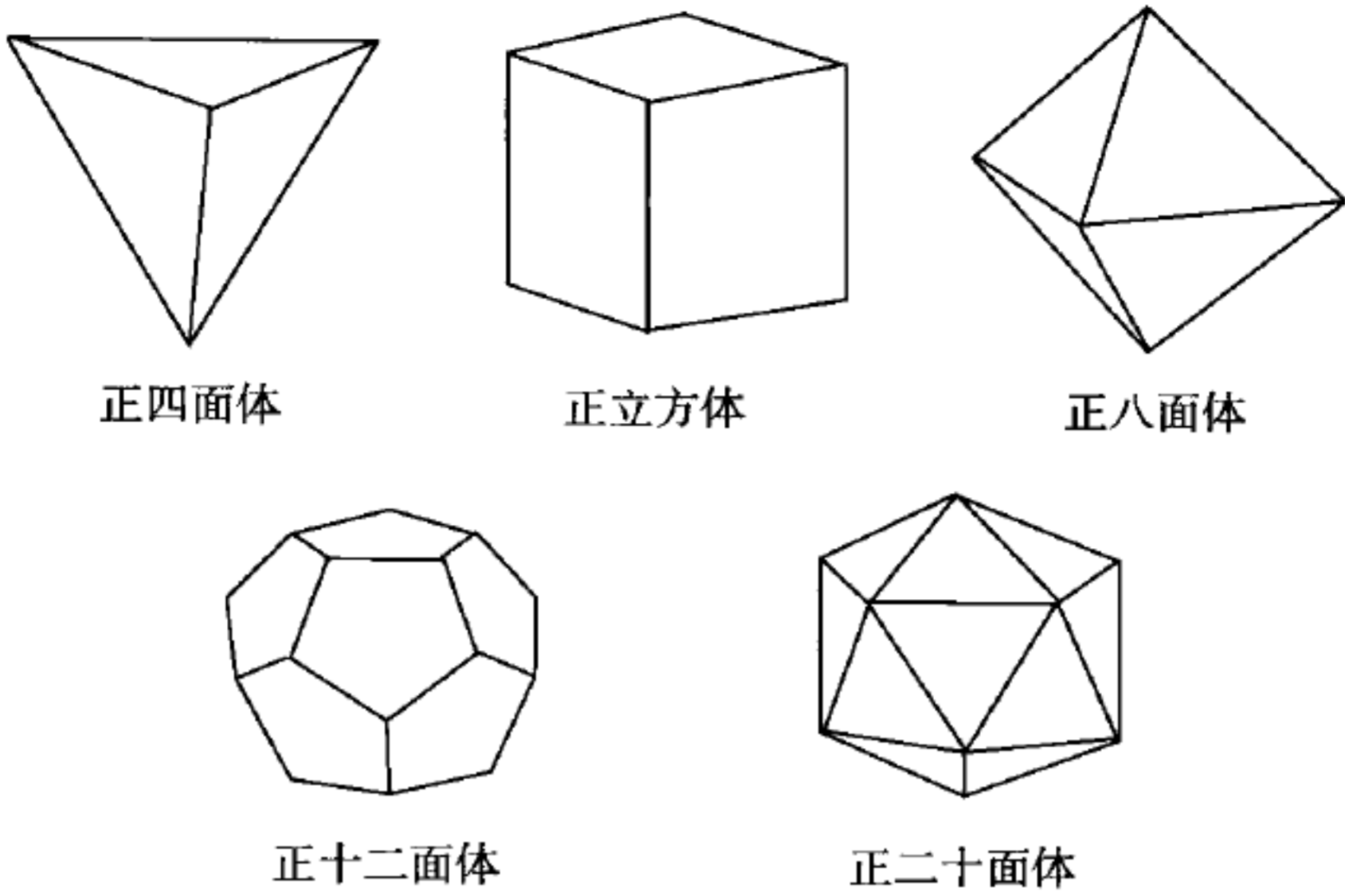
图 25 正多面体。正四面体有四个面，每一个面都是等边三角形。正立方体有六个面，每一个面都是正方形。正八面体有八个面，每一个面都是等边三角形。正十二面体有十二个面，每一个面都是等边五角形。正二十面体有二十个面，每一个面都是等边三角形。
