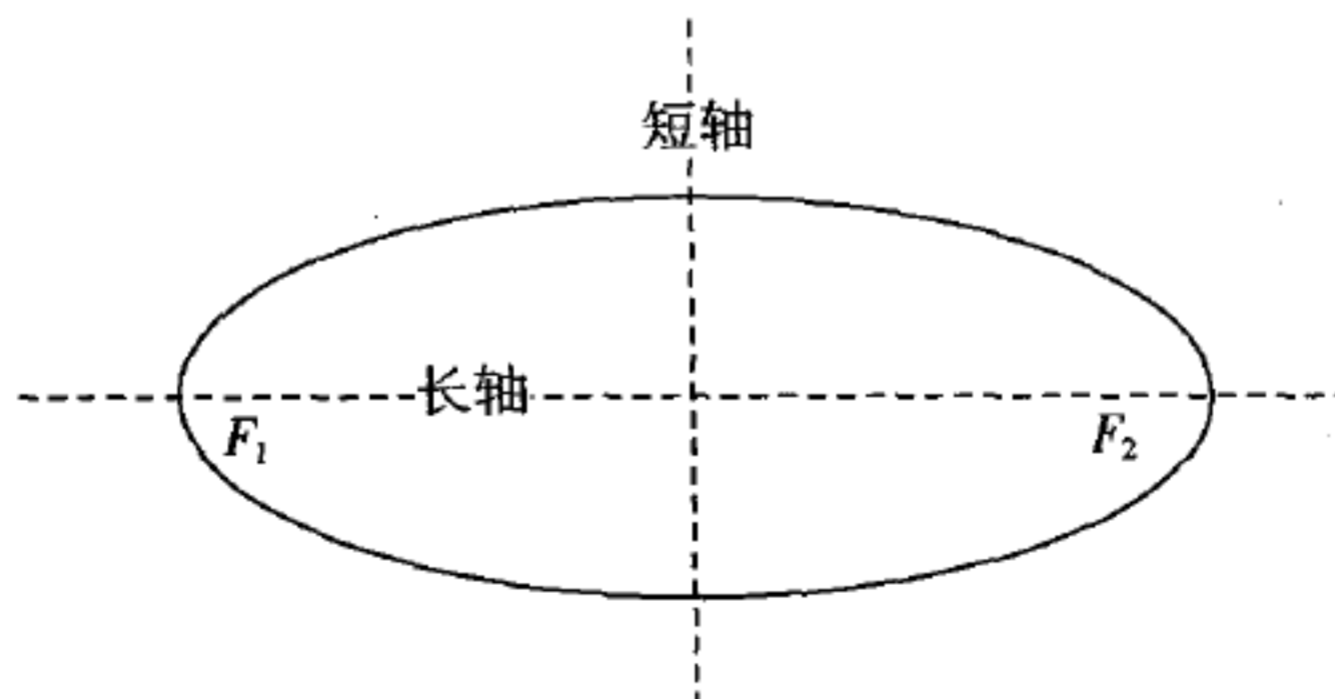
图 22 椭圆的画法如 (A) 所示。如果使用同样的线，但是将钉子之间的距离变为 F_2, F_3, F_4 等等，则可以画出 (B) 中的所有图形。
