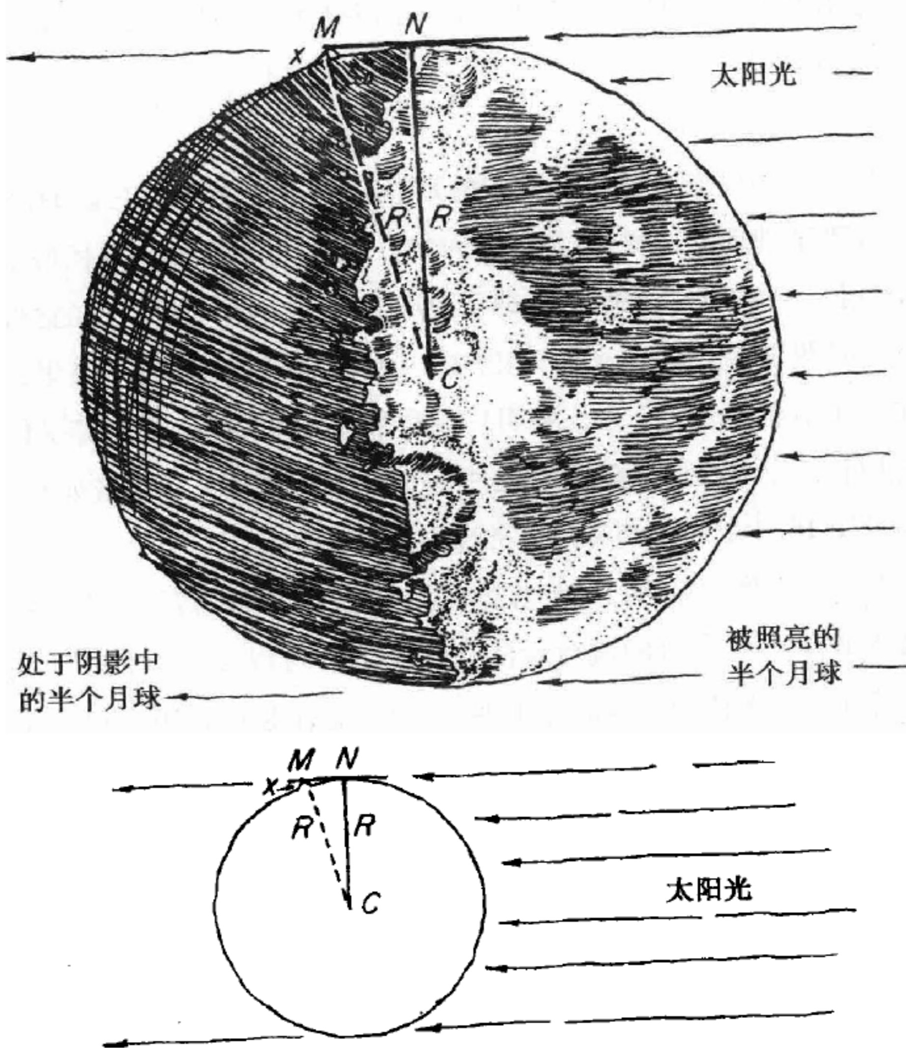
图 16 伽利略对月球山高的测量简单而令人信服。点 N 是月球明暗的界点（分界）。点 M 是暗区观察到的一个亮点；伽利略正确地猜测，这个亮点就是山的顶峰，由于月球的弯曲，山脚仍处于阴影中。由已知的月地距离可以计算出月球半径，并通过望远镜估算出 MN 的距离。根据毕达哥拉斯定理， CM^2 = MN^2 + CN^2 。既然 R 是半径， x 是山的高度，则有
