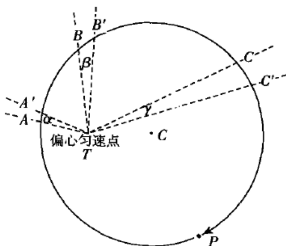
图 7 偏心匀速点是托勒密体系中用来解释表观的行星速度变化的一种技巧。虽然 P 从 A 到 A' 、从 B 到 B' 、从 C 到 C' 的运动相对于圆心 C 并非均匀, 但相对于偏心匀速点 T 却是均匀的, 因为 \alpha 、 \beta 、 \gamma 这三个角相等。行星在相同时间内走过弧 AA' 、 BB' 和 CC' , 但速度看上去却是不同的。
