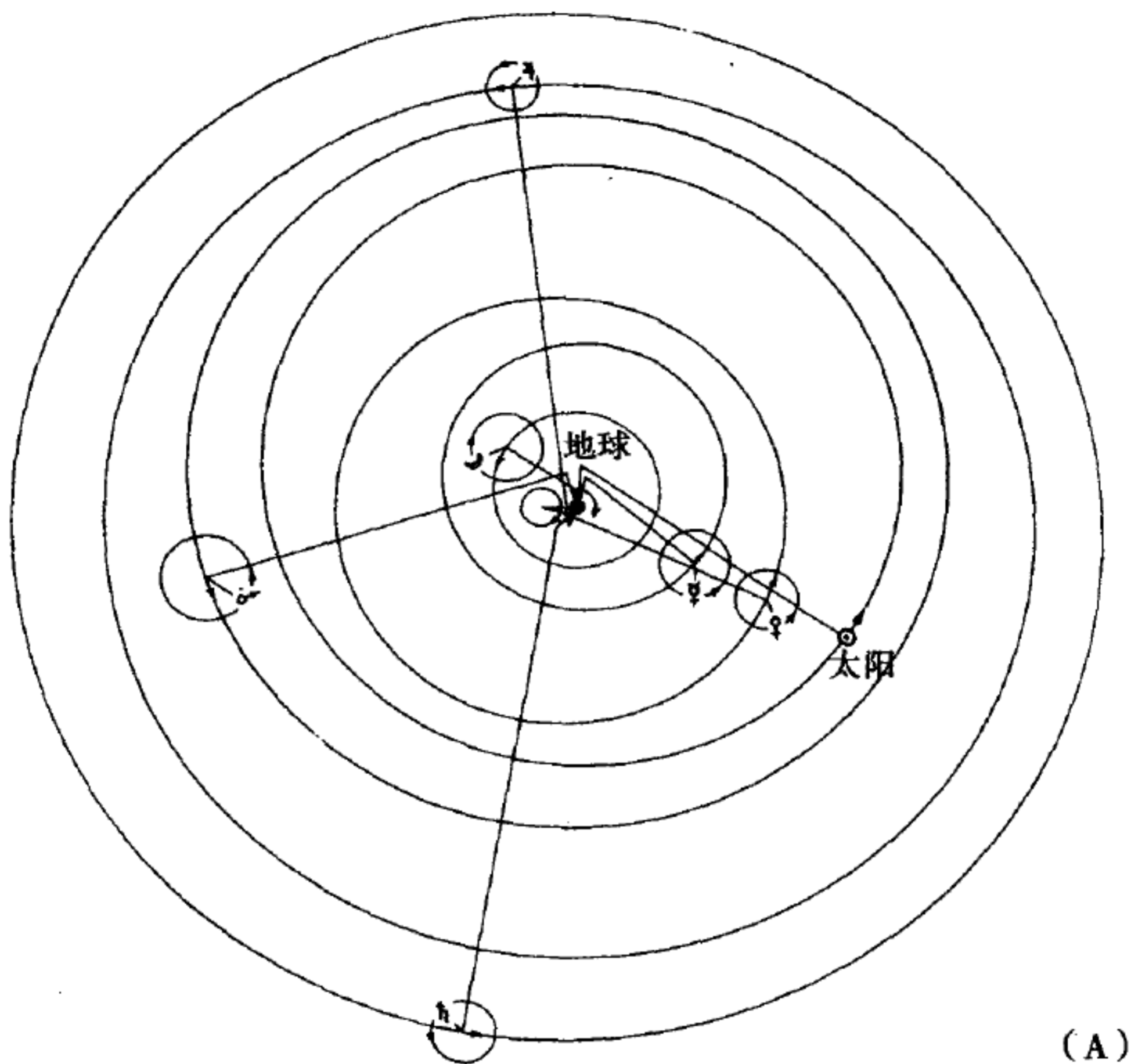
图 14 由这种比较可以看出，托勒密体系 (A) 和哥白尼体系 (B) 差不多同样复杂。行星均轮 (大圆) 半径内端的点表示托勒密体系中相对于太阳轨道中心的轨道中心，以及哥白尼体系中相对于太阳的轨道中心。注意两个体系中本轮的使用。在这张图中，为了看起来更清楚，金星 (♀) 本轮和水星 (☿) 本轮的中心被移了位。在托勒密体系中，这两个本轮的中心仍然固定在日地连线上。(根据 William D. Stahlman)
