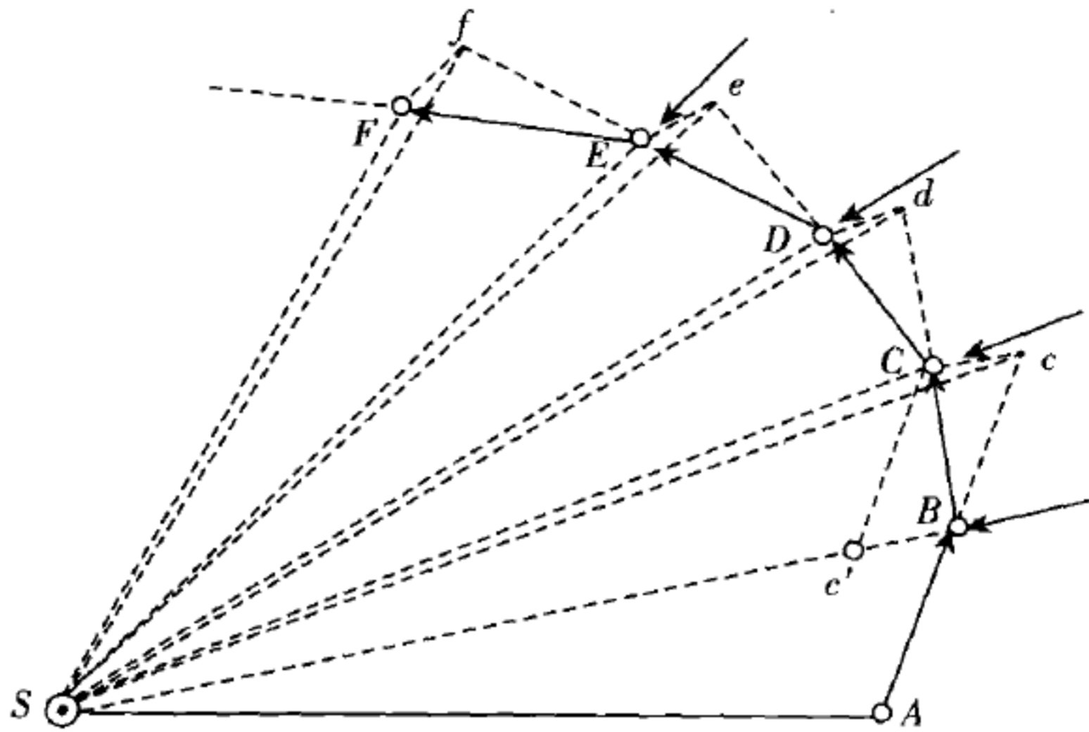
图 31 如果物体在 B 没有受到推力，则在时间 T 内，它将沿着 AB 的延长线移动到 c 。然而， B 点的推力使物体获得了朝向 S 的运动分量。如果在时间 T 内物体的运动只来自这一推力，则物体将从 B 运动到 c' 。这两种运动的组合将使物体在时间 T 内从 B 运动至 C 。牛顿证明了三角形 SBC 的面积等于三角形 Sbc 的面积。因此，即使有朝向 S 的推力，等面积定律也依然成立。
