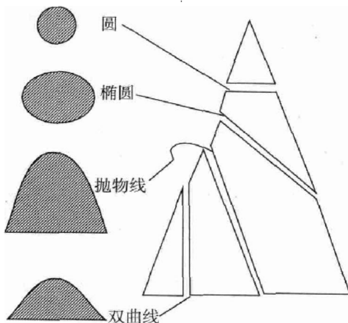
图 24 使用如图所示的切割方法便可获得圆锥曲线。注意，圆是平行于锥底切出的截面，抛物线则是平行于母线切出的截面。
