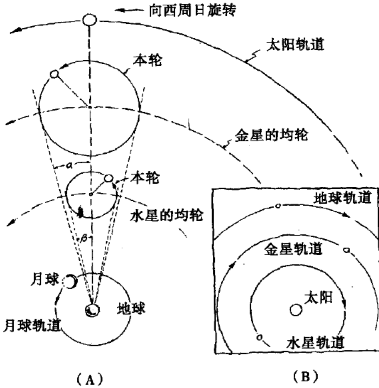
图 10 内行星（即轨道落在地球与太阳之间的行星）的逆行也可以用视线来解释。金星绕太阳运行的速度要快于地球。
