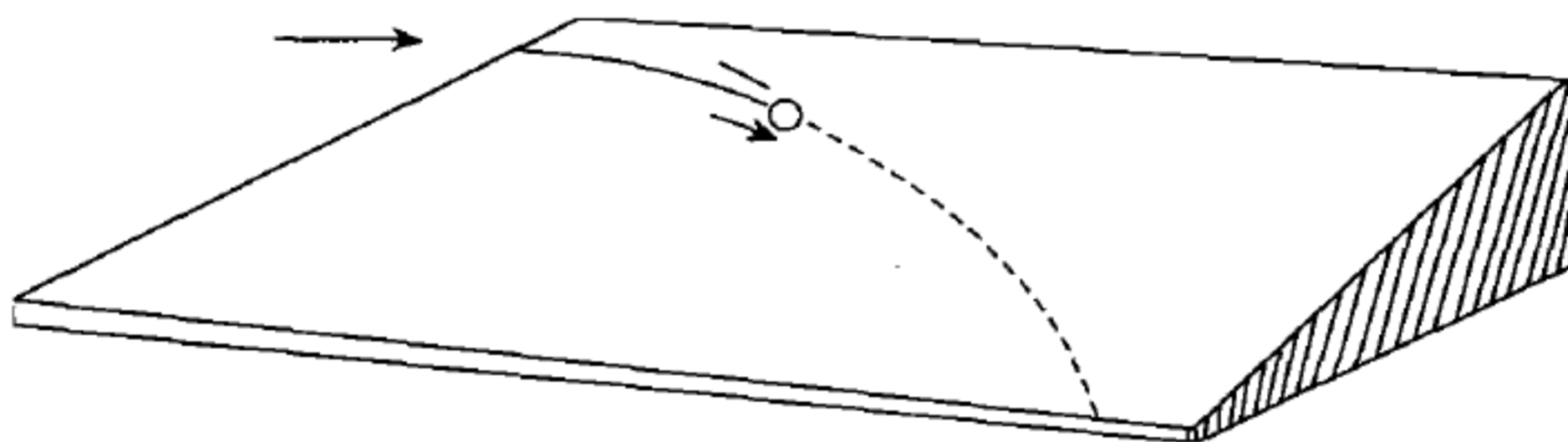
图 21 伽利略用于证明抛射体运动的装置是一个楔形物。小球从楔形物的顶端以水平方向开始运动，以抛物线落向斜面底端。
