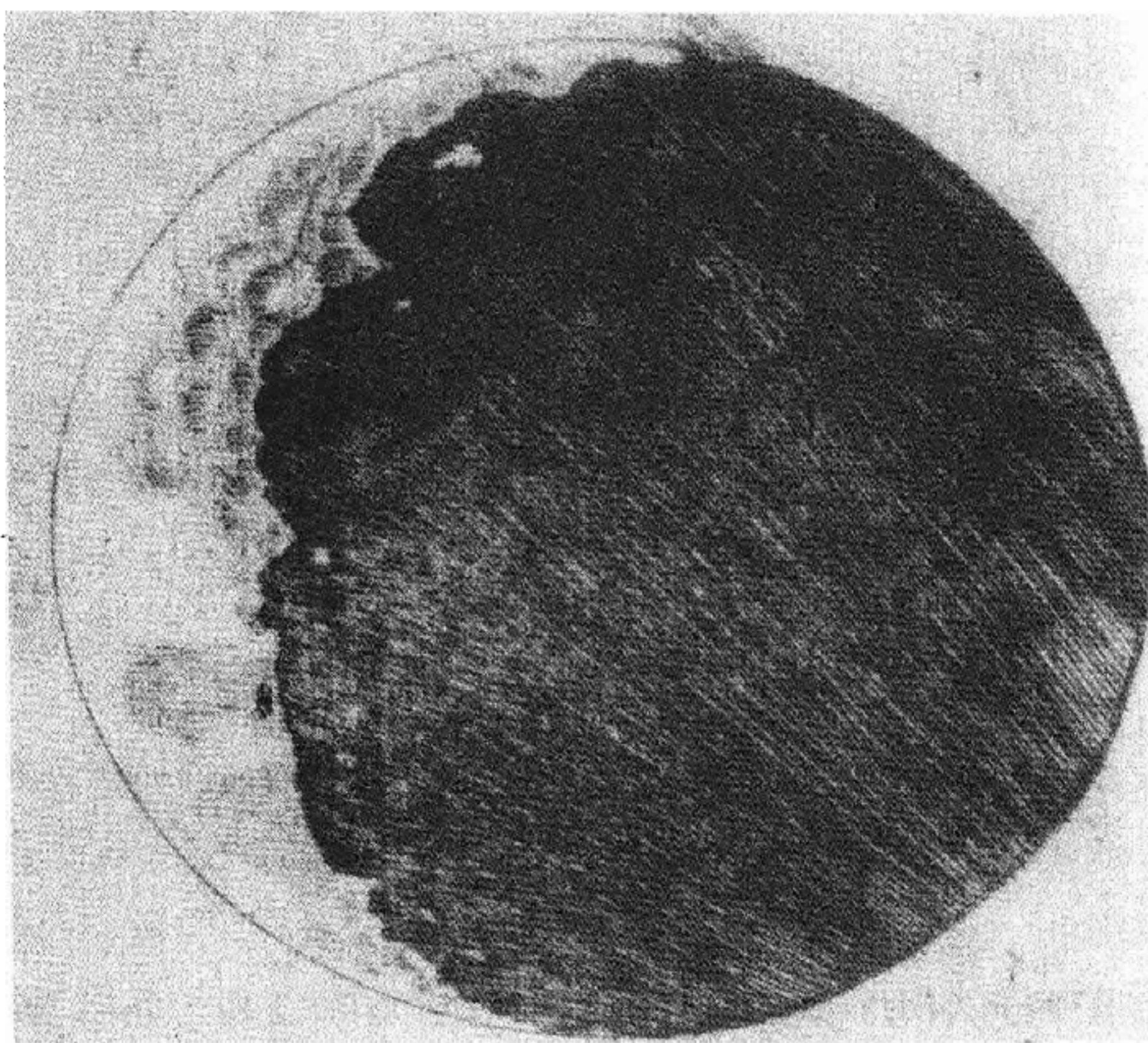
插图4 伽利略本人所绘的月球，这里按照展示天文图片的习惯作了颠倒。望远镜镜头中呈现的是颠倒的景象。
