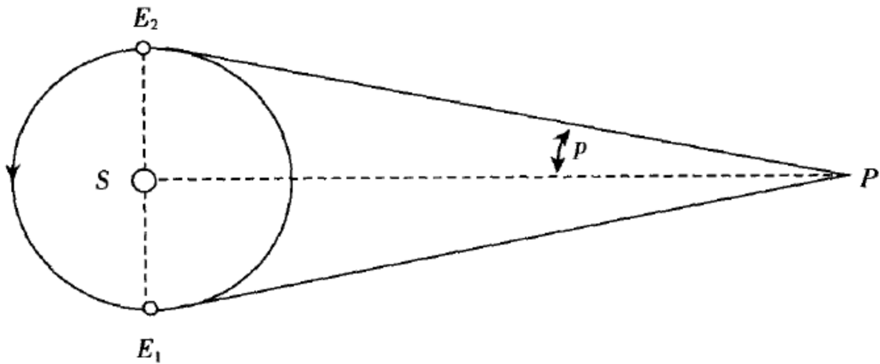
图 15 恒星的周年视差是角 p ，通过它可以计算出恒星与太阳和地球的距离。地球在半年间的位置分别为 E_1 和 E_2 。 E_1E_2 给出了一条 200000000 英里的基线，由它可以观测恒星 P ，得到角 E_1PE_2 或 2p 。
