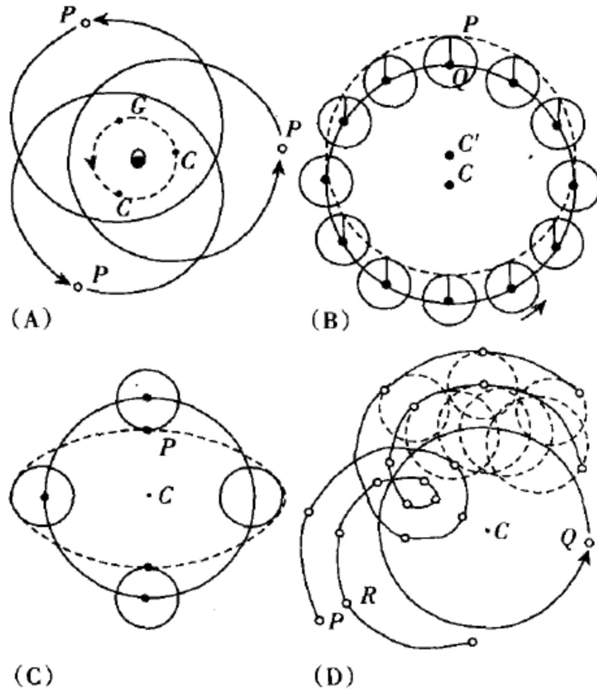
图 6 凭借着本轮和均轮（以及聪敏），天文学家借助托勒密体系几乎能够描述观察到的一切行星运动。在（A）中， P 点沿着一个圆心为 C 的圆周旋转，而 C 又沿着一个圆心为 X 的小圆旋转。在（B）中，本轮均轮组合的结果是将 P 的轨道的视中心由 C 移至 C' 。在（C）中，本轮均轮组合产生了一条椭圆曲线。（D）描绘的是沿着本轮上的一个本轮移动的 P 点的轨迹。 P 所在的圆的圆心是 R ， R 所在的圆的圆心是 Q ， Q 所在的圆的圆心是 C 。
