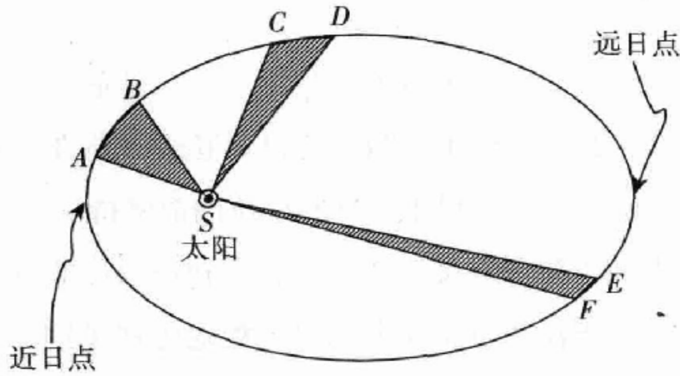
图 27 开普勒的等面积定律。由于行星在相等时间内通过 AB 、 CD 和 EF 三个弧（因为 SAB 、 SCD 和 SEF 的面积相等），所以行星在近日点（距太阳最近）时速度最大，在远日点（距太阳最远）时速度最小。此椭圆的形状为一颗彗星的轨道。行星的椭圆轨道更接近圆形。
