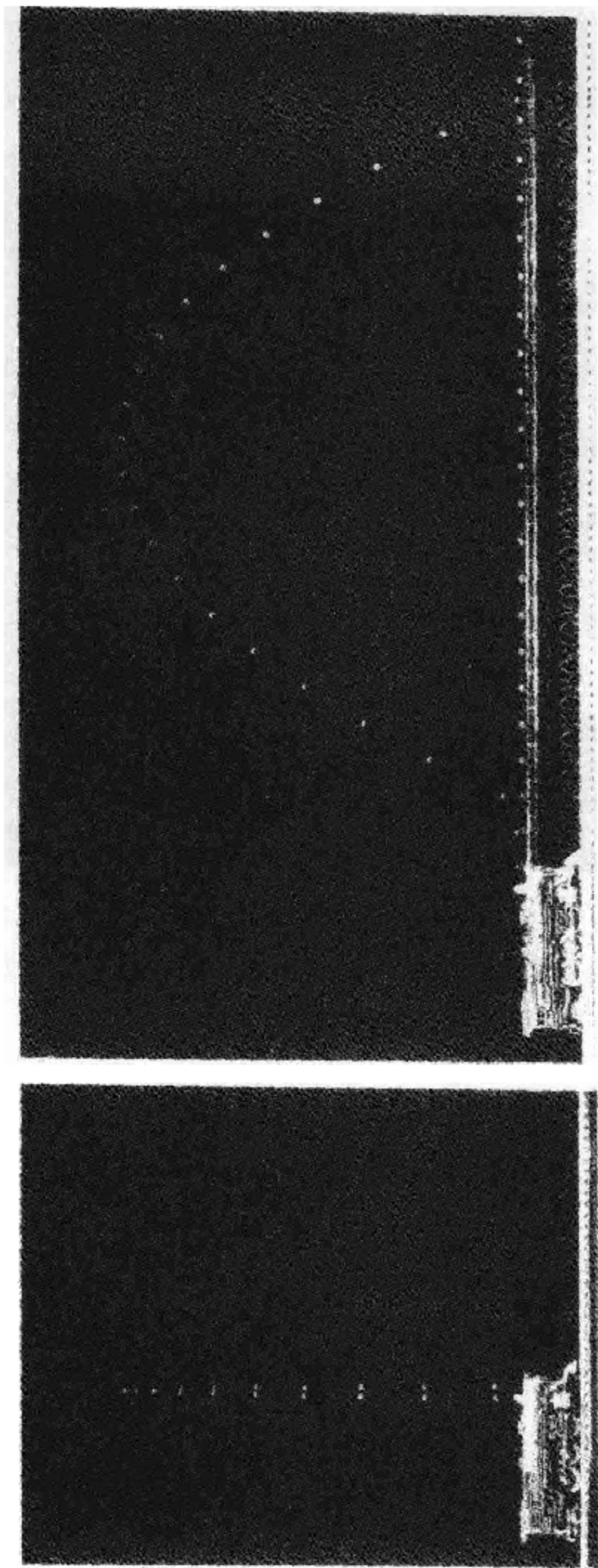
插图6 一列玩具火车在向前运动,一个小球由烟窗中的弹簧枪射出,在空中画出一道抛物线后落在火车上,而不是火车静止不动,小球直上直下地运动。这些用频闪观测仪拍摄的照片显示了伽利略关于落体行为的一个论点,解决了关于从运动船桅上释放的物体的运动的古代争论。如果火车速度是绝对均匀的,而且小球没有遇到空气阻力,它就将落在烟窗里。(事实上,甚至在不完美的实验条件下,小球大多也会击中烟窗。)我们注意到,无论火车是运动还是静止,小球都会到达同一高度。此外,在火车静止情况下拍摄的照片中,小球在曝光时间段内走过的距离几乎完全一致。小球上升时,重力减慢了它的速度;而下落时,重力又使之加速。Berenice Abbott 摄。
