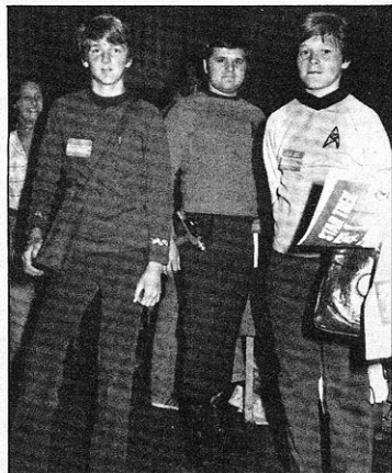
MLM
