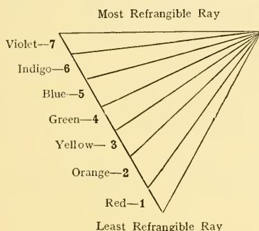
Fig. 33 : PRISMATIC SPECTRUM
